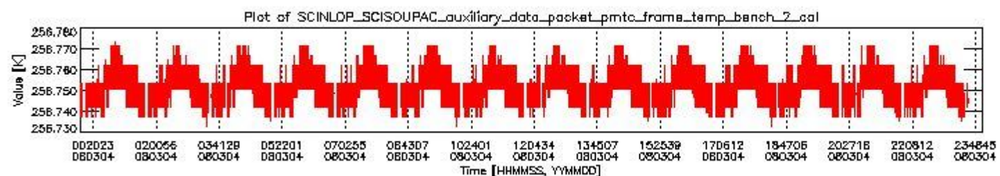
sciamachy_daily_report_level0_KSPT_L0_4303_N_20080304_1.PNG
