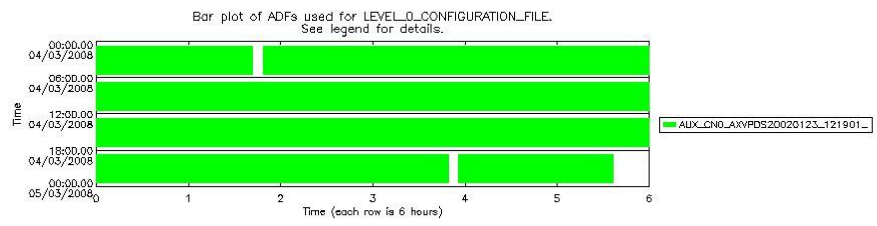
sciamachy_daily_report_level0_KSPT_L0_4303_N_20080304_7.PNG
