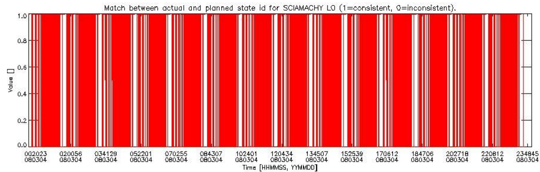
sciamachy_daily_report_level0_KSPT_L0_4303_N_20080304_5.PNG
