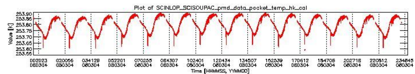
sciamachy_daily_report_level0_KSPT_L0_4303_N_20080304_3.PNG
