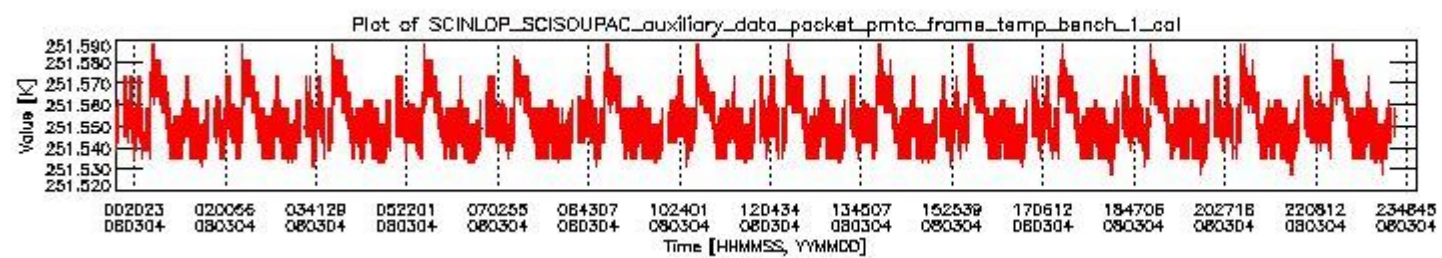
sciamachy_daily_report_level0_KSPT_L0_4303_N_20080304_0.PNG
