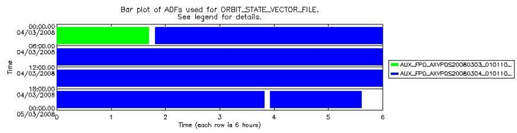
sciamachy_daily_report_level0_KSPT_L0_4303_N_20080304_8.PNG
