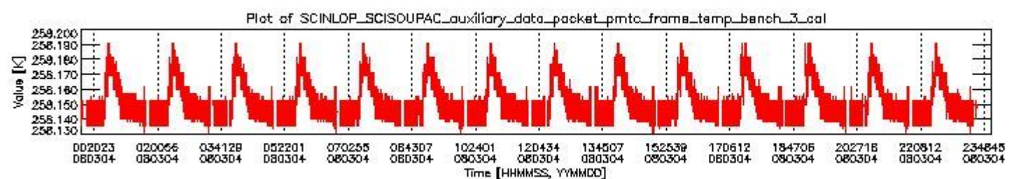
sciamachy_daily_report_level0_KSPT_L0_4303_N_20080304_2.PNG
