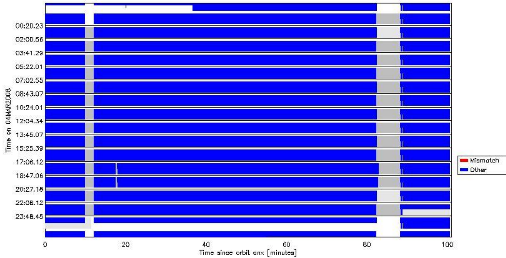
sciamachy_daily_report_level0_KSPT_L0_4303_N_20080304_6.PNG
