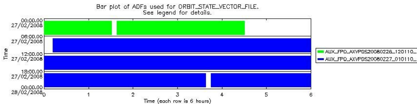
sciamachy_daily_report_level0_KSPT_L0_4303_N_20080227_5.PNG
