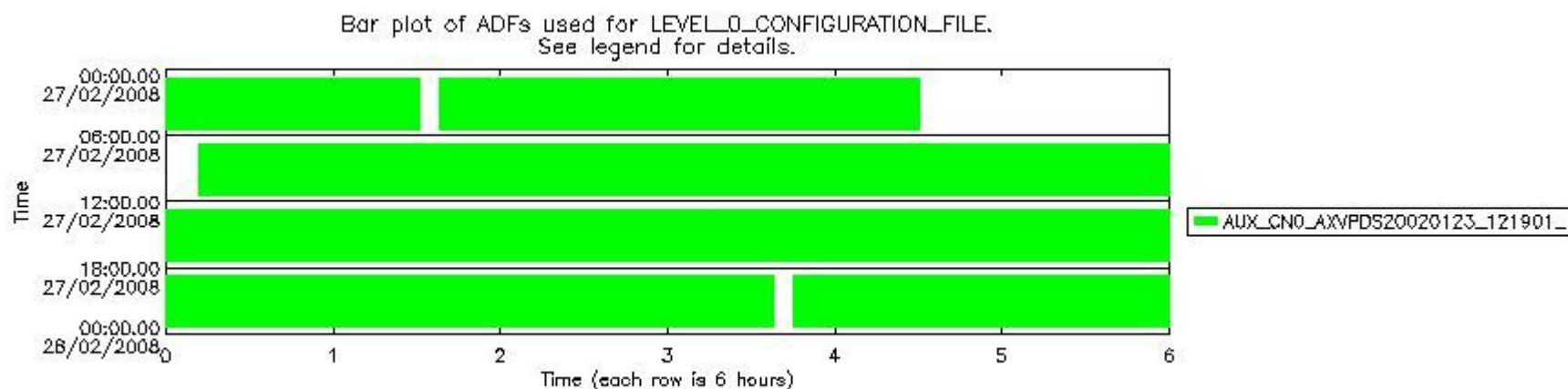
sciamachy_daily_report_level0_KSPT_L0_4303_N_20080227_5.PNG
