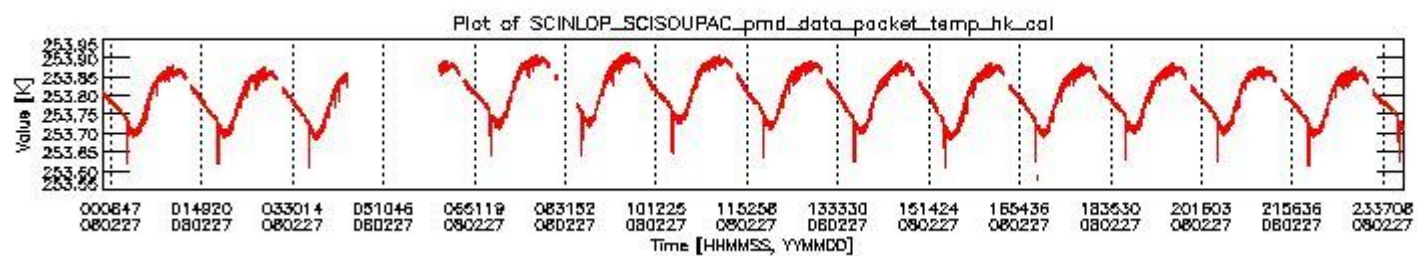
sciamachy_daily_report_level0_KSPT_L0_4303_N_20080227_3.PNG
