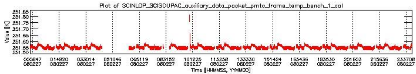
sciamachy_daily_report_level0_KSPT_L0_4303_N_20080227_0.PNG
