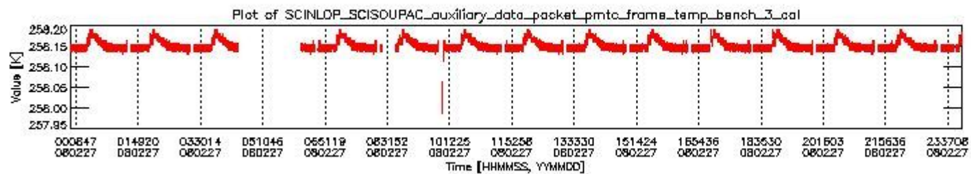
sciamachy_daily_report_level0_KSPT_L0_4303_N_20080227_2.PNG
