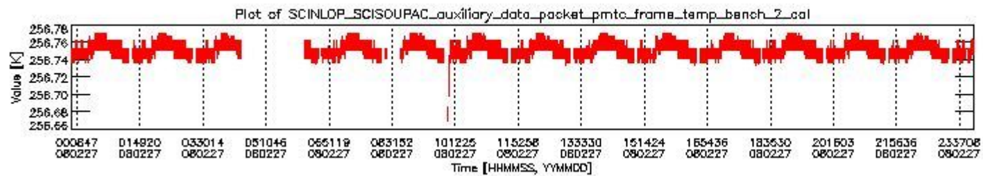
sciamachy_daily_report_level0_KSPT_L0_4303_N_20080227_1.PNG
