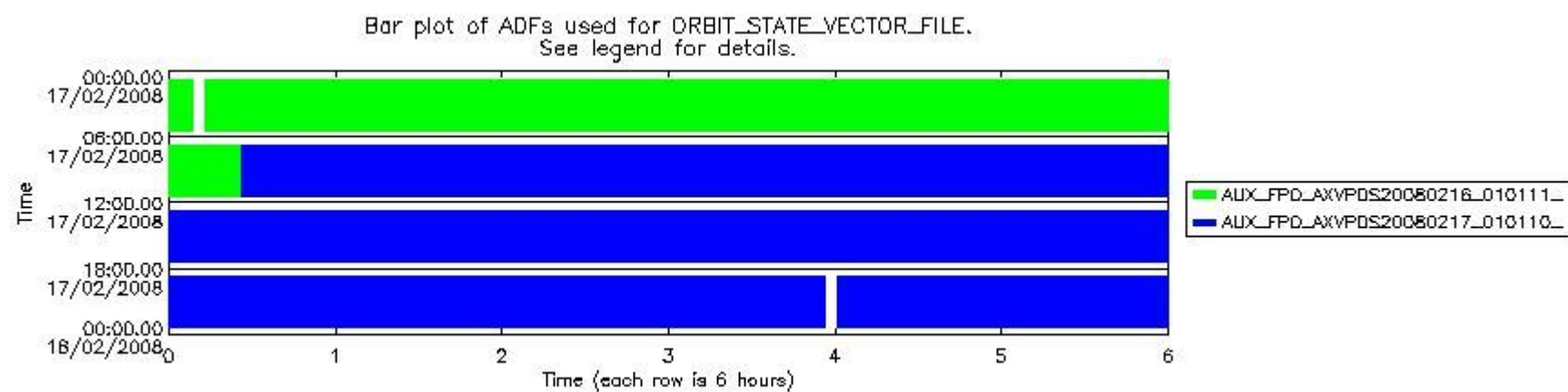
sciamachy_daily_report_level0_KSPT_L0_4303_N_20080217_8.PNG
