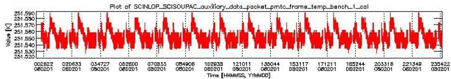
sciamachy_daily_report_level0_KSPT_L0_4303_N_20080201_0.PNG
