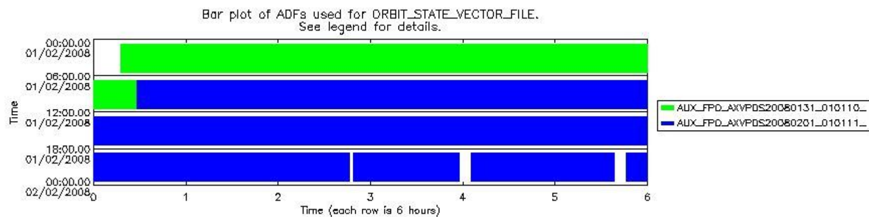
sciamachy_daily_report_level0_KSPT_L0_4303_N_20080201_8.PNG
