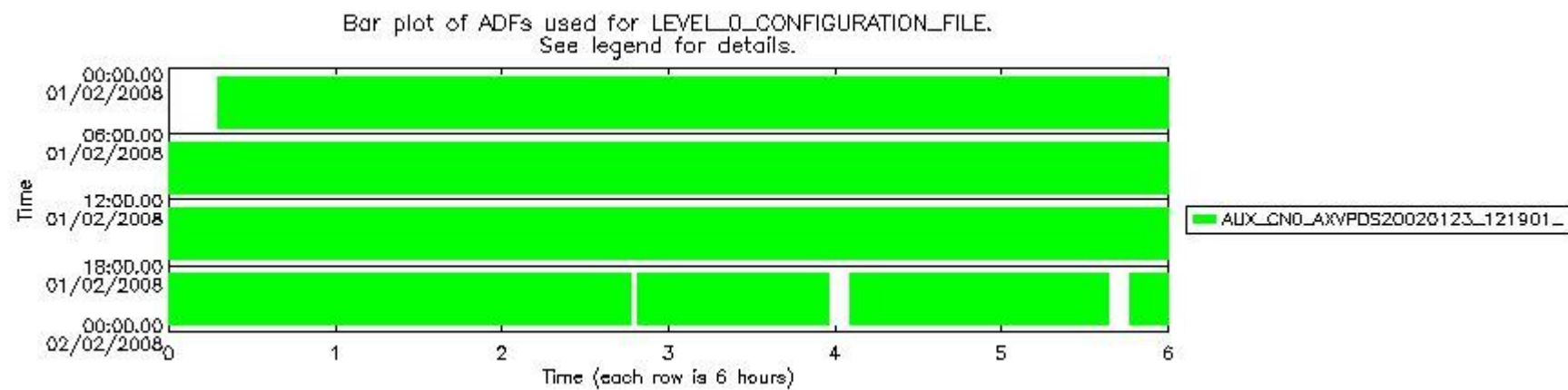
sciamachy_daily_report_level0_KSPT_L0_4303_N_20080201_7.PNG
