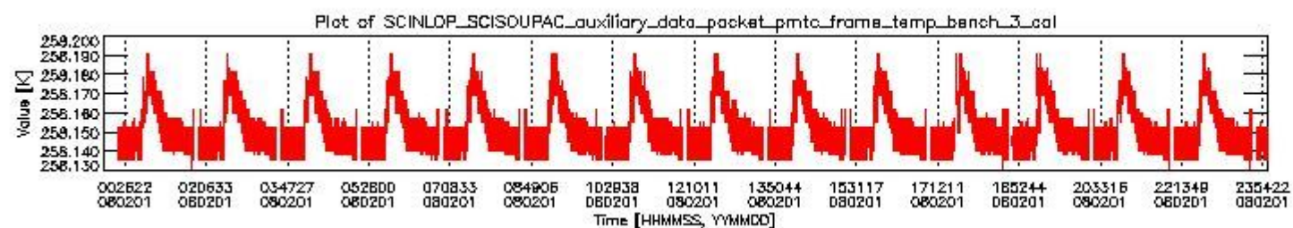
sciamachy_daily_report_level0_KSPT_L0_4303_N_20080201_2.PNG
