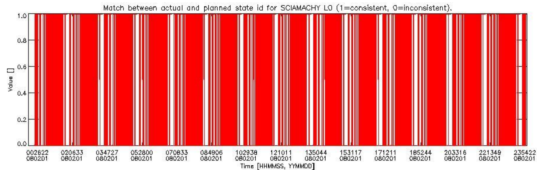
sciamachy_daily_report_level0_KSPT_L0_4303_N_20080201_5.PNG
