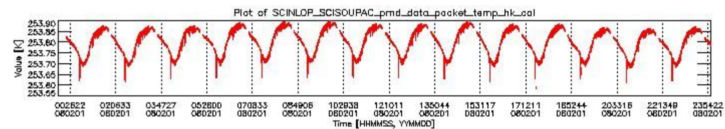
sciamachy_daily_report_level0_KSPT_L0_4303_N_20080201_3.PNG
