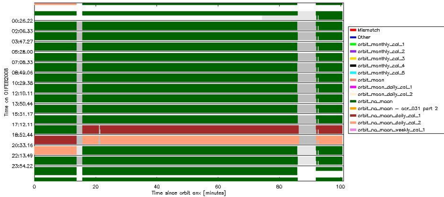
sciamachy_daily_report_level0_KSPT_L0_4303_N_20080201_6.PNG
