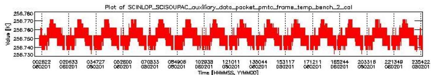
sciamachy_daily_report_level0_KSPT_L0_4303_N_20080201_1.PNG
