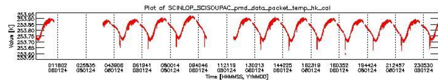
sciamachy_daily_report_level0_KSPT_L0_4303_N_20080124_3.PNG
