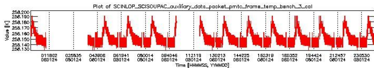
sciamachy_daily_report_level0_KSPT_L0_4303_N_20080124_2.PNG
