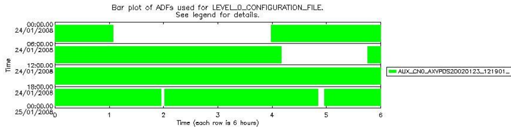
sciamachy_daily_report_level0_KSPT_L0_4303_N_20080124_6.PNG
