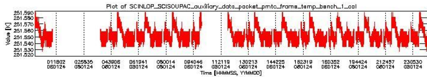
sciamachy_daily_report_level0_KSPT_L0_4303_N_20080124_0.PNG
