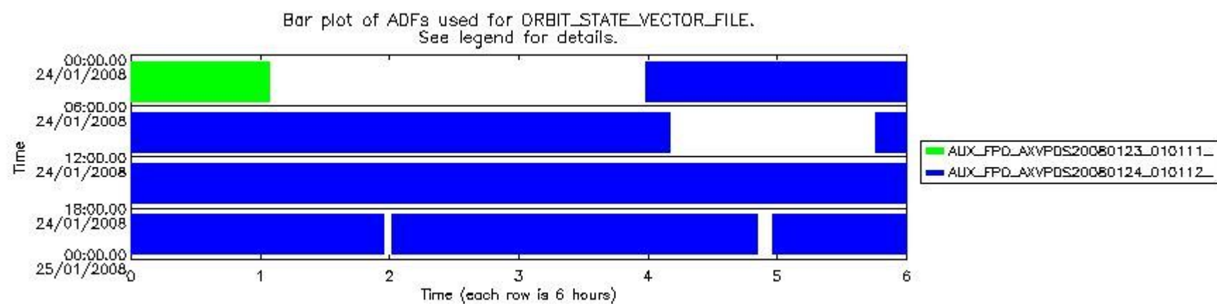
sciamachy_daily_report_level0_KSPT_L0_4303_N_20080124_7.PNG
