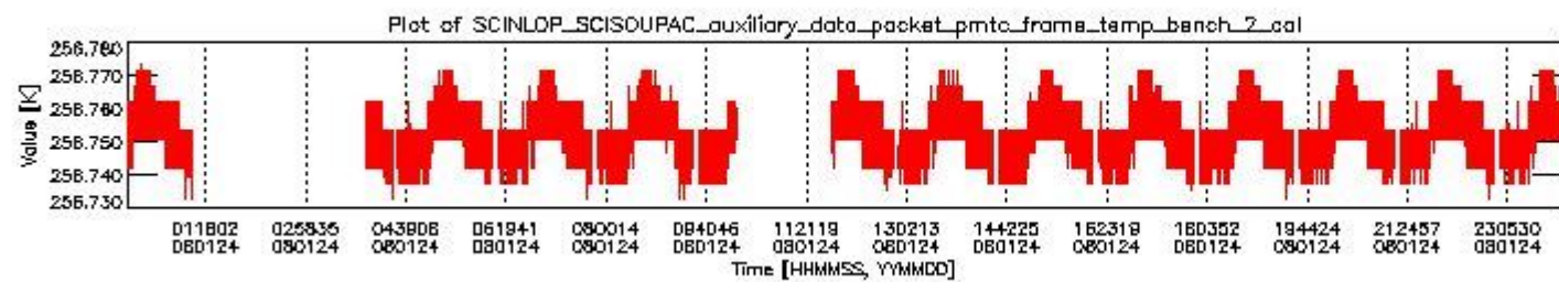
sciamachy_daily_report_level0_KSPT_L0_4303_N_20080124_1.PNG
