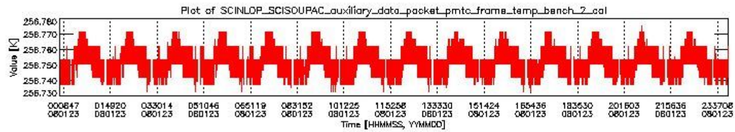
sciamachy_daily_report_level0_KSPT_L0_4303_N_20080123_1.PNG
