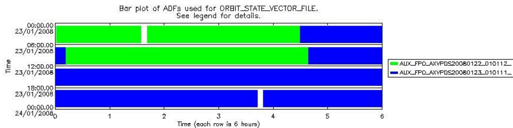
sciamachy_daily_report_level0_KSPT_L0_4303_N_20080123_7.PNG
