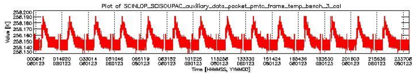
sciamachy_daily_report_level0_KSPT_L0_4303_N_20080123_2.PNG
