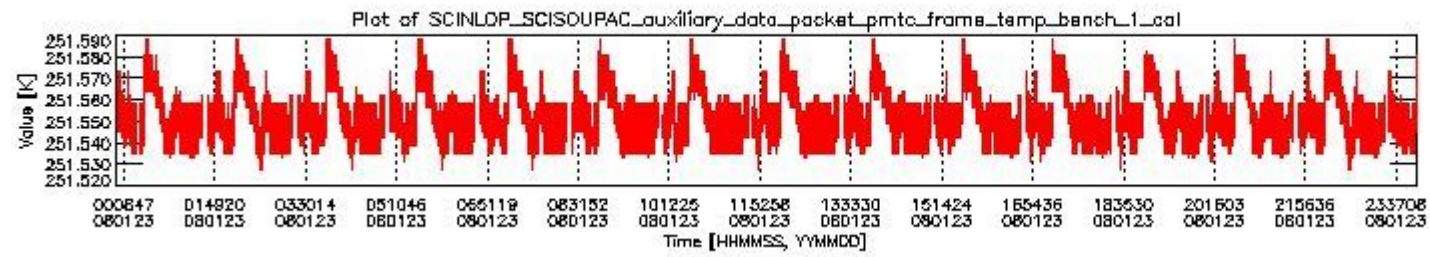
sciamachy_daily_report_level0_KSPT_L0_4303_N_20080123_0.PNG
