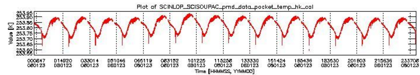
sciamachy_daily_report_level0_KSPT_L0_4303_N_20080123_3.PNG
