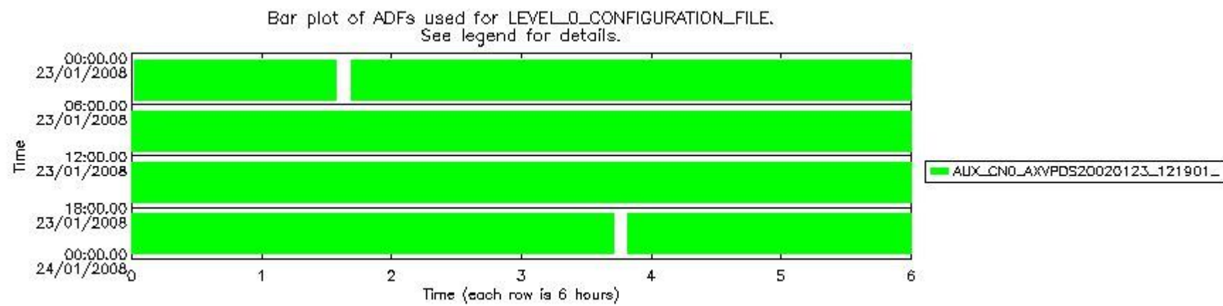
sciamachy_daily_report_level0_KSPT_L0_4303_N_20080123_6.PNG
