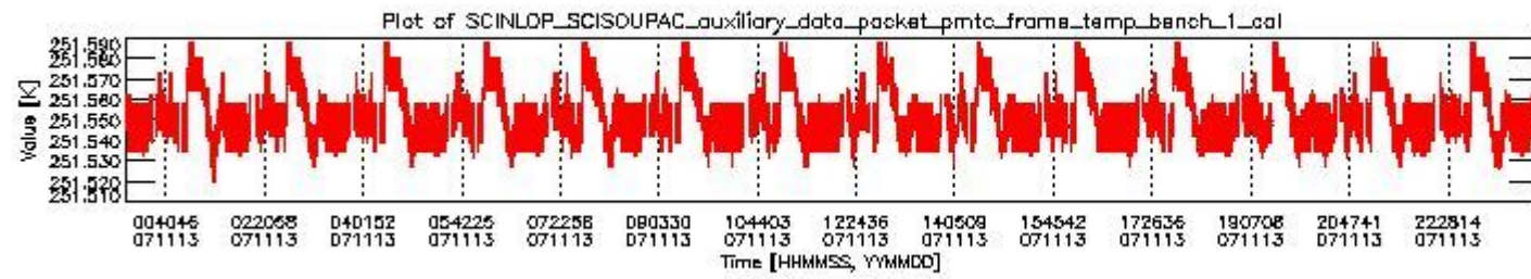
sciamachy_daily_report_level0_KSPT_L0_4302_N_20071113_0.PNG
