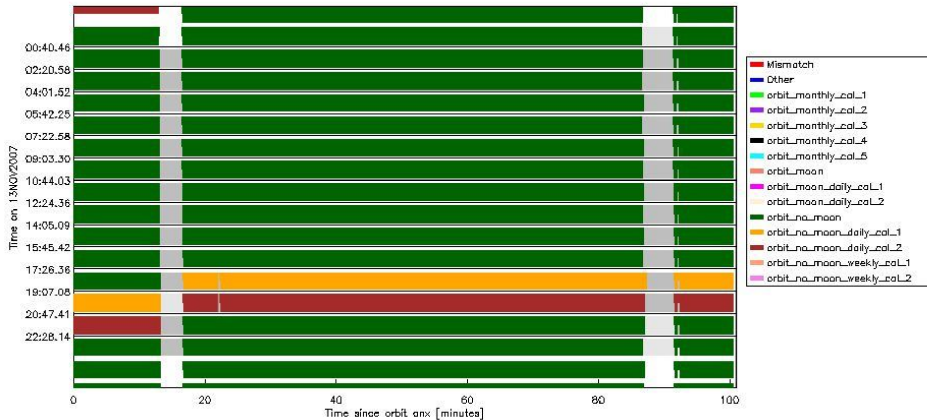
sciamachy_daily_report_level0_KSPT_L0_4302_N_20071113_6.PNG
