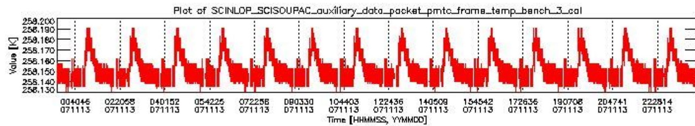
sciamachy_daily_report_level0_KSPT_L0_4302_N_20071113_2.PNG
