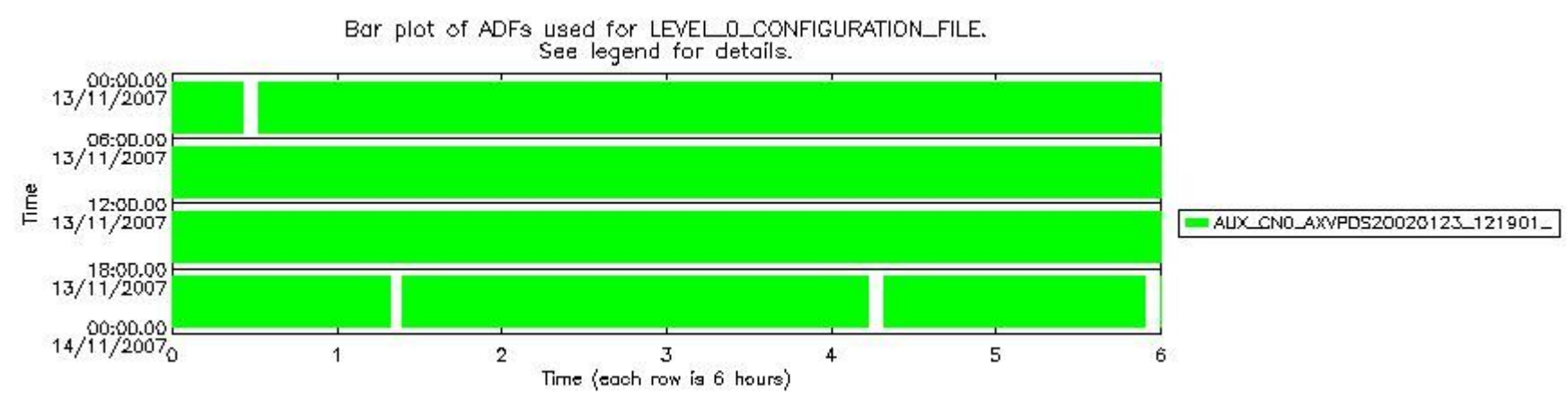
sciamachy_daily_report_level0_KSPT_L0_4302_N_20071113_7.PNG
