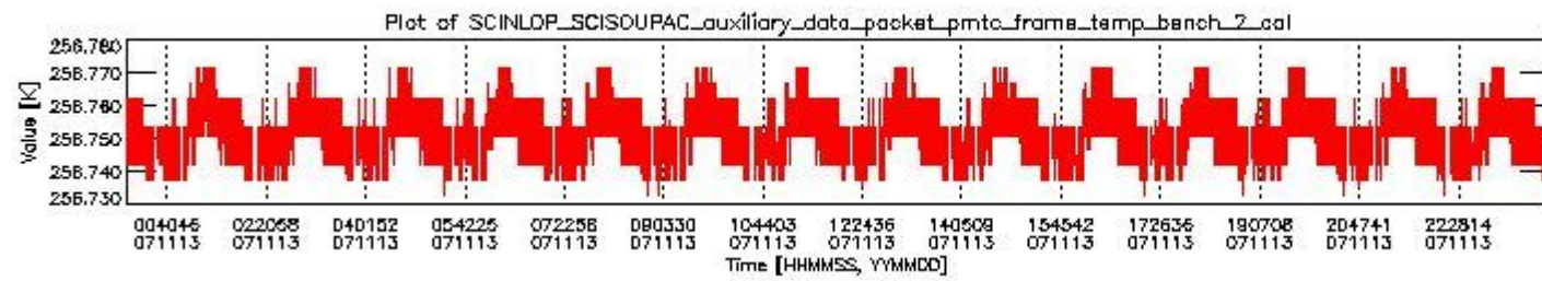
sciamachy_daily_report_level0_KSPT_L0_4302_N_20071113_1.PNG
