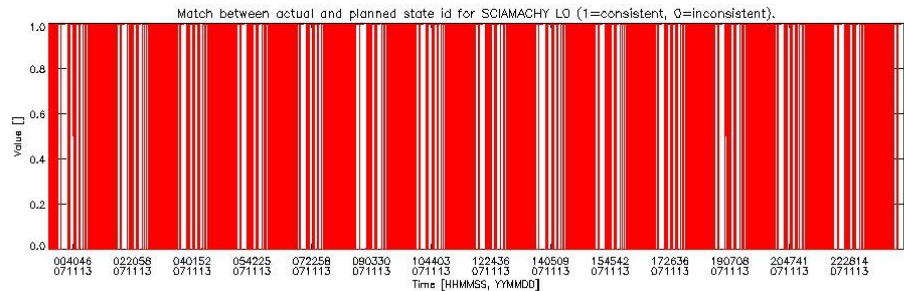
sciamachy_daily_report_level0_KSPT_L0_4302_N_20071113_5.PNG
