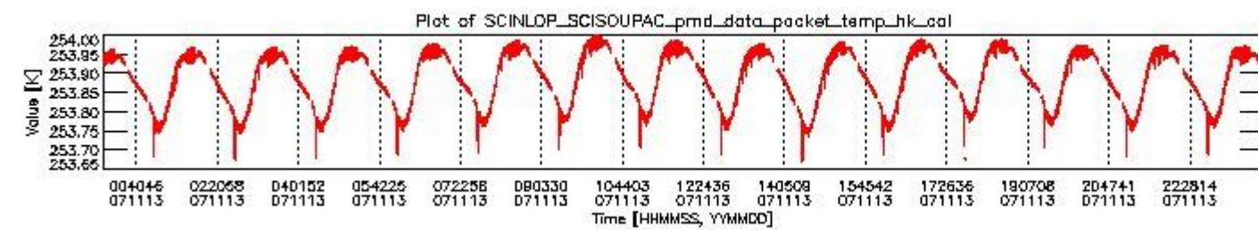
sciamachy_daily_report_level0_KSPT_L0_4302_N_20071113_3.PNG
