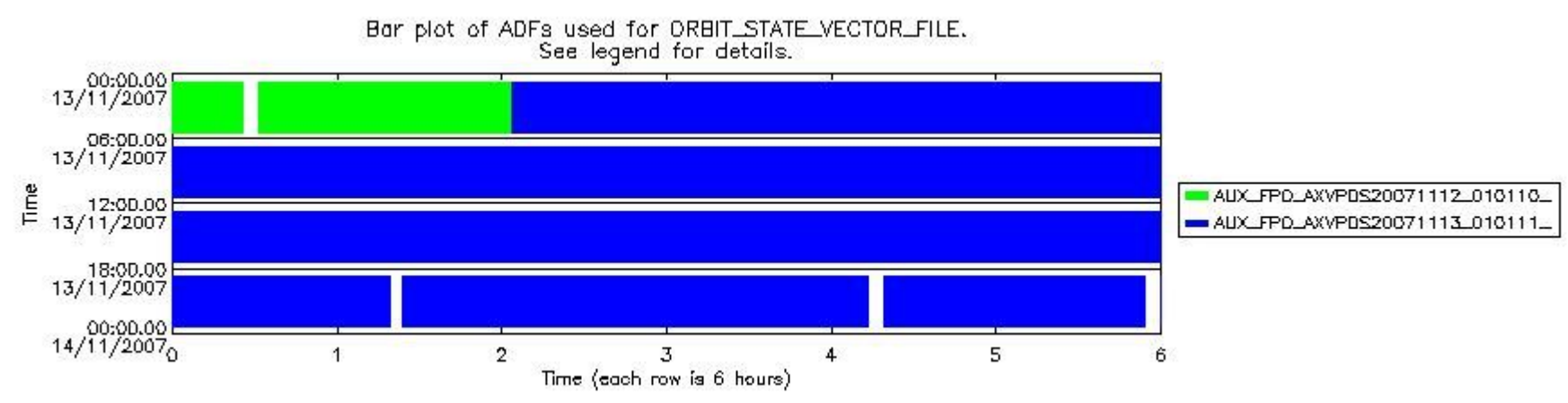
sciamachy_daily_report_level0_KSPT_L0_4302_N_20071113_8.PNG
