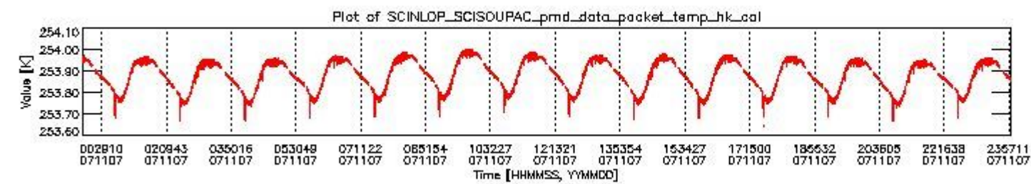
sciamachy_daily_report_level0_KSPT_L0_4302_N_20071107_3.PNG
