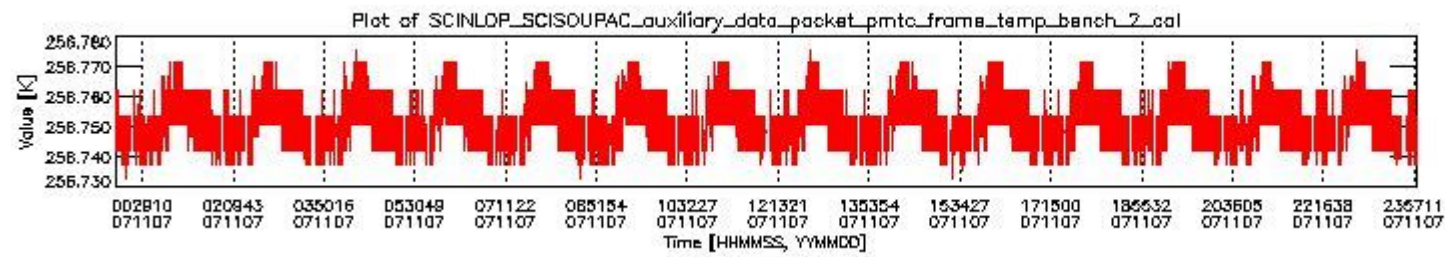
sciamachy_daily_report_level0_KSPT_L0_4302_N_20071107_1.PNG
