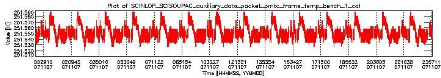
sciamachy_daily_report_level0_KSPT_L0_4302_N_20071107_0.PNG
