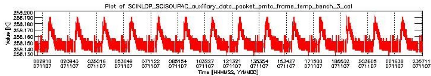
sciamachy_daily_report_level0_KSPT_L0_4302_N_20071107_2.PNG
