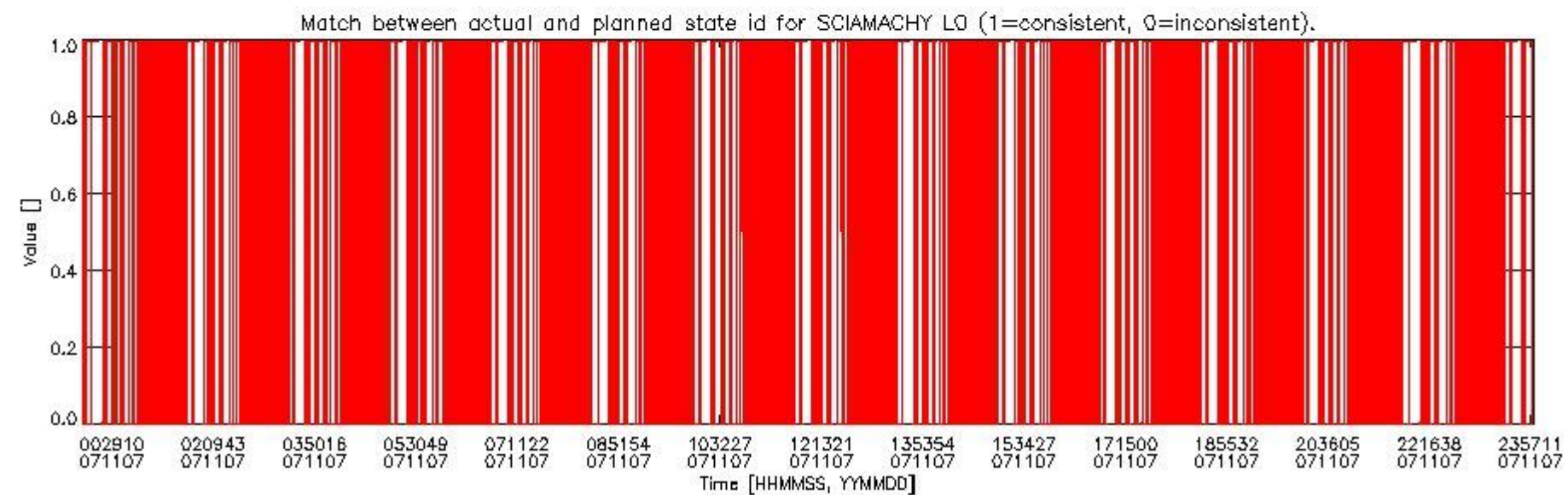
sciamachy_daily_report_level0_KSPT_L0_4302_N_20071107_5.PNG
