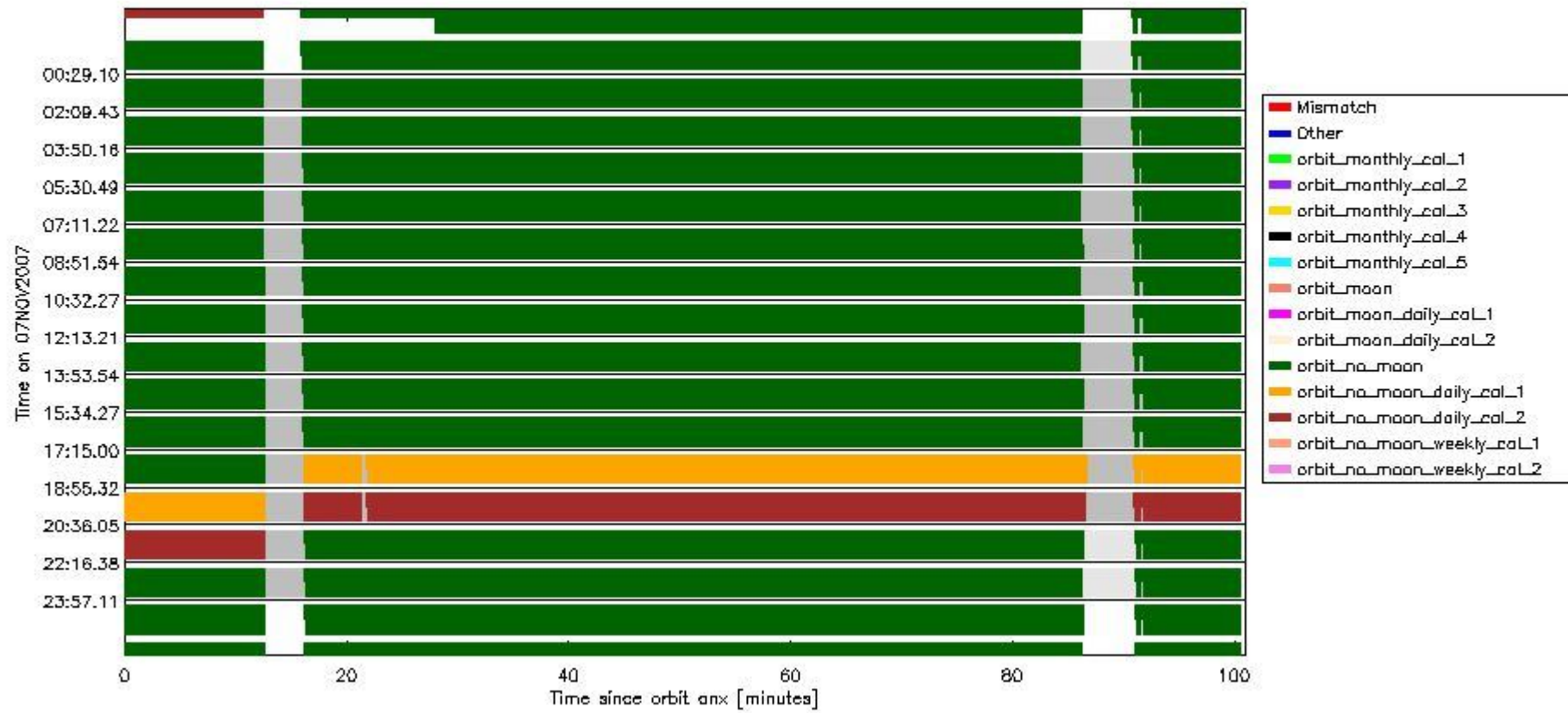
sciamachy_daily_report_level0_KSPT_L0_4302_N_20071107_6.PNG
