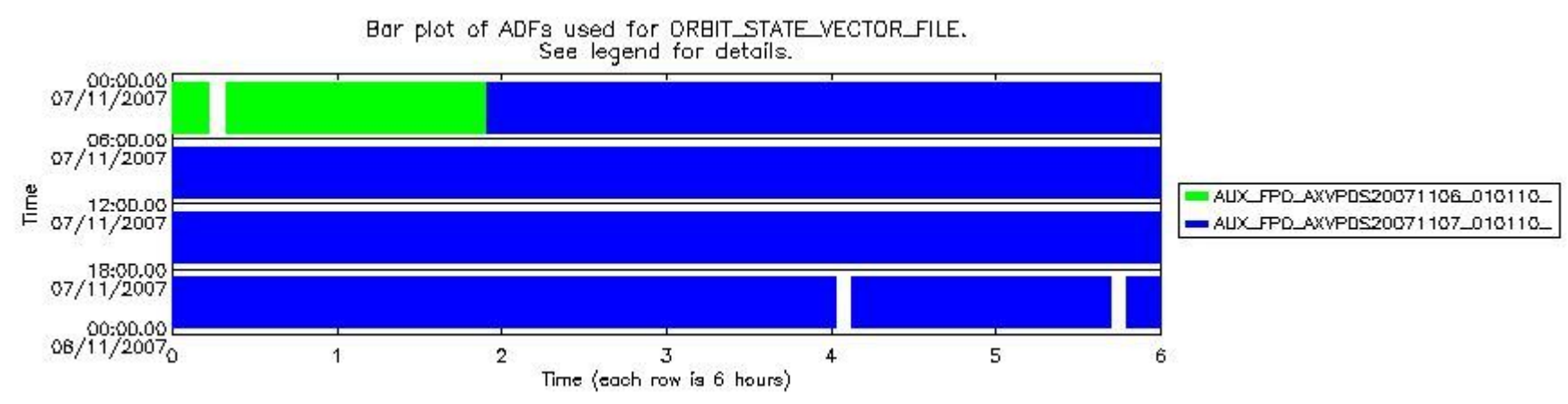
sciamachy_daily_report_level0_KSPT_L0_4302_N_20071107_8.PNG
