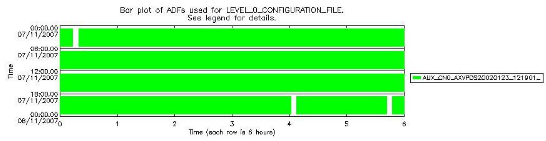
sciamachy_daily_report_level0_KSPT_L0_4302_N_20071107_7.PNG
