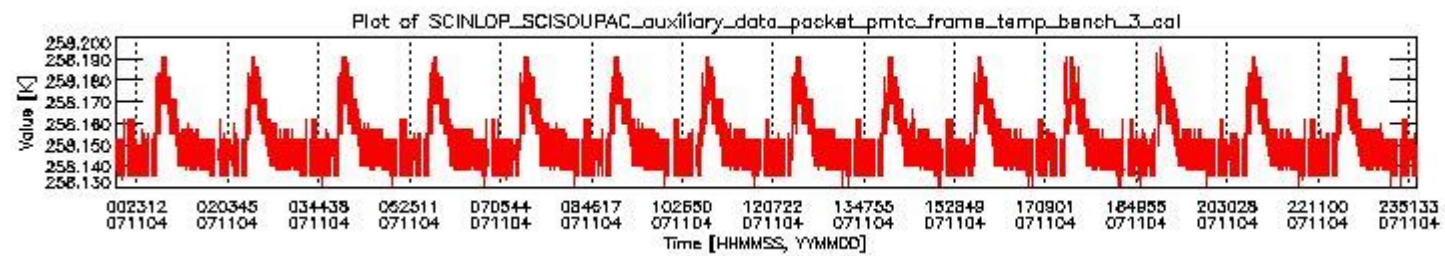
sciamachy_daily_report_level0_KSPT_L0_4302_N_20071104_2.PNG
