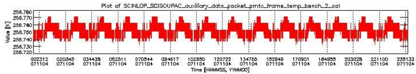
sciamachy_daily_report_level0_KSPT_L0_4302_N_20071104_1.PNG
