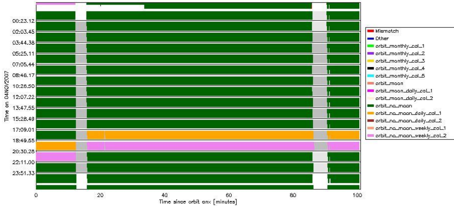
sciamachy_daily_report_level0_KSPT_L0_4302_N_20071104_6.PNG
