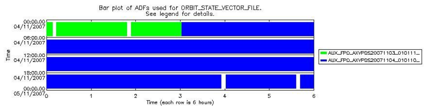
sciamachy_daily_report_level0_KSPT_L0_4302_N_20071104_8.PNG
