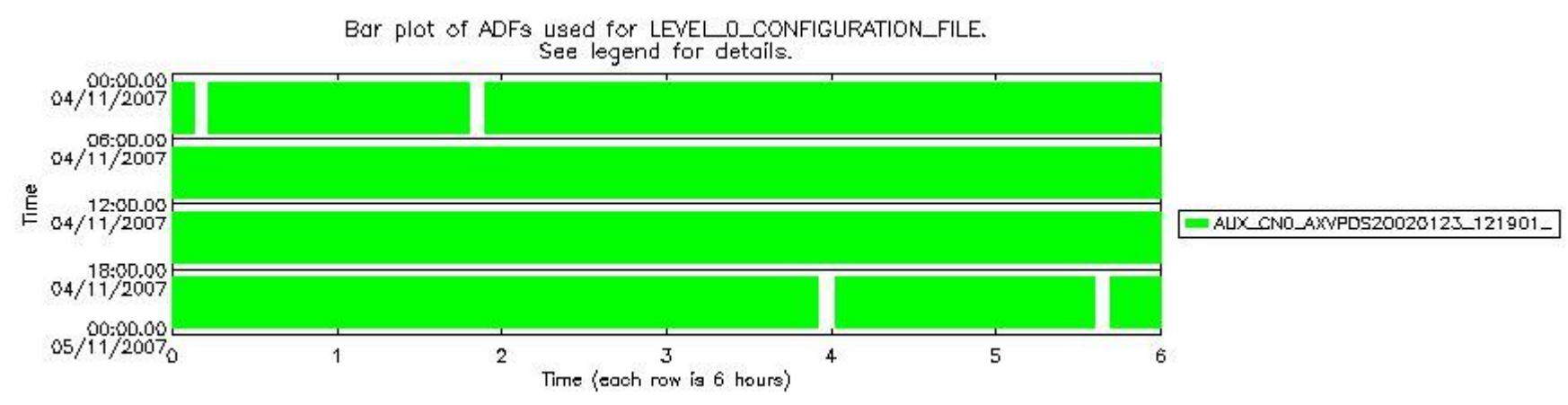
sciamachy_daily_report_level0_KSPT_L0_4302_N_20071104_7.PNG
