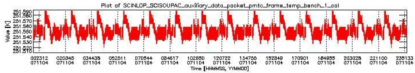
sciamachy_daily_report_level0_KSPT_L0_4302_N_20071104_0.PNG
