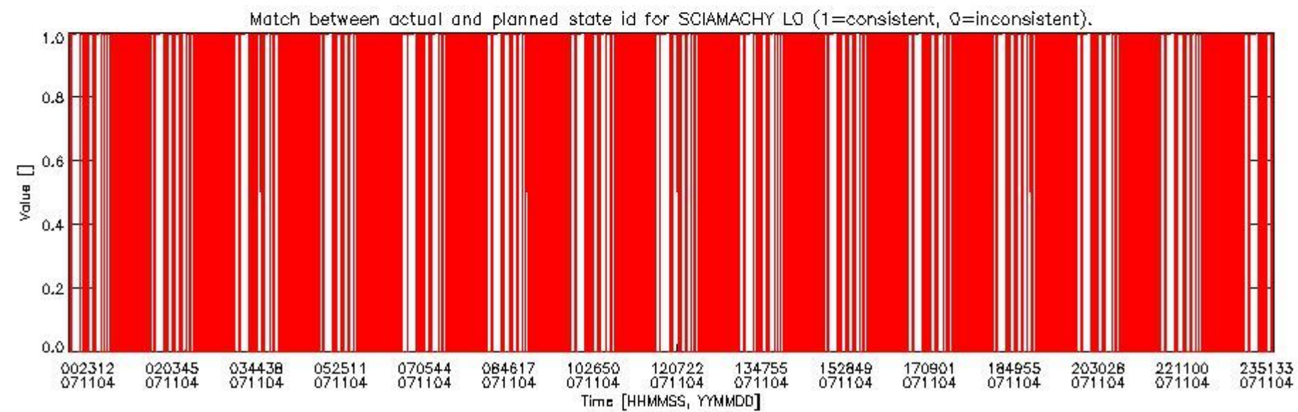
sciamachy_daily_report_level0_KSPT_L0_4302_N_20071104_5.PNG
