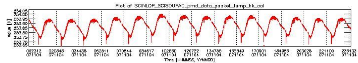
sciamachy_daily_report_level0_KSPT_L0_4302_N_20071104_3.PNG
