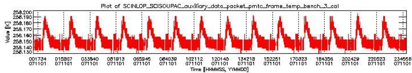
sciamachy_daily_report_level0_KSPT_L0_4302_N_20071101_2.PNG
