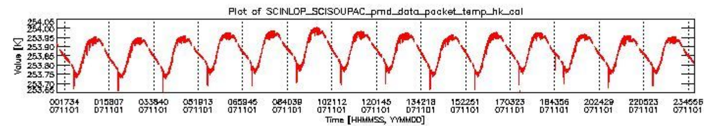
sciamachy_daily_report_level0_KSPT_L0_4302_N_20071101_3.PNG
