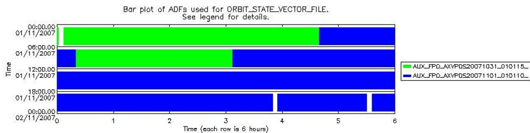
sciamachy_daily_report_level0_KSPT_L0_4302_N_20071101_8.PNG
