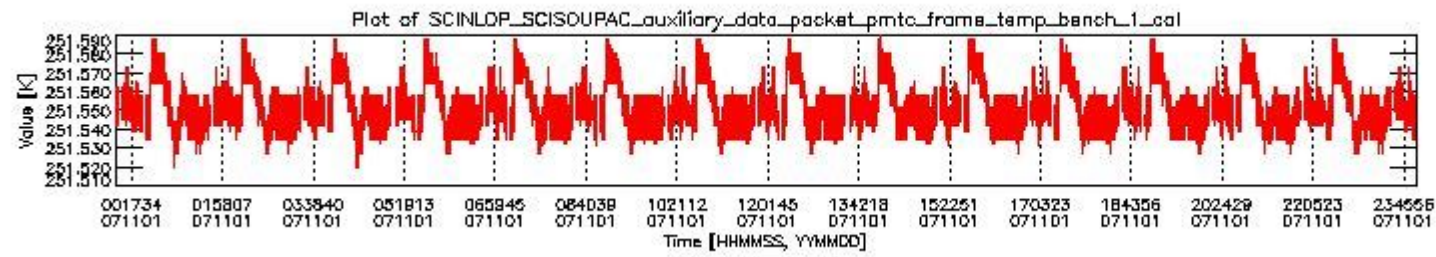
sciamachy_daily_report_level0_KSPT_L0_4302_N_20071101_0.PNG
