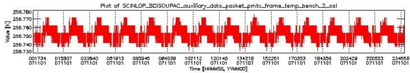
sciamachy_daily_report_level0_KSPT_L0_4302_N_20071101_1.PNG
