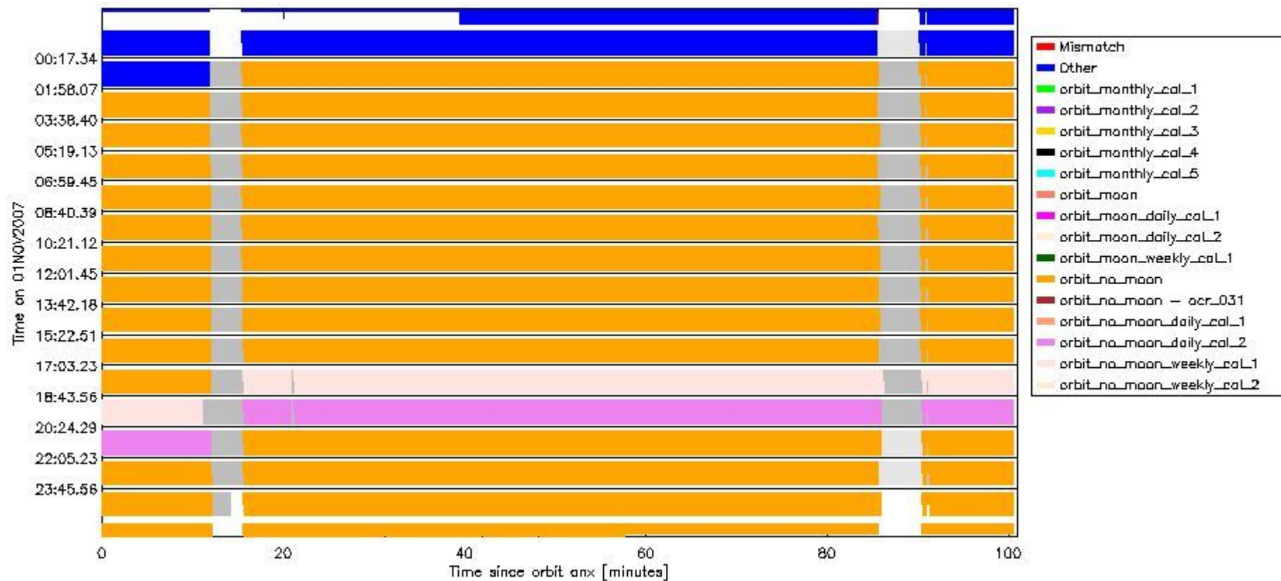
sciamachy_daily_report_level0_KSPT_L0_4302_N_20071101_6.PNG
