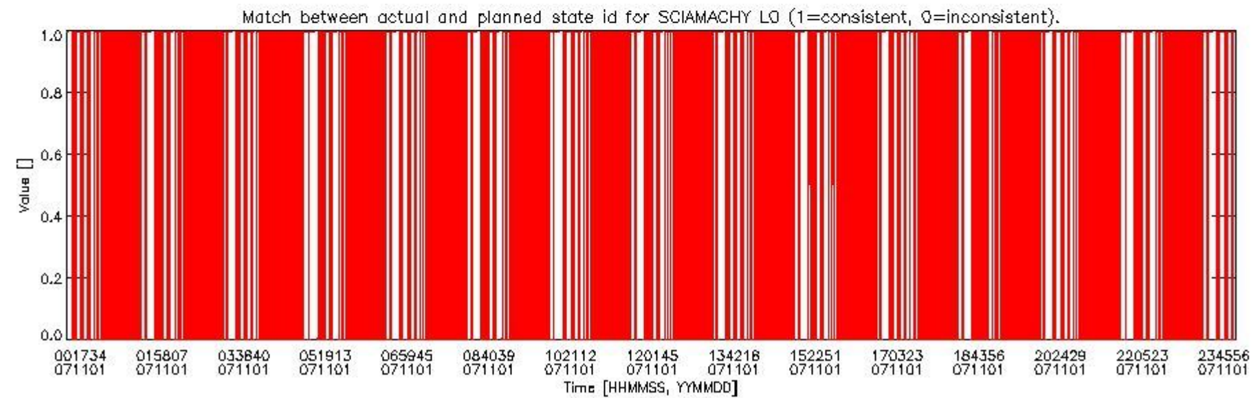
sciamachy_daily_report_level0_KSPT_L0_4302_N_20071101_5.PNG
