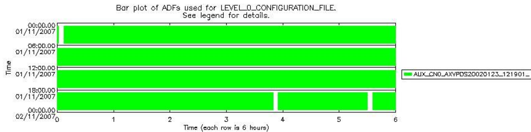
sciamachy_daily_report_level0_KSPT_L0_4302_N_20071101_7.PNG
