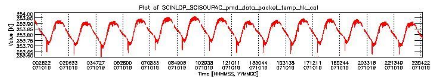
sciamachy_daily_report_level0_KSPT_L0_4302_N_20071019_3.PNG
