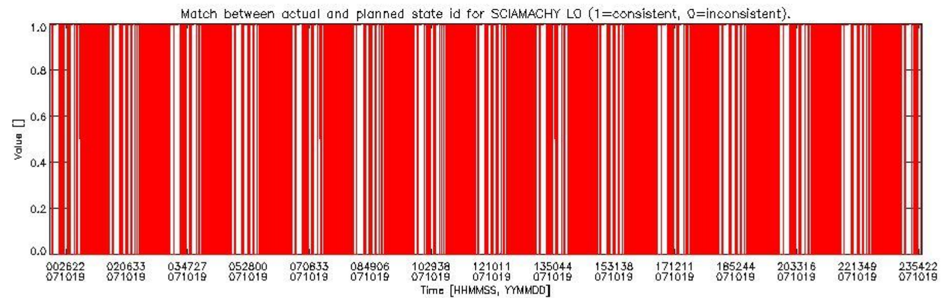
sciamachy_daily_report_level0_KSPT_L0_4302_N_20071019_5.PNG
