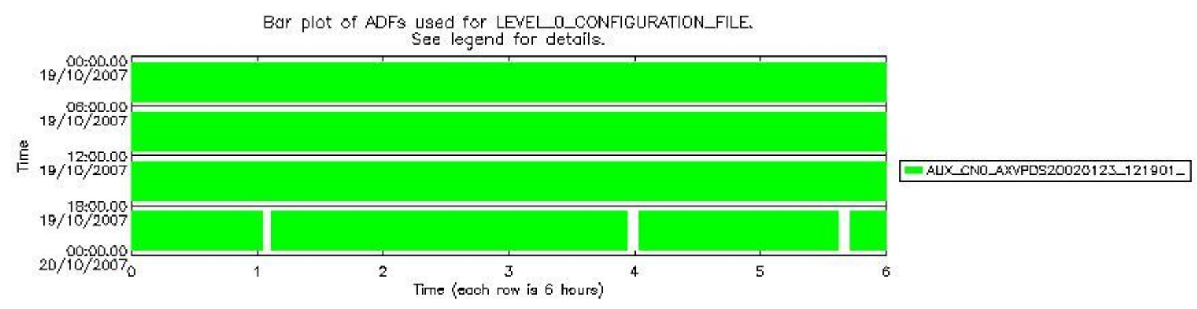
sciamachy_daily_report_level0_KSPT_L0_4302_N_20071019_7.PNG
