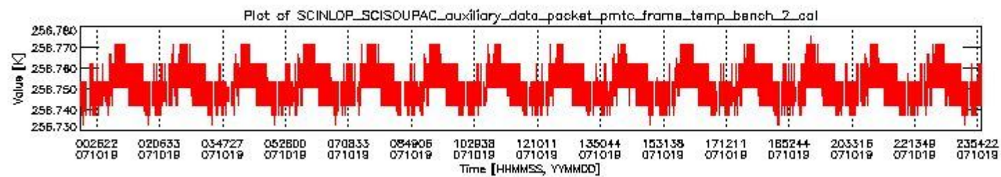
sciamachy_daily_report_level0_KSPT_L0_4302_N_20071019_1.PNG
