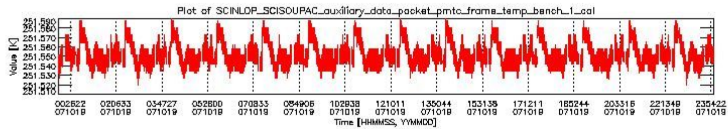
sciamachy_daily_report_level0_KSPT_L0_4302_N_20071019_0.PNG
