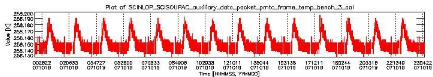
sciamachy_daily_report_level0_KSPT_L0_4302_N_20071019_2.PNG
