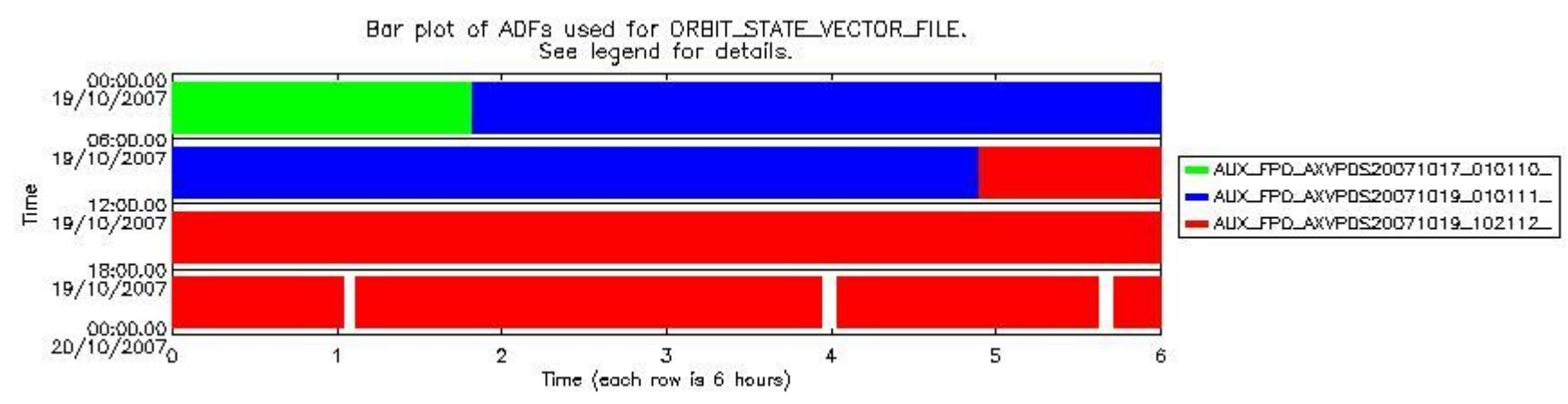
sciamachy_daily_report_level0_KSPT_L0_4302_N_20071019_8.PNG
