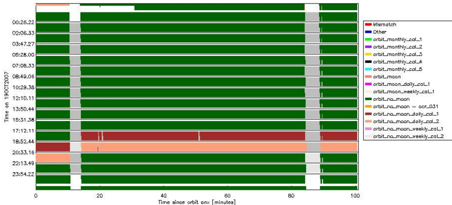
sciamachy_daily_report_level0_KSPT_L0_4302_N_20071019_6.PNG
