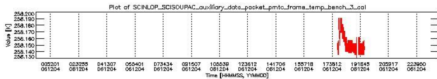
sciamachy_daily_report_level0_PFHS_5_37_N_20061204_2.PNG
