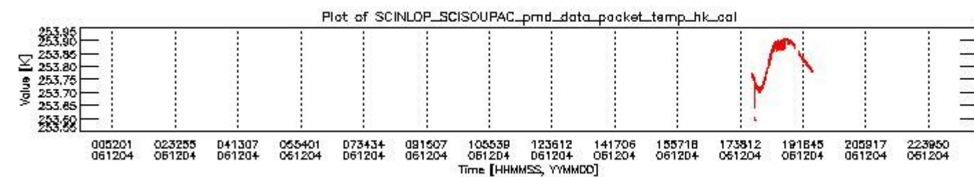
sciamachy_daily_report_level0_PFHS_5_37_N_20061204_3.PNG
