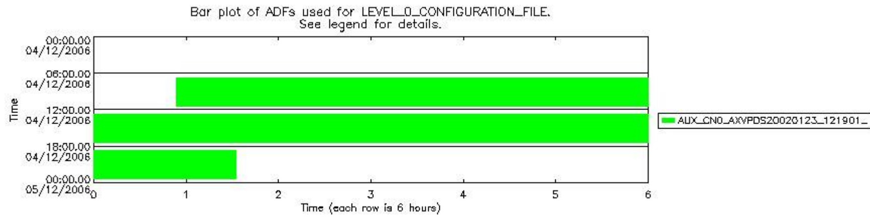
sciamachy_daily_report_level0_PPHS_5_37_N_20061204_7.PNG
