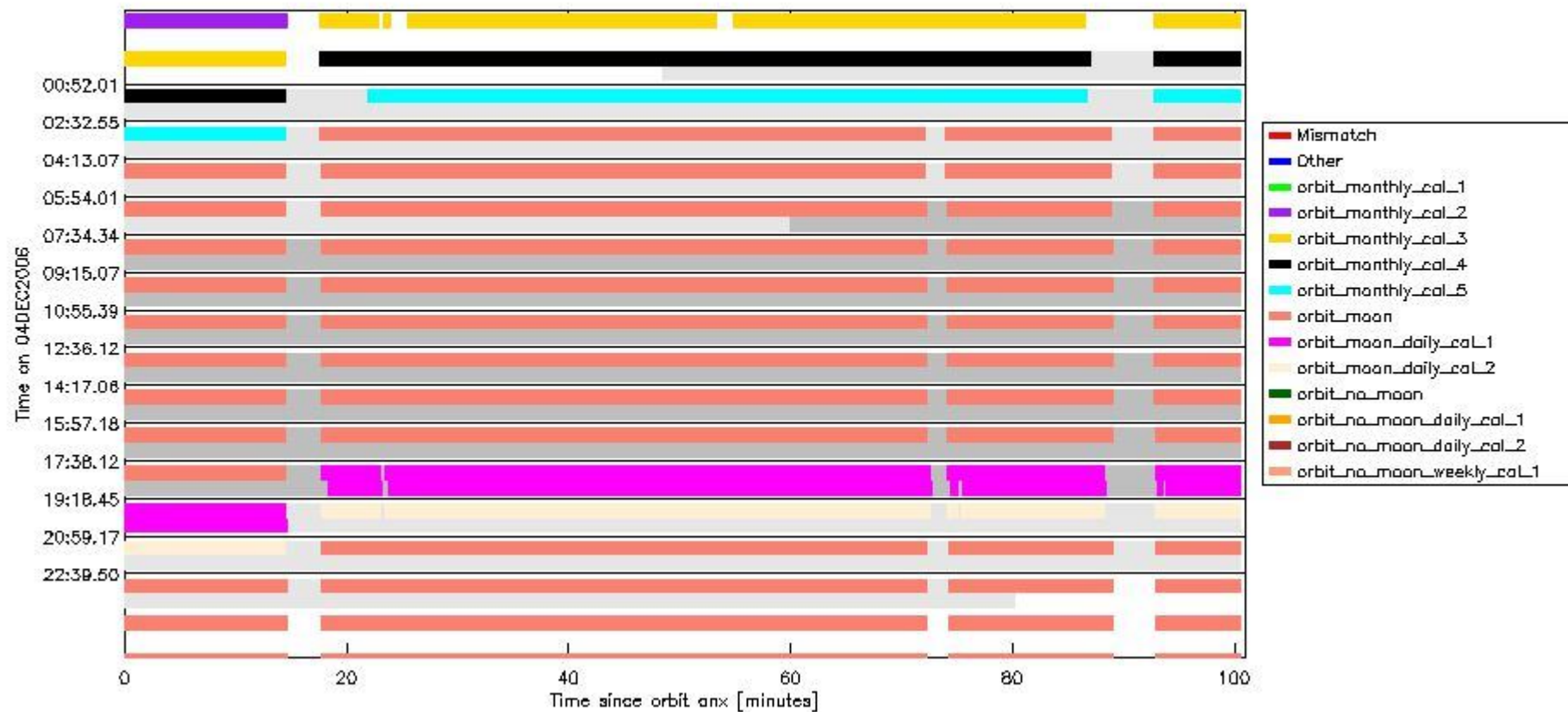
sciamachy_daily_report_level0_PFHS_5_37_N_20061204_6.PNG
