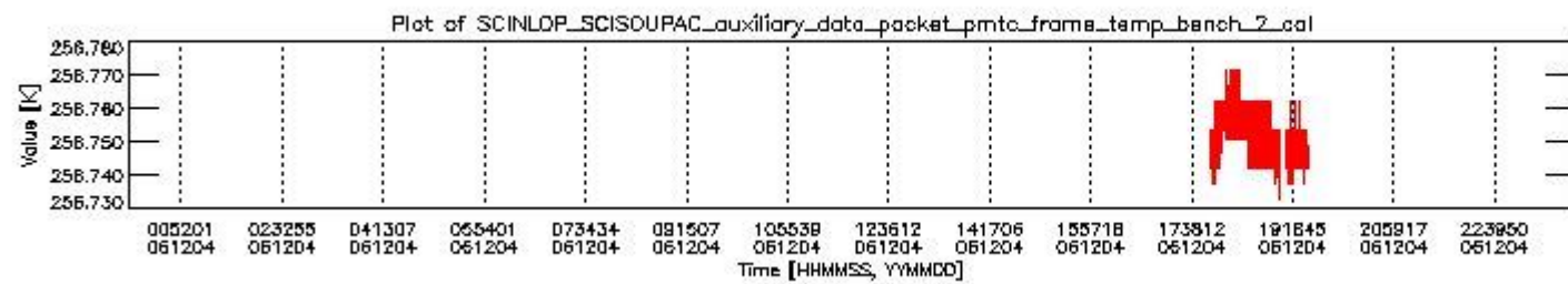
sciamachy_daily_report_level0_PFHS_5_37_N_20061204_1.PNG
