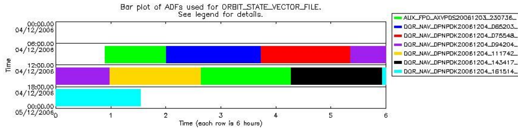
sciamachy_daily_report_level0_PPHS_5_37_N_20061204_8.PNG
