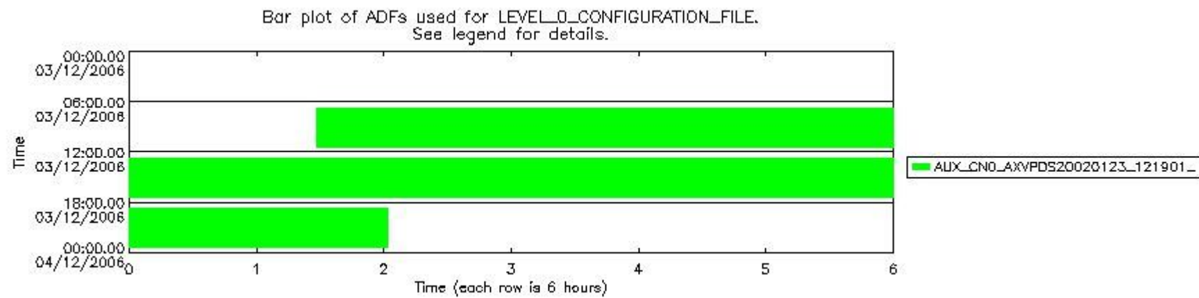
sciamachy_daily_report_level0_PFHS_5_37_N_20061203_6.PNG
