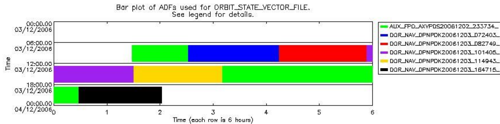
sciamachy_daily_report_level0_PFHS_5_37_N_20061203_7.PNG
