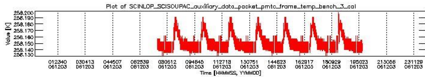
sciamachy_daily_report_level0_PFHS_5_37_N_20061203_2.PNG
