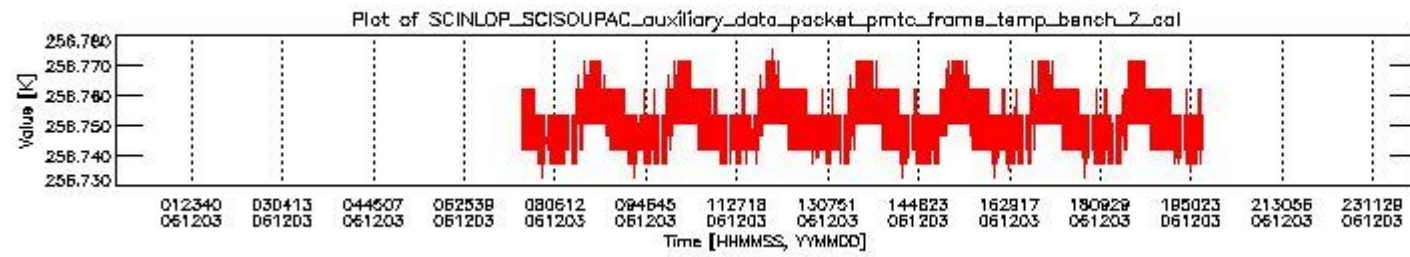
sciamachy_daily_report_level0_PFHS_5_37_N_20061203_1.PNG
