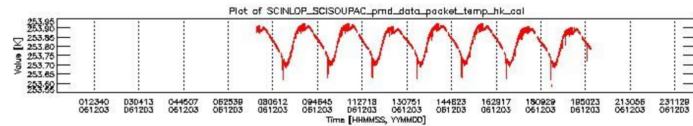
sciamachy_daily_report_level0_PFHS_5_37_N_20061203_3.PNG
