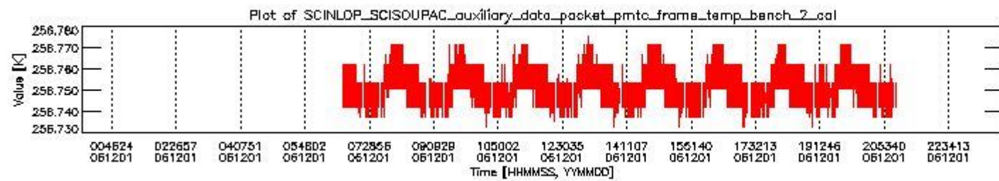
sciamachy_daily_report_level0_PFHS_5_37_N_20061201_1.PNG
