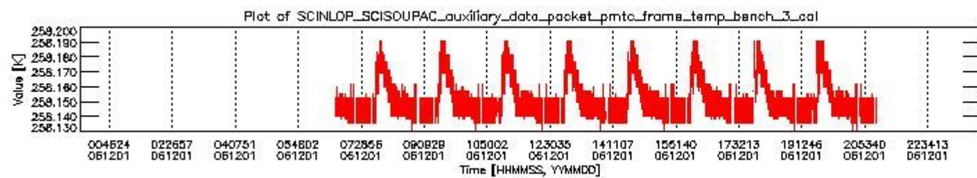
sciamachy_daily_report_level0_PFHS_5_37_N_20061201_2.PNG
