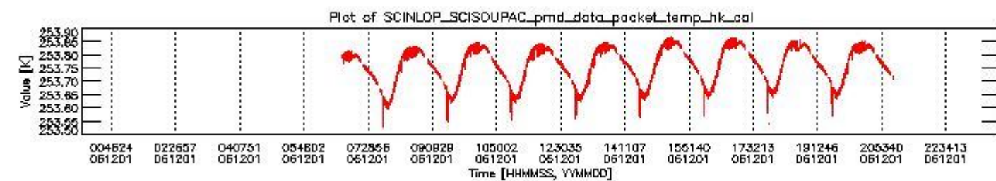
sciamachy_daily_report_level0_PFHS_5_37_N_20061201_3.PNG
