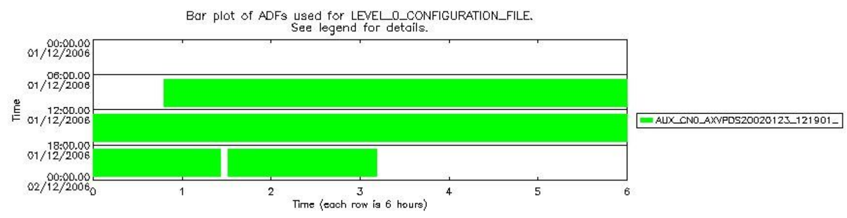
sciamachy_daily_report_level0_PFHS_5_37_N_20061201_6.PNG
