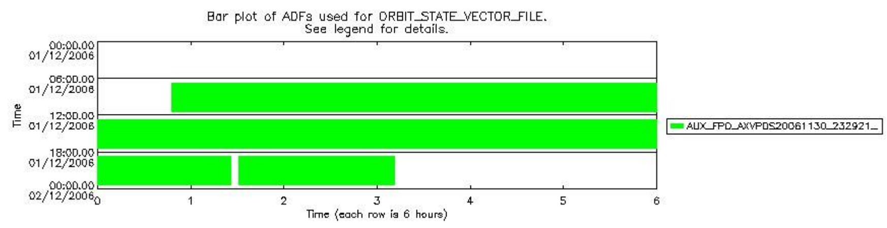
sciamachy_daily_report_level0_PFHS_5_37_N_20061201_7.PNG
