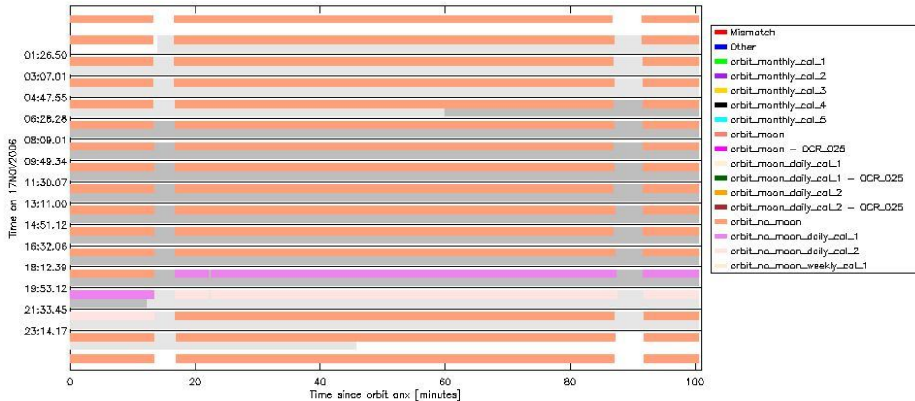
sciamachy_daily_report_level0_PFHS_5_37_N_20061117_0.PNG
