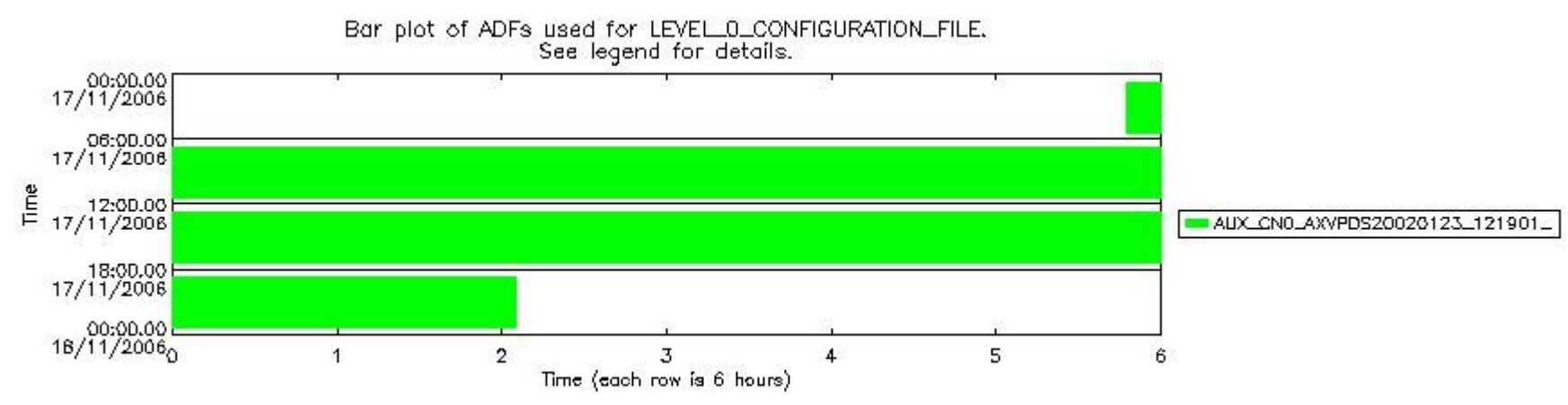
sciamachy_daily_report_level0_PFHS_5_37_N_20061117_1.PNG
