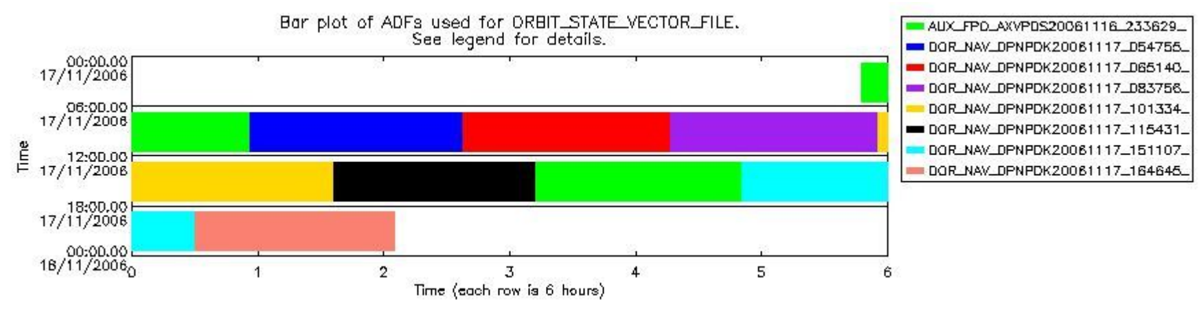
sciamachy_daily_report_level0_PFHS_5_37_N_20061117_2.PNG
