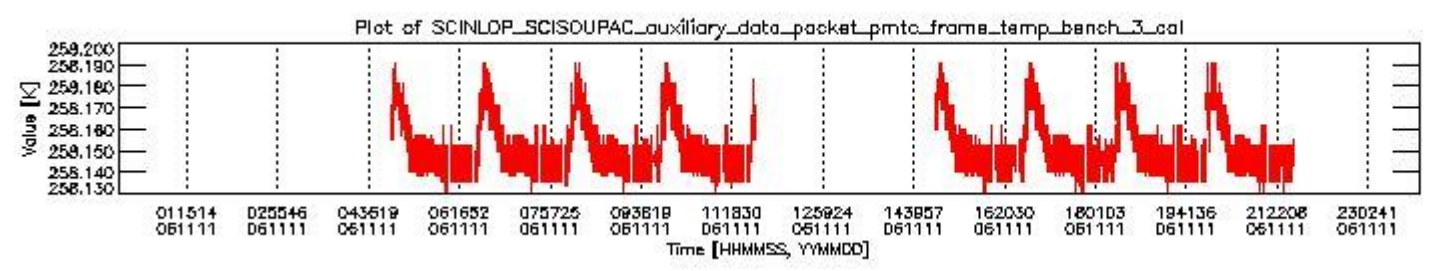
sciamachy_daily_report_level0_PFHS_5_37_N_20061111_2.PNG
