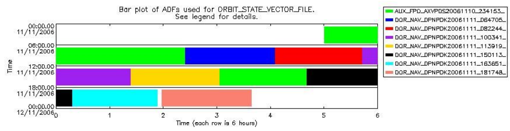
sciamachy_daily_report_level0_PPHS_5_37_N_20061111_8.PNG
