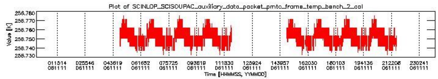
sciamachy_daily_report_level0_PFHS_5_37_N_20061111_1.PNG
