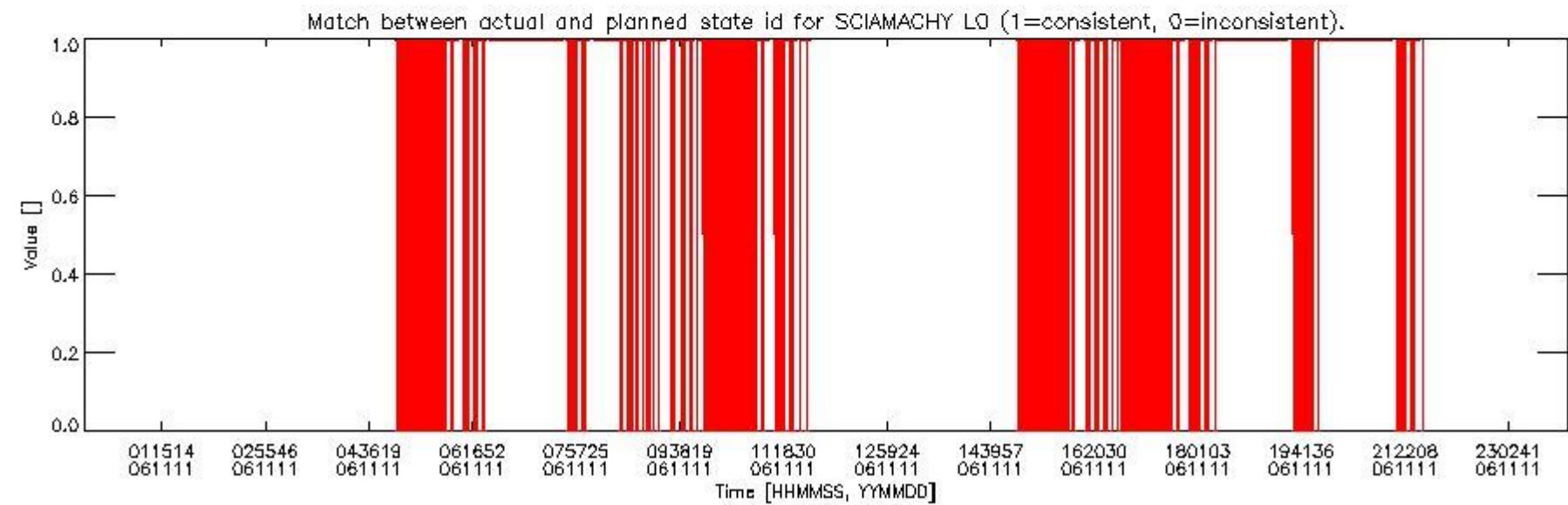
sciamachy_daily_report_level0_PFHS_5_37_N_20061111_5.PNG
