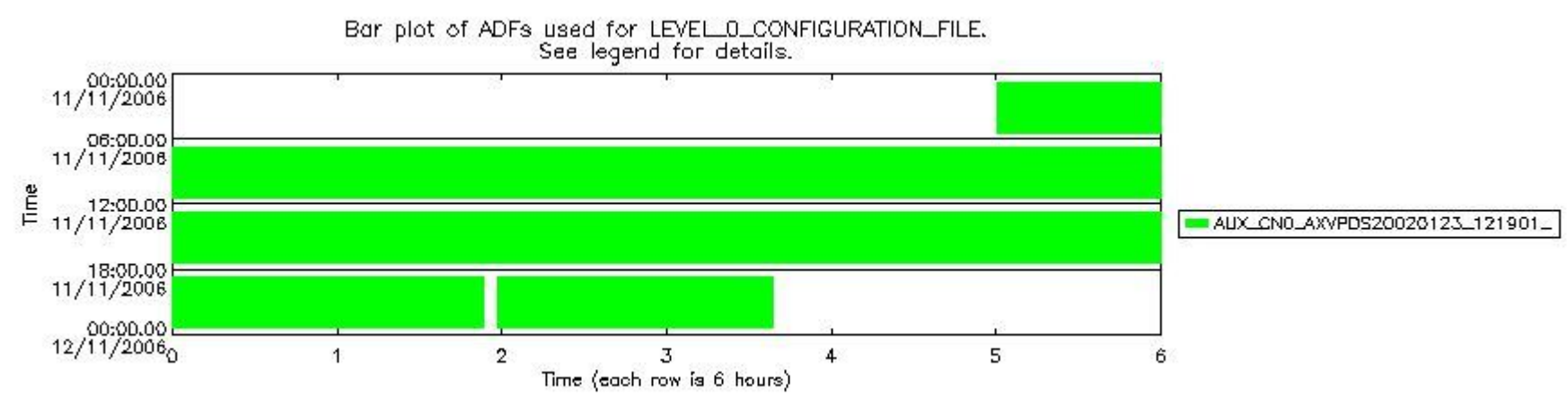
sciamachy_daily_report_level0_PPHS_5_37_N_20061111_7.PNG
