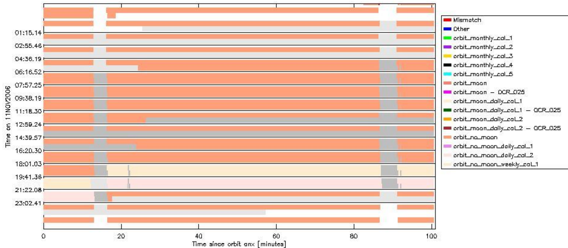
sciamachy_daily_report_level0_PPHS_5_37_N_20061111_6.PNG
