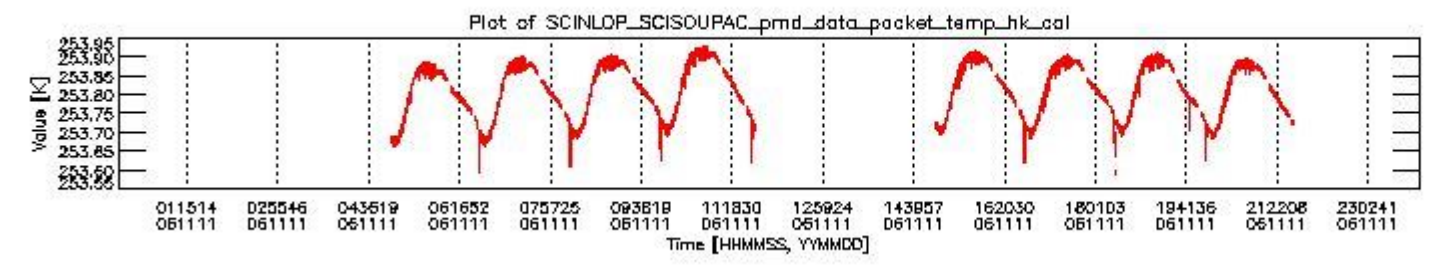
sciamachy_daily_report_level0_PFHS_5_37_N_20061111_3.PNG
