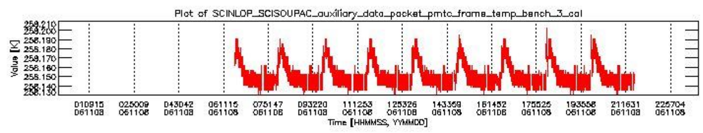
sciamachy_daily_report_level0_PFHS_5_37_N_20061108_2.PNG
