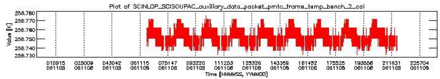
sciamachy_daily_report_level0_PFHS_5_37_N_20061108_1.PNG
