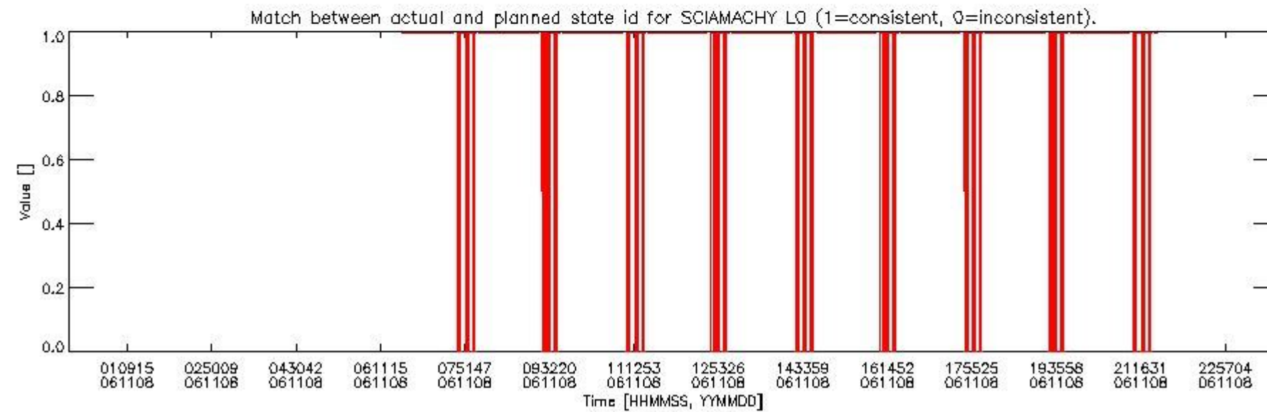
sciamachy_daily_report_level0_PFHS_5_37_N_20061108_5.PNG
