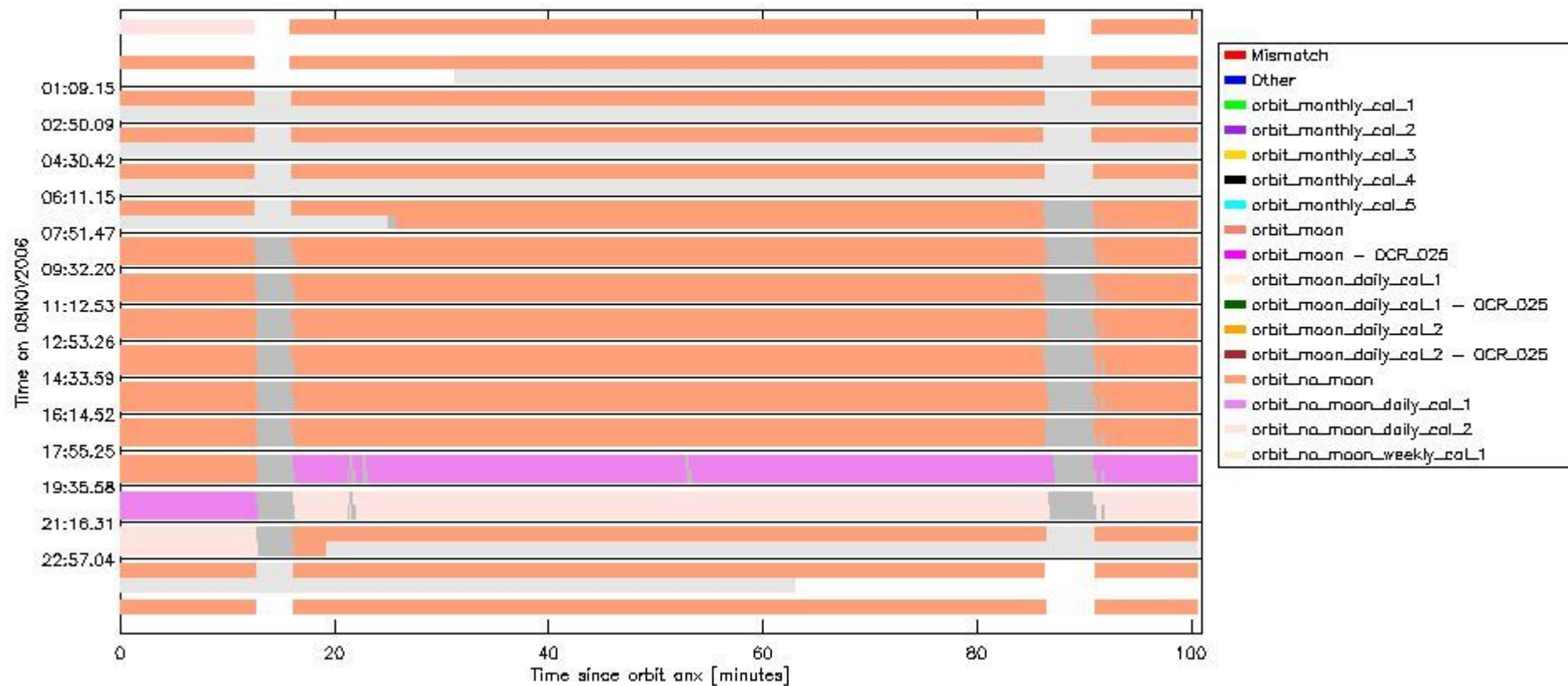
sciamachy_daily_report_level0_PPHS_5_37_N_20061108_6.PNG
