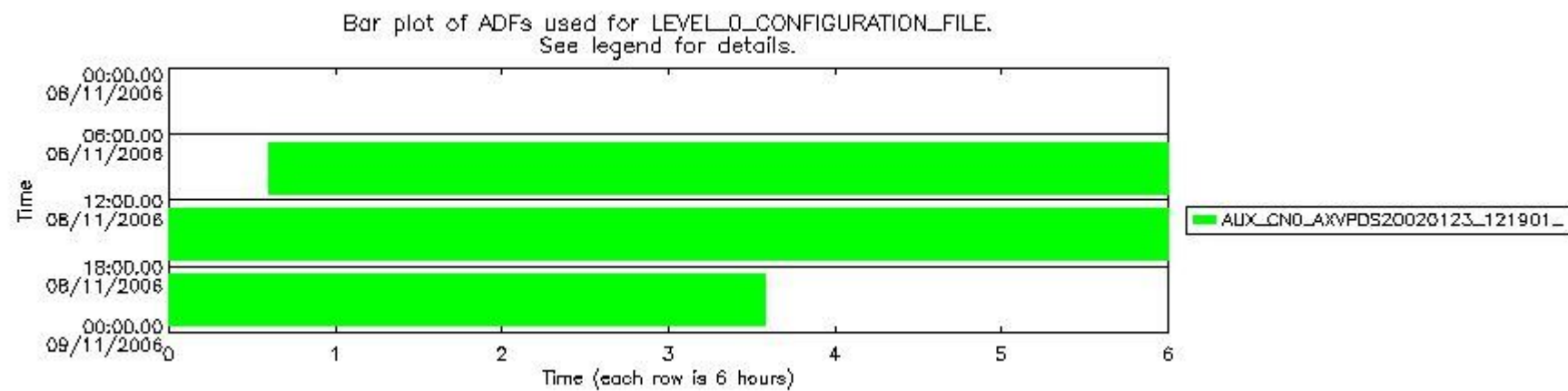
sciamachy_daily_report_level0_PPHS_5_37_N_20061108_7.PNG
