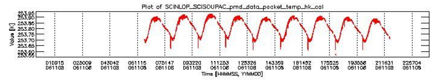
sciamachy_daily_report_level0_PFHS_5_37_N_20061108_3.PNG
