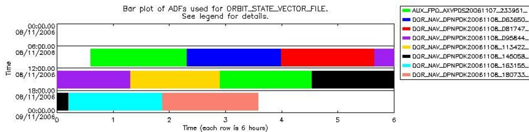
sciamachy_daily_report_level0_PPHS_5_37_N_20061108_8.PNG
