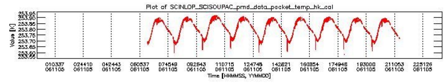
sciamachy_daily_report_level0_PFHS_5_37_N_20061105_3.PNG
