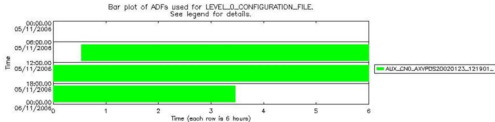
sciamachy_daily_report_level0_PFHS_5_37_N_20061105_6.PNG
