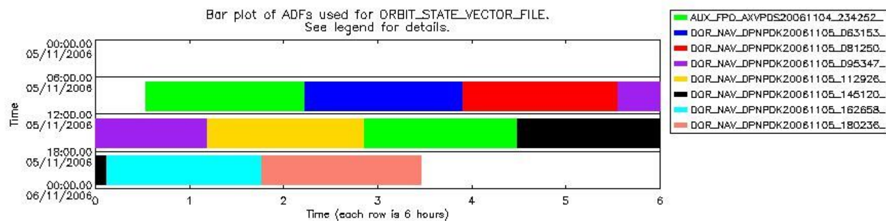
sciamachy_daily_report_level0_PFHS_5_37_N_20061105_7.PNG
