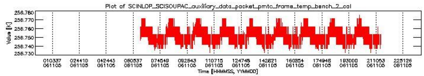
sciamachy_daily_report_level0_PFHS_5_37_N_20061105_1.PNG
