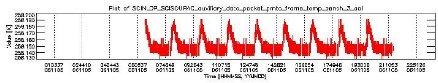
sciamachy_daily_report_level0_PFHS_5_37_N_20061105_2.PNG
