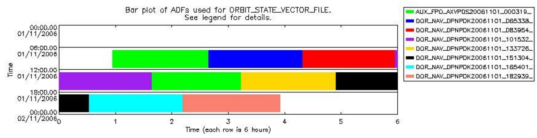
sciamachy_daily_report_level0_PPHS_5_37_N_20061101_8.PNG
