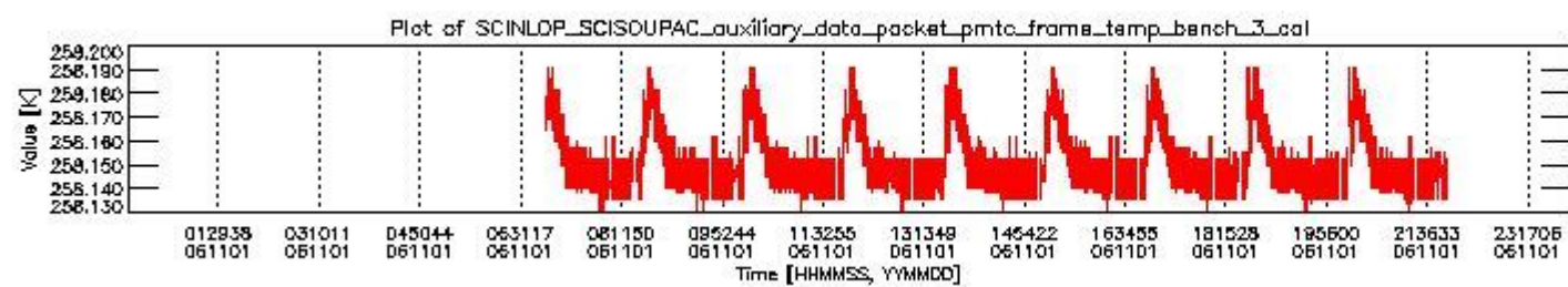
sciamachy_daily_report_level0_PFHS_5_37_N_20061101_2.PNG
