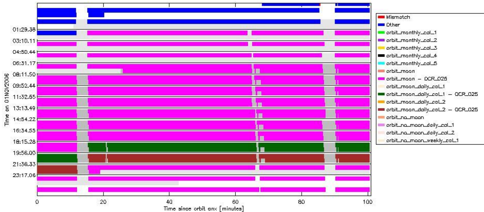
sciamachy_daily_report_level0_PPHS_5_37_N_20061101_6.PNG
