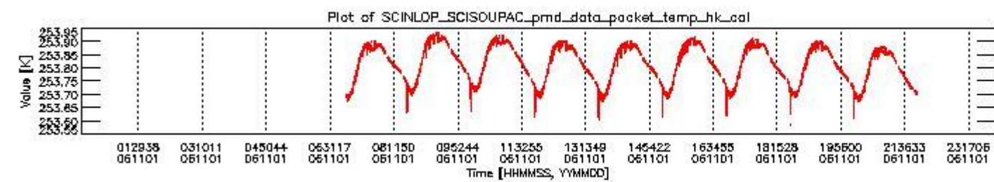
sciamachy_daily_report_level0_PFHS_5_37_N_20061101_3.PNG
