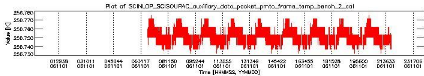
sciamachy_daily_report_level0_PFHS_5_37_N_20061101_1.PNG
