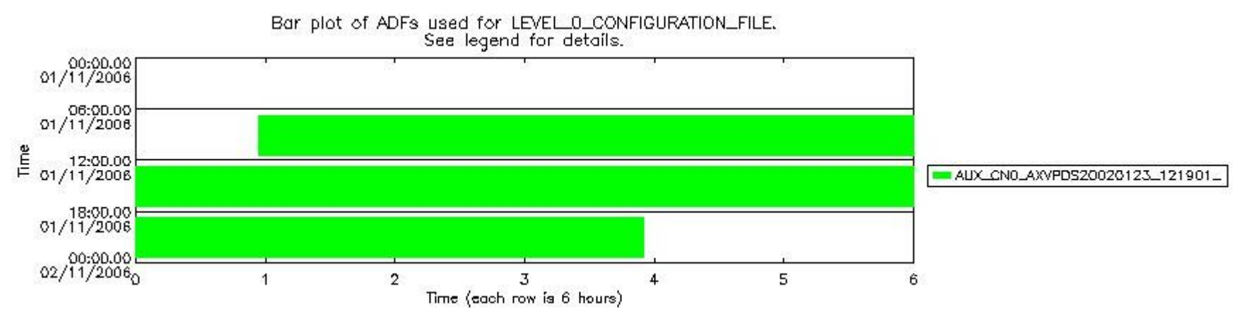
sciamachy_daily_report_level0_PPHS_5_37_N_20061101_7.PNG
