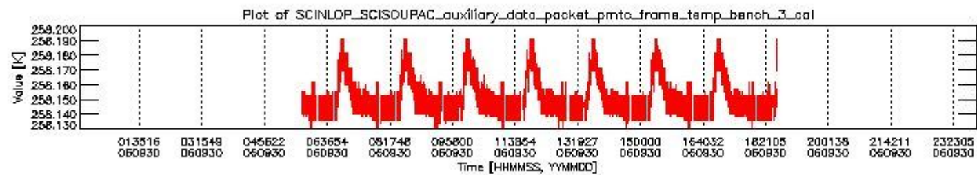
sciamachy_daily_report_level0_PFHS_5_37_N_20060930_2.PNG
