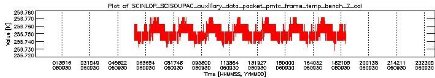
sciamachy_daily_report_level0_PFHS_5_37_N_20060930_1.PNG
