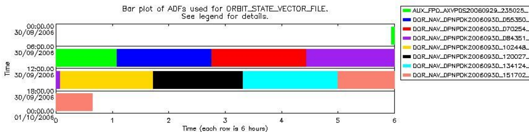
sciamachy_daily_report_level0_PFHS_5_37_N_20060930_5.PNG
