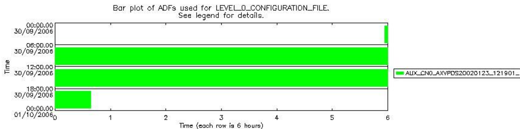
sciamachy_daily_report_level0_PFHS_5_37_N_20060930_4.PNG
