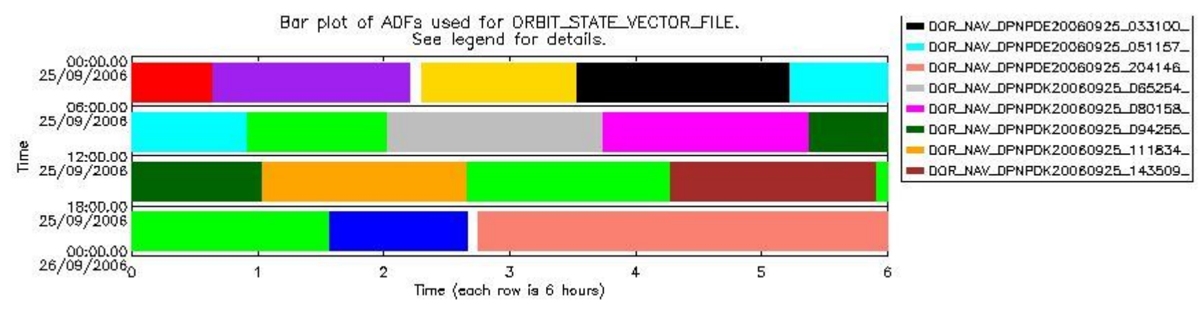
sciamachy_daily_report_level0_PFHS_5_37_N_20060925_8.PNG
