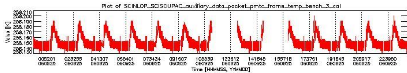
sciamachy_daily_report_level0_PFHS_5_37_N_20060925_2.PNG
