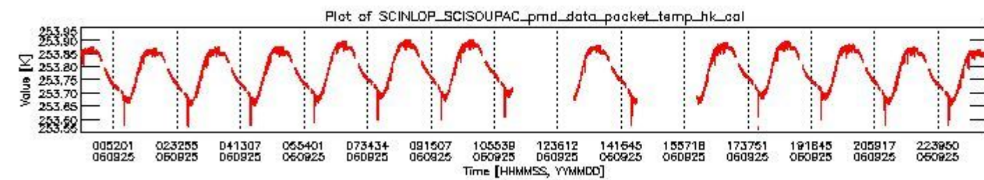
sciamachy_daily_report_level0_PFHS_5_37_N_20060925_3.PNG
