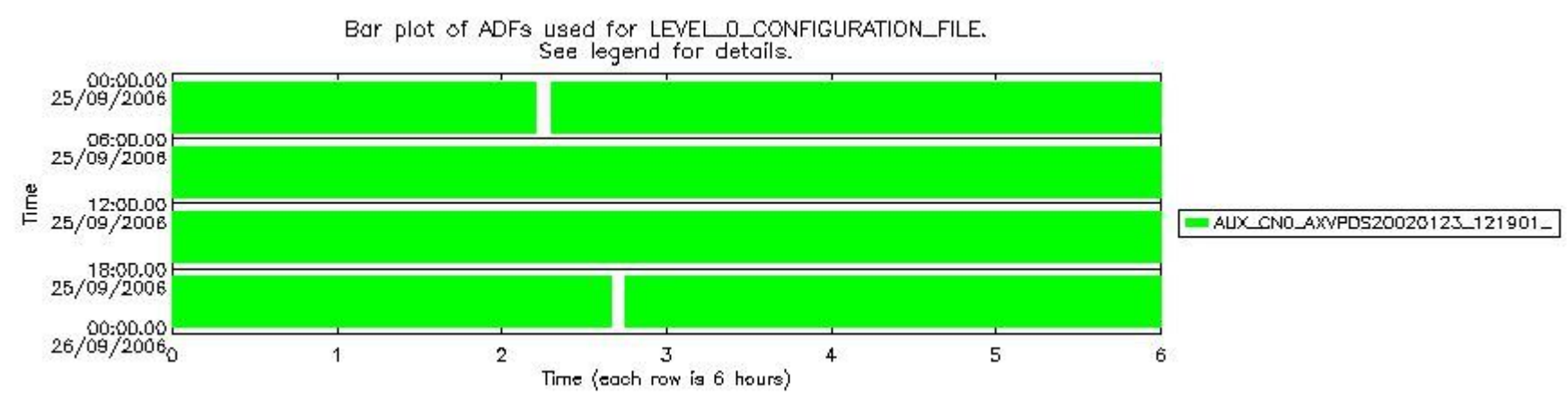
sciamachy_daily_report_level0_PFHS_5_37_N_20060925_7.PNG
