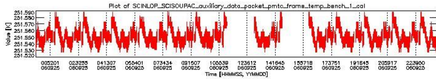
sciamachy_daily_report_level0_PFHS_5_37_N_20060925_0.PNG
