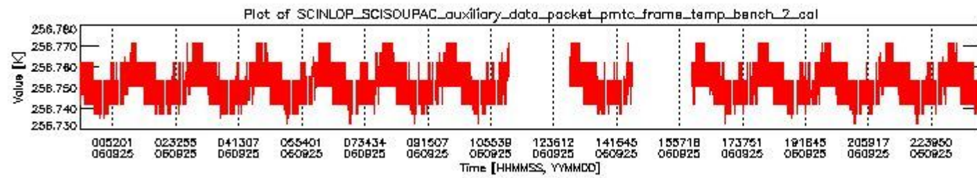
sciamachy_daily_report_level0_PFHS_5_37_N_20060925_1.PNG
