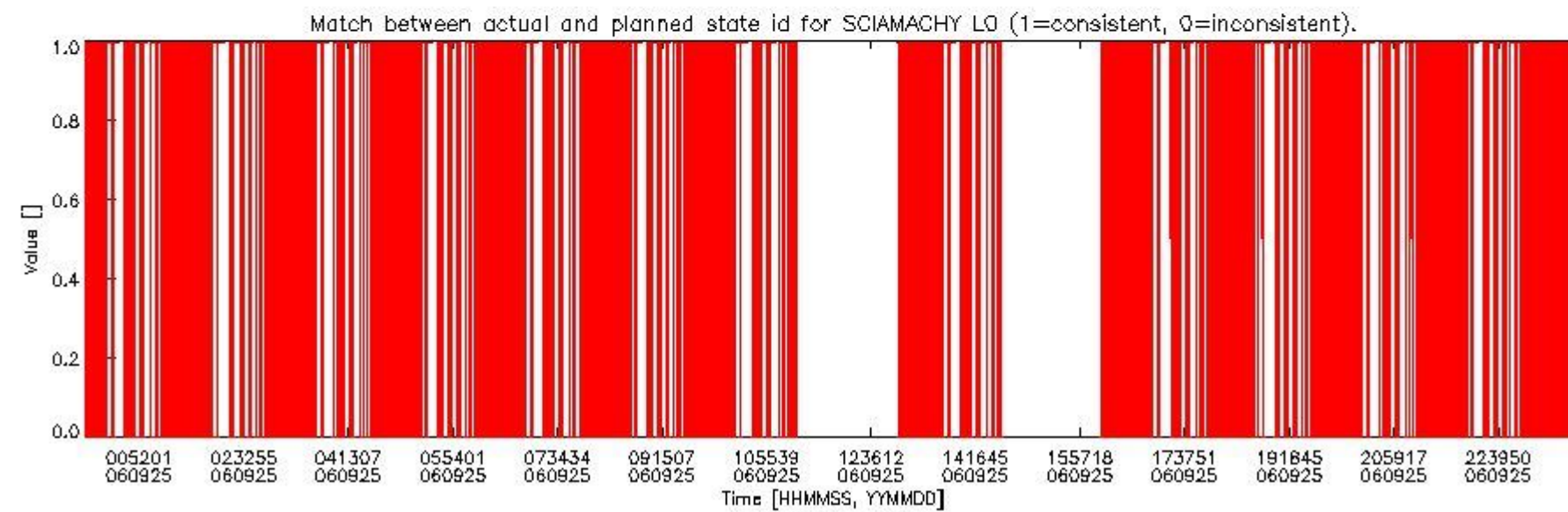
sciamachy_daily_report_level0_PFHS_5_37_N_20060925_5.PNG
