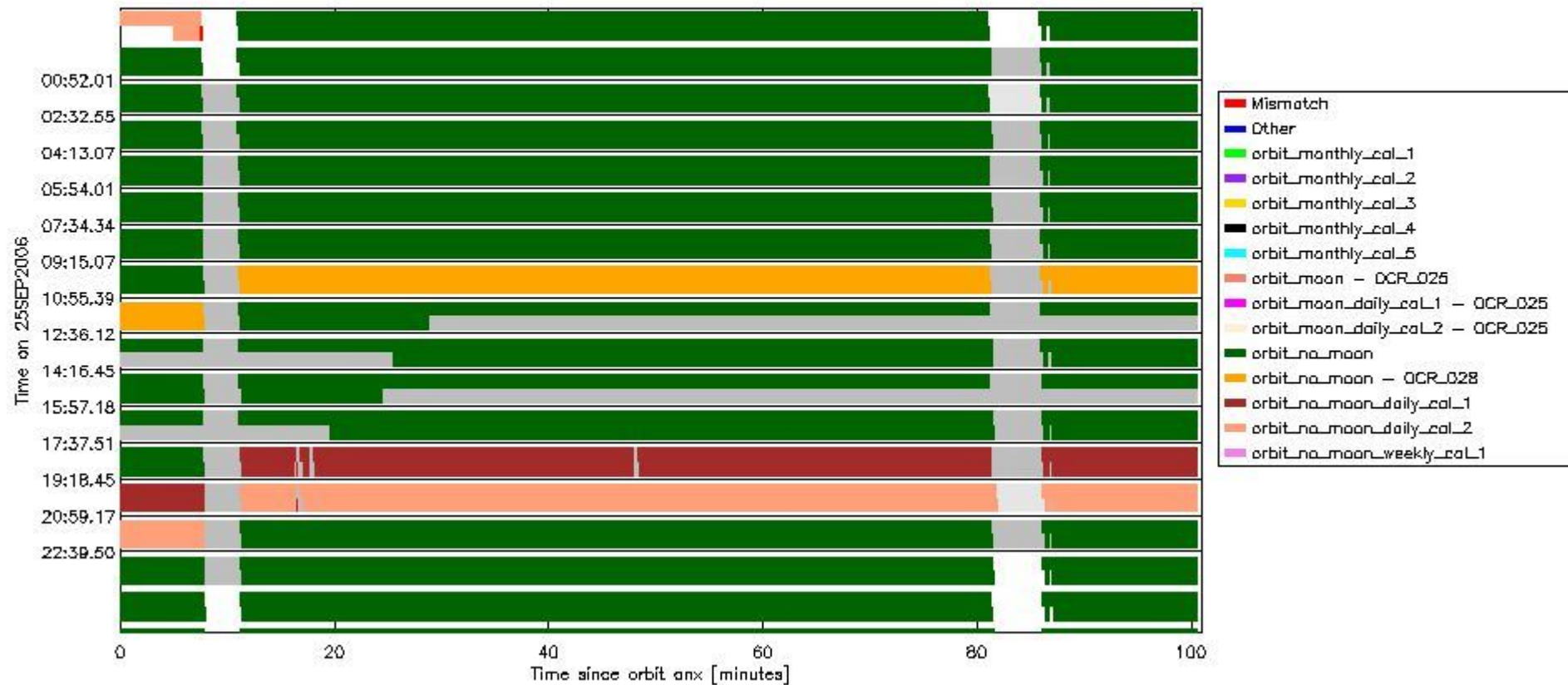
sciamachy_daily_report_level0_PFH5_5_37_N_20060925_6.PNG
