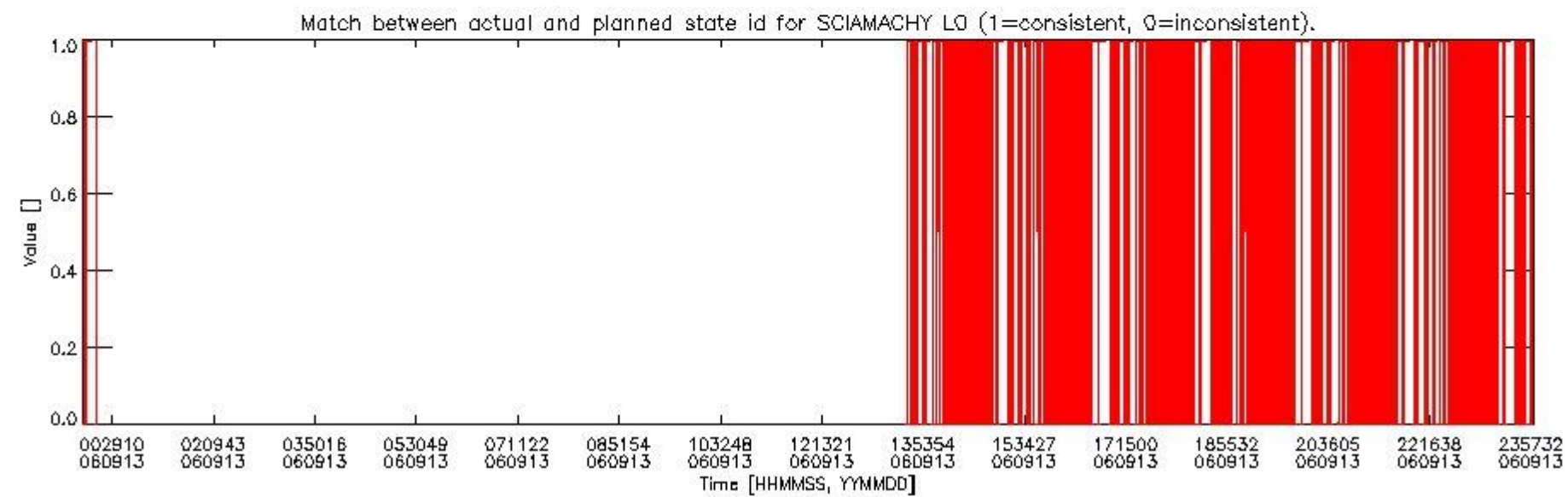
sciamachy_daily_report_level0_PFHS_5_37_N_20060913_5.PNG
