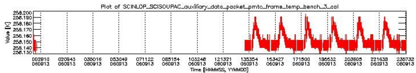
sciamachy_daily_report_level0_PFHS_5_37_N_20060913_2.PNG
