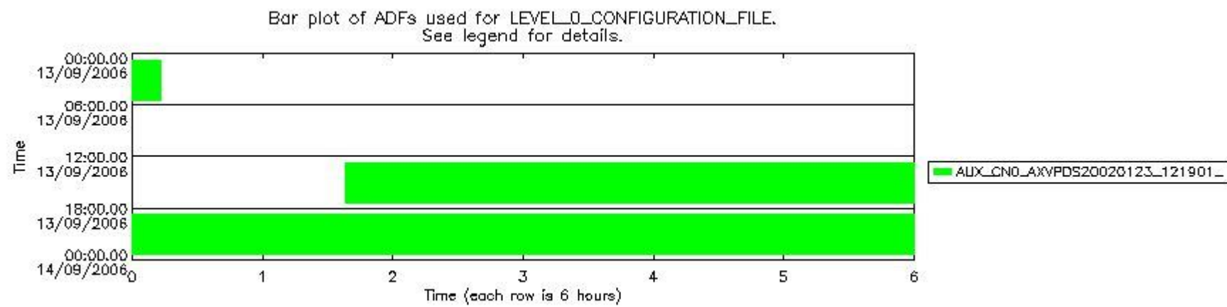
sciamachy_daily_report_level0_PFHS_5_37_N_20060913_7.PNG
