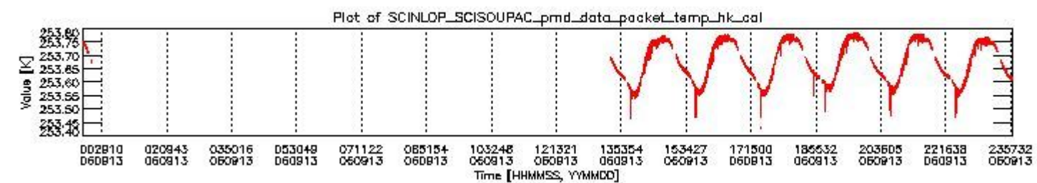
sciamachy_daily_report_level0_PFHS_5_37_N_20060913_3.PNG
