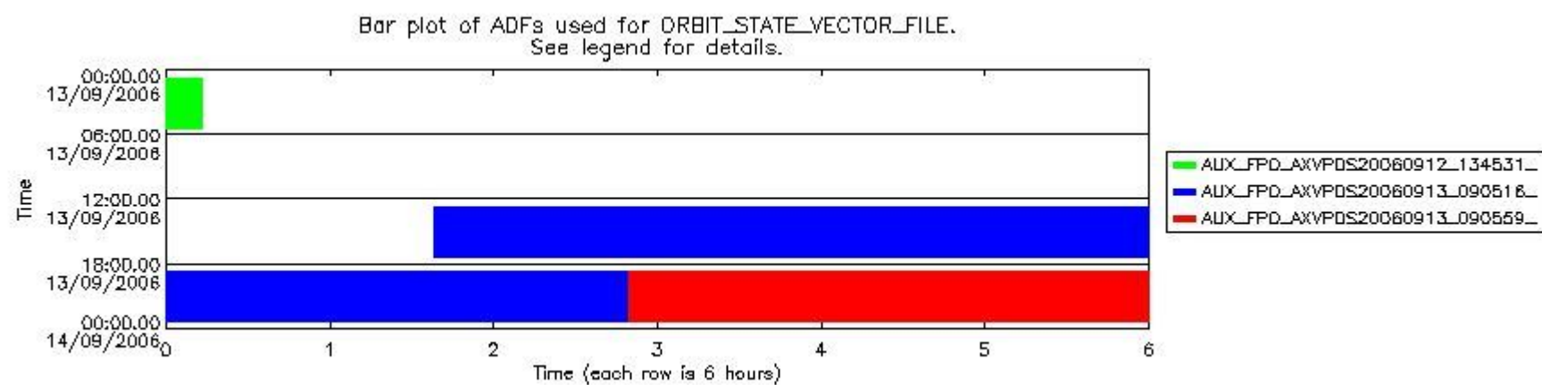
sciamachy_daily_report_level0_PFHS_5_37_N_20060913_8.PNG
