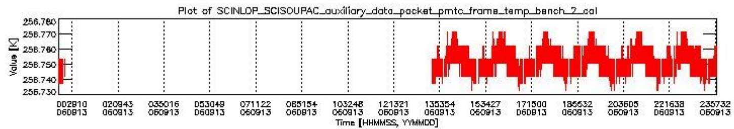
sciamachy_daily_report_level0_PFHS_5_37_N_20060913_1.PNG
