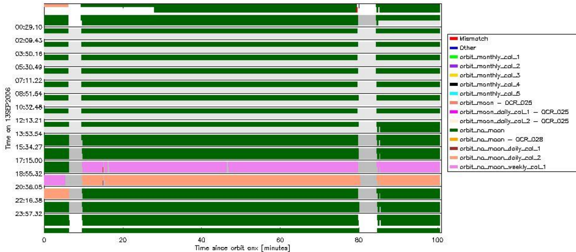
sciamachy_daily_report_level0_PPHS_5_37_N_20060913_6.PNG
