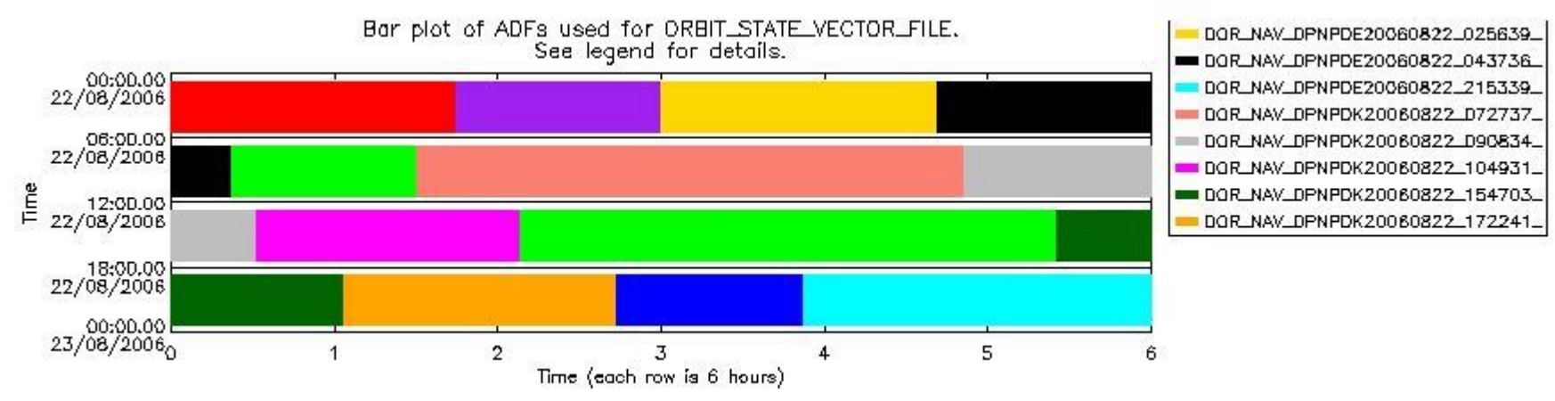
sciamachy_daily_report_level0_PFHS_5_37_N_20060822_8.PNG
