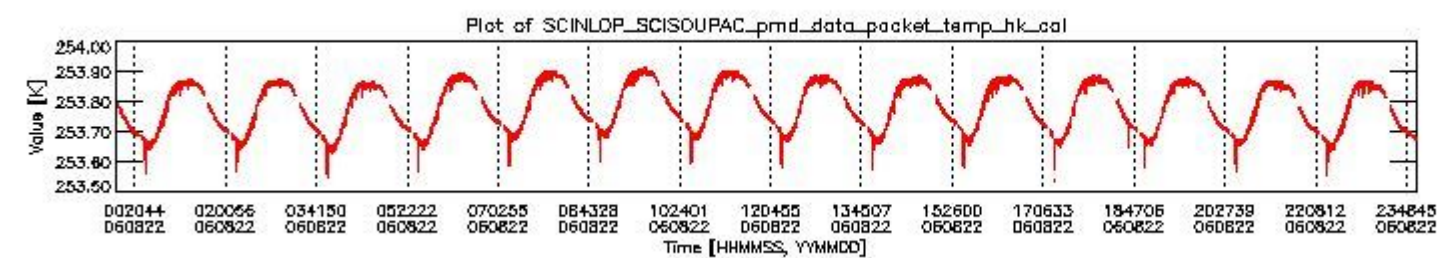
sciamachy_daily_report_level0_PFHS_5_37_N_20060822_3.PNG
