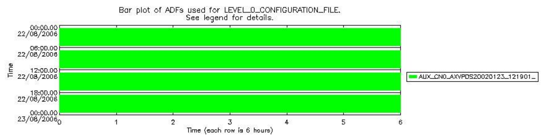
sciamachy_daily_report_level0_PFHS_5_37_N_20060822_7.PNG
