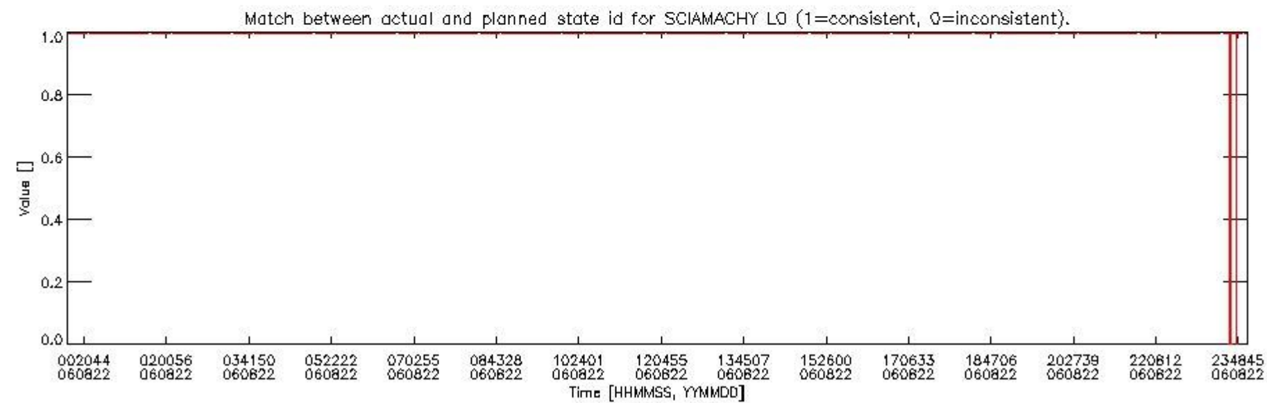
sciamachy_daily_report_level0_PFHS_5_37_N_20060822_5.PNG
