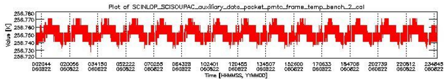
sciamachy_daily_report_level0_PFHS_5_37_N_20060822_1.PNG
