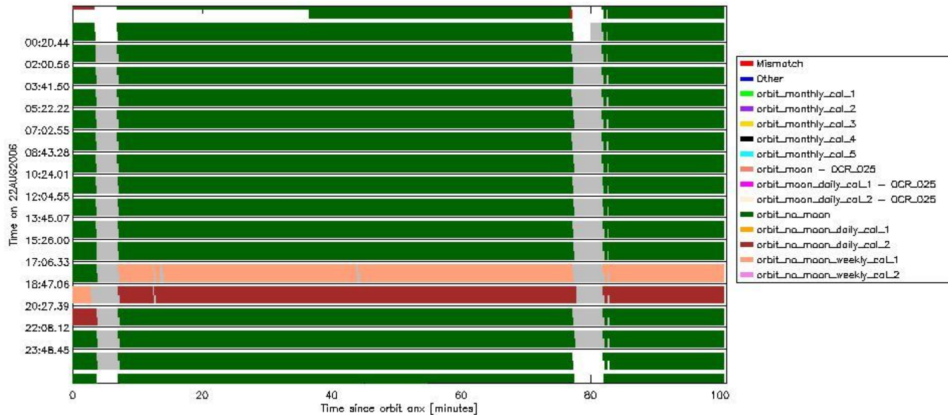
sciamachy_daily_report_level0_PFHS_5_37_N_20060822_6.PNG
