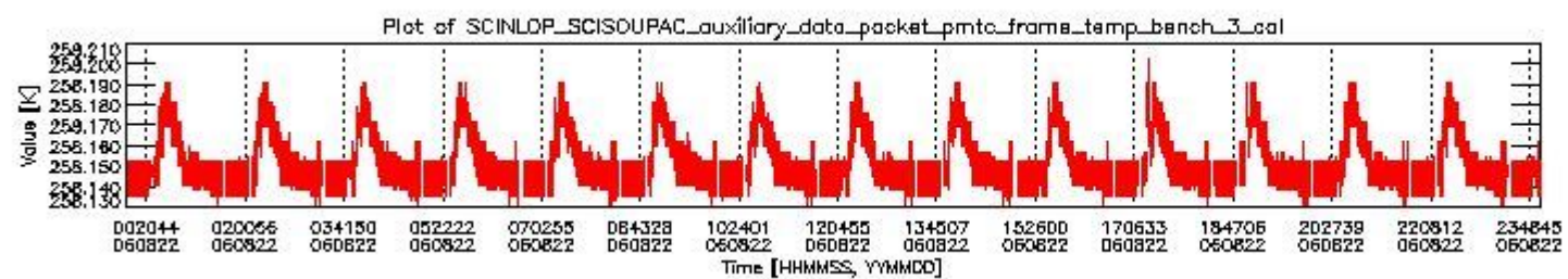
sciamachy_daily_report_level0_PFHS_5_37_N_20060822_2.PNG
