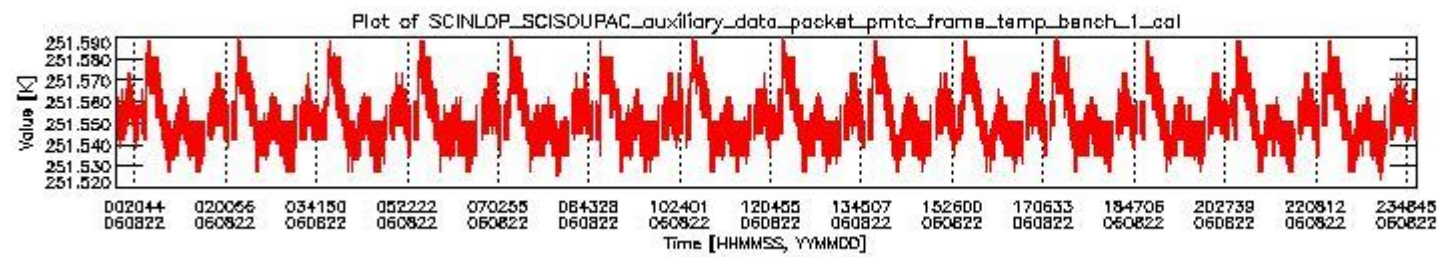
sciamachy_daily_report_level0_PFHS_5_37_N_20060822_0.PNG
