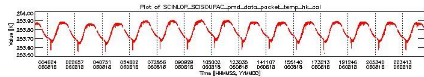
sciamachy_daily_report_level0_PFHS_5_37_N_20060818_3.PNG
