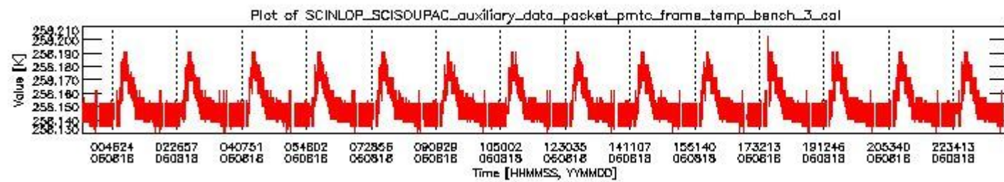
sciamachy_daily_report_level0_PFHS_5_37_N_20060818_2.PNG
