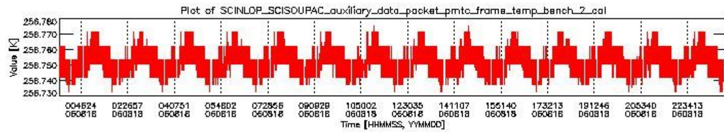
sciamachy_daily_report_level0_PFHS_5_37_N_20060818_1.PNG
