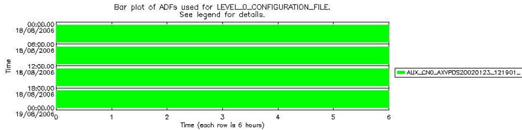
sciamachy_daily_report_level0_PFHS_5_37_N_20060818_7.PNG
