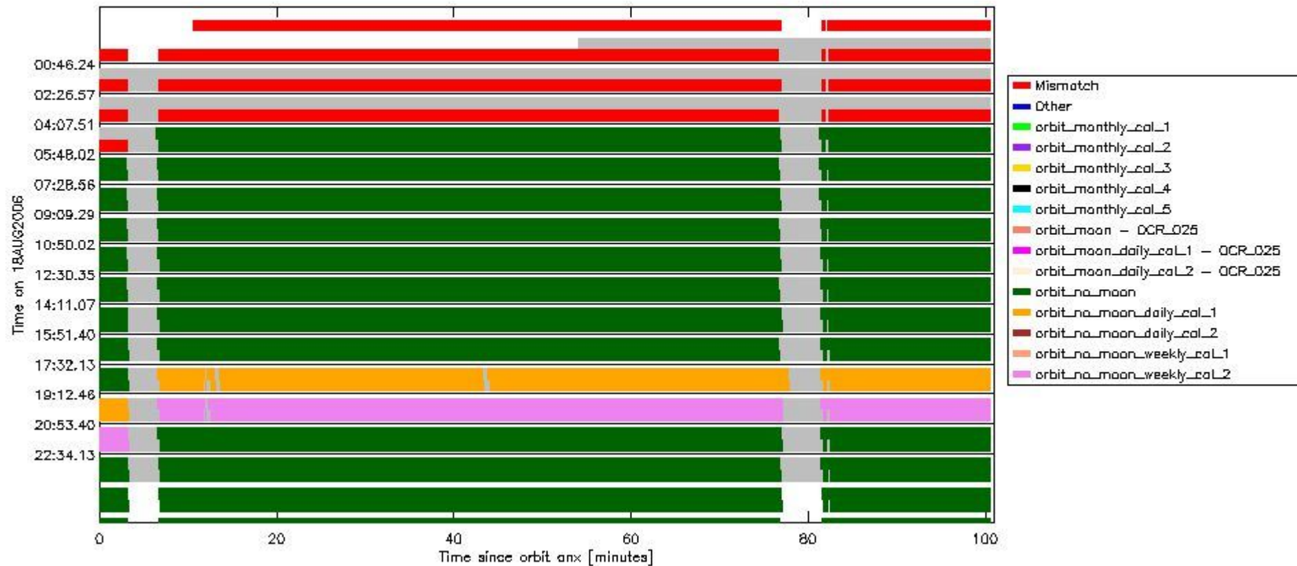
sciamachy_daily_report_level0_PFH5_5_37_N_20060818_6.PNG
