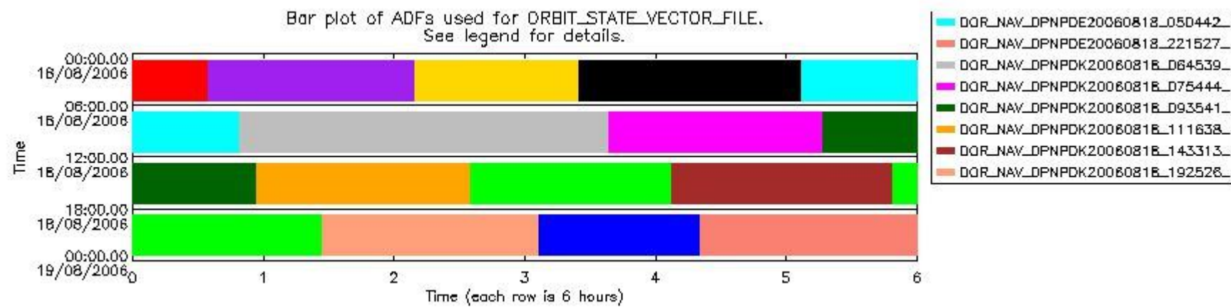
sciamachy_daily_report_level0_PFHS_5_37_N_20060818_8.PNG
