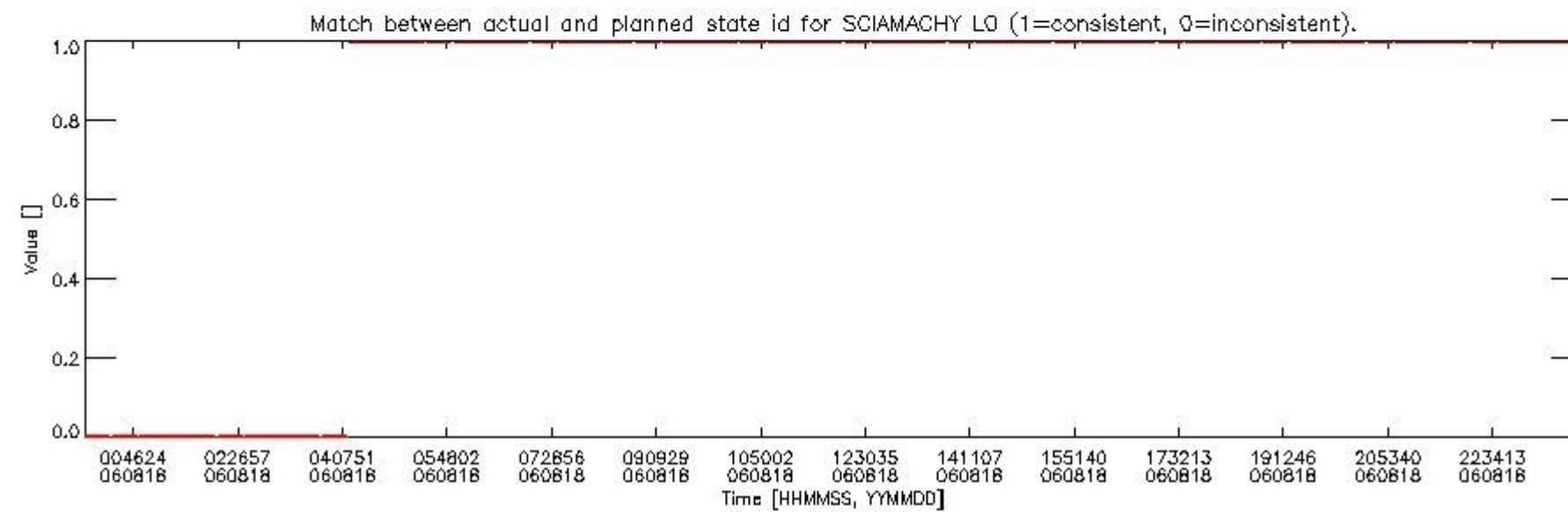
sciamachy_daily_report_level0_PFHS_5_37_N_20060818_5.PNG
