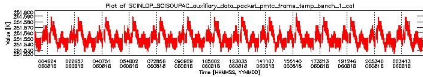
sciamachy_daily_report_level0_PFHS_5_37_N_20060818_0.PNG
