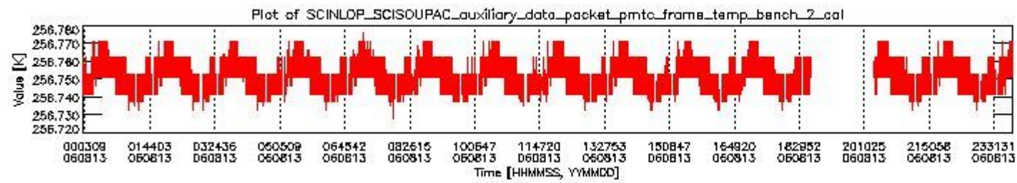
sciamachy_daily_report_level0_PFHS_5_37_N_20060813_1.PNG
