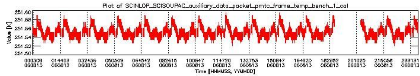
sciamachy_daily_report_level0_PFHS_5_37_N_20060813_0.PNG
