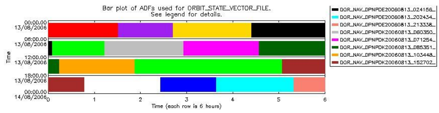
sciamachy_daily_report_level0_PFHS_5_37_N_20060813_8.PNG
