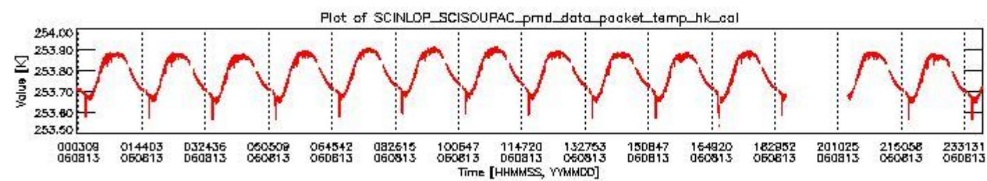
sciamachy_daily_report_level0_PFHS_5_37_N_20060813_3.PNG
