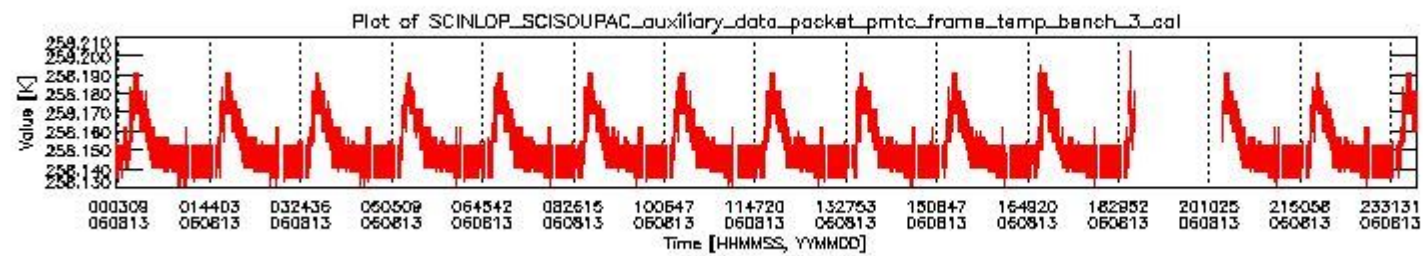
sciamachy_daily_report_level0_PFHS_5_37_N_20060813_2.PNG
