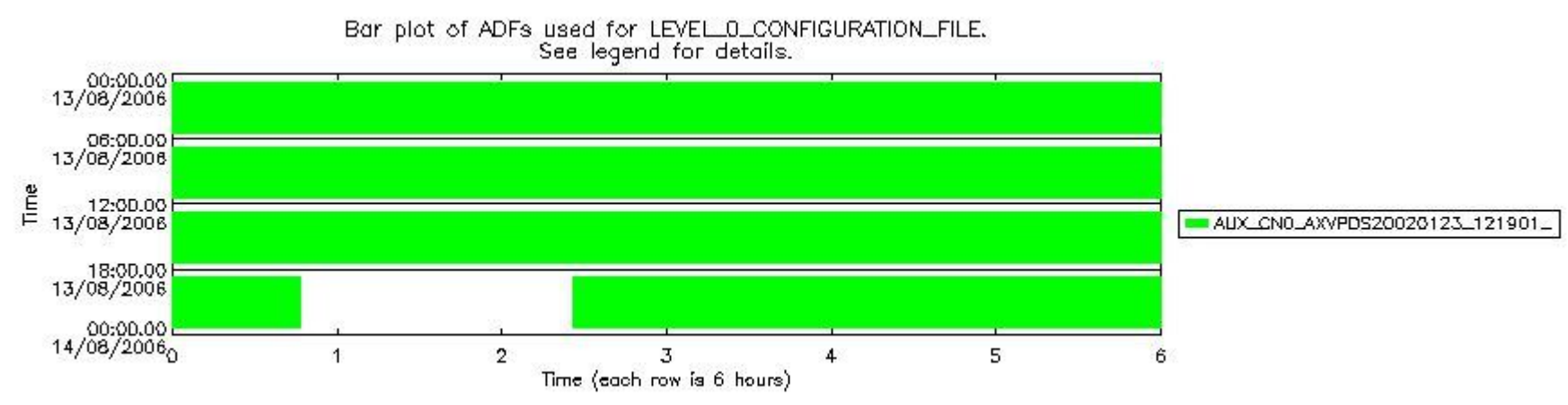
sciamachy_daily_report_level0_PFHS_5_37_N_20060813_7.PNG
