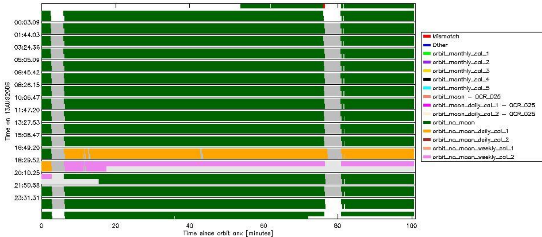
sciamachy_daily_report_level0_PPHS_5_37_N_20060813_6.PNG
