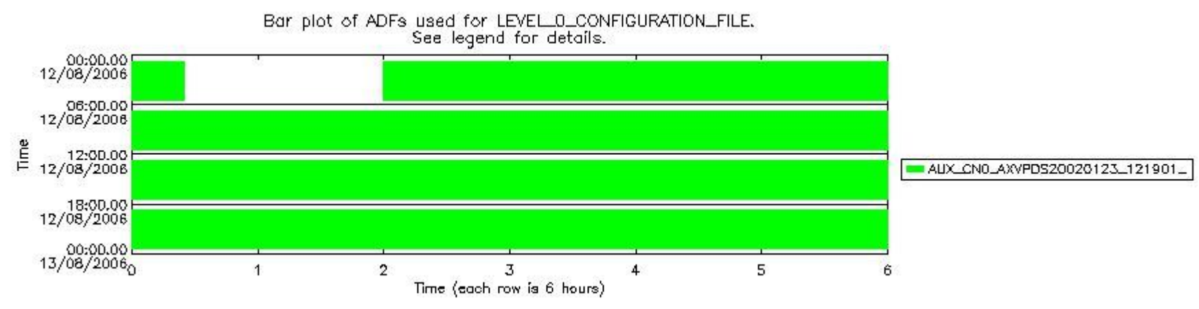
sciamachy_daily_report_level0_PFHS_5_37_N_20060812_7.PNG
