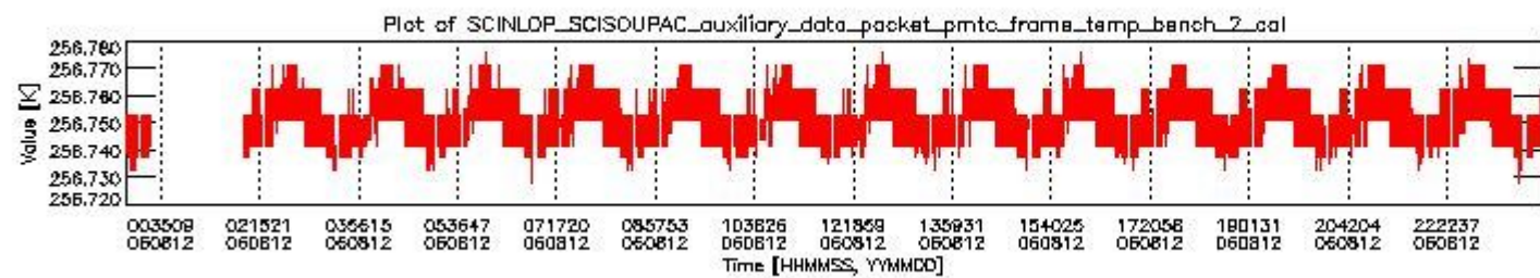
sciamachy_daily_report_level0_PFHS_5_37_N_20060812_1.PNG
