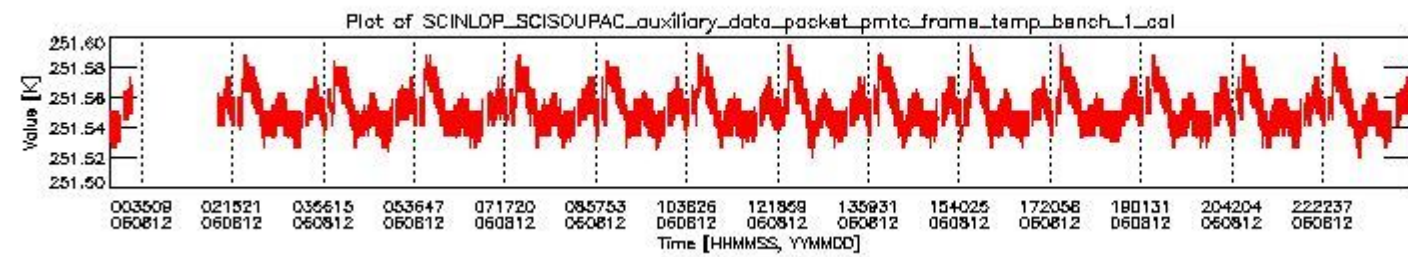
sciamachy_daily_report_level0_PFHS_5_37_N_20060812_0.PNG
