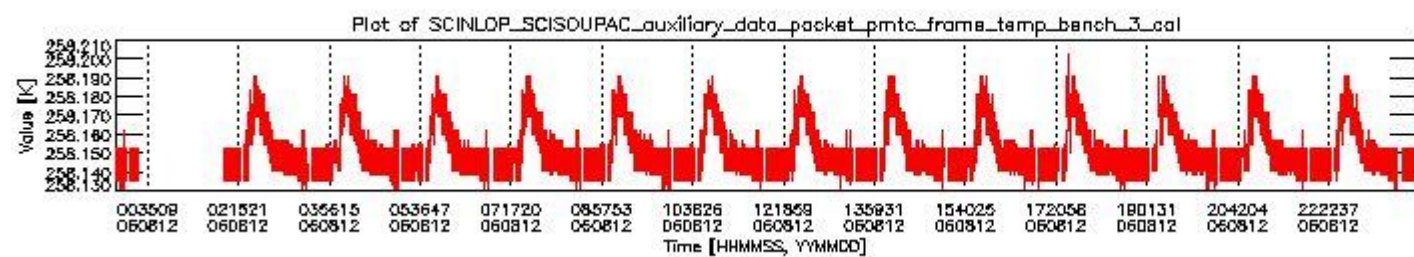
sciamachy_daily_report_level0_PFHS_5_37_N_20060812_2.PNG
