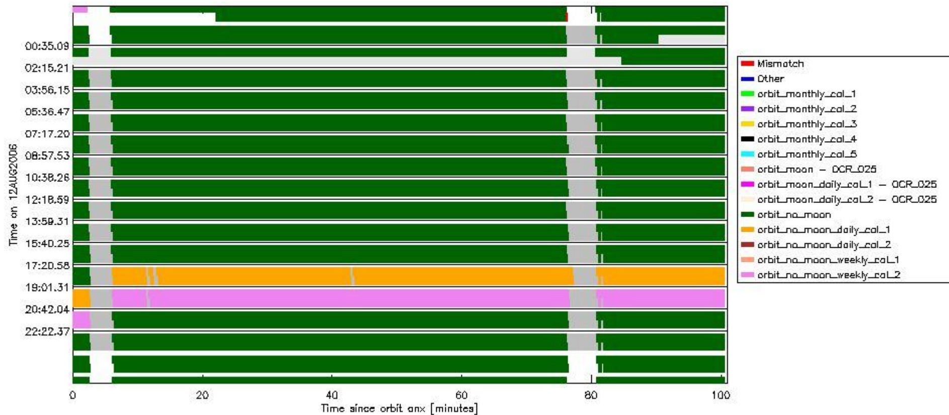
sciamachy_daily_report_level0_PPHS_5_37_N_20060812_6.PNG
