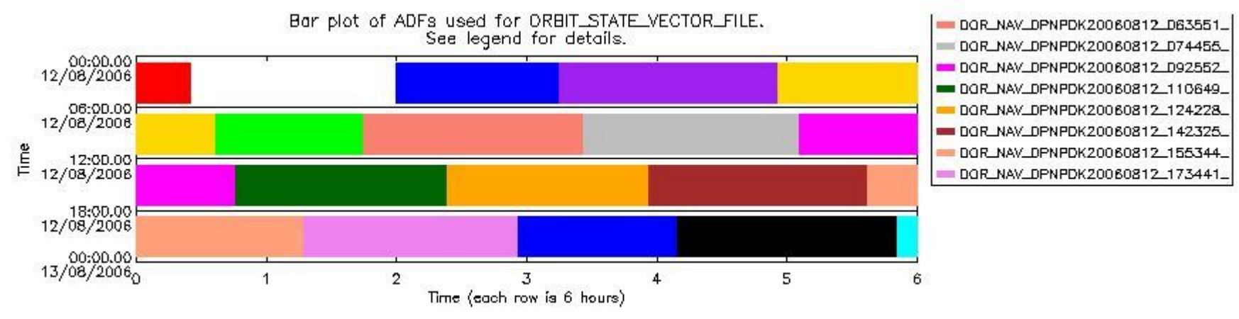
sciamachy_daily_report_level0_PFHS_5_37_N_20060812_8.PNG
