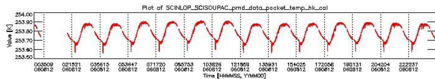
sciamachy_daily_report_level0_PFHS_5_37_N_20060812_3.PNG
