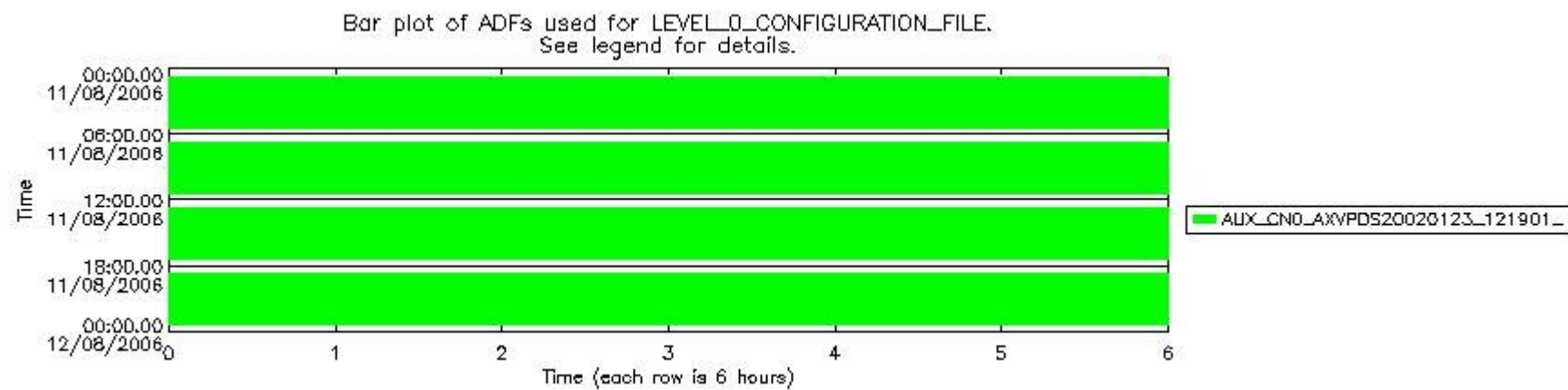
sciamachy_daily_report_level0_PFHS_5_37_N_20060811_7.PNG
