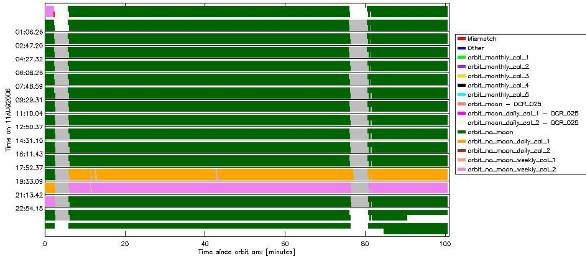
sciamachy_daily_report_level0_PPHS_5_37_N_20060811_6.PNG
