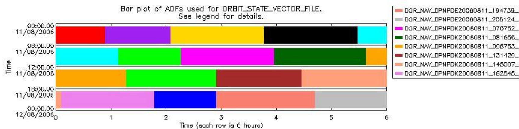
sciamachy_daily_report_level0_PFHS_5_37_N_20060811_8.PNG
