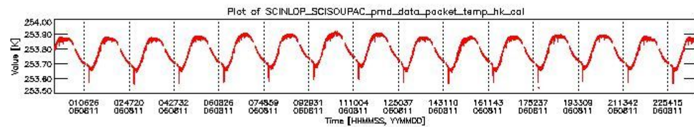
sciamachy_daily_report_level0_PFHS_5_37_N_20060811_3.PNG
