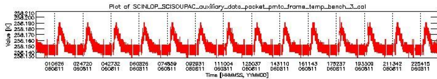
sciamachy_daily_report_level0_PFHS_5_37_N_20060811_2.PNG
