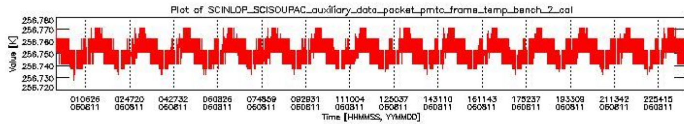
sciamachy_daily_report_level0_PFHS_5_37_N_20060811_1.PNG
