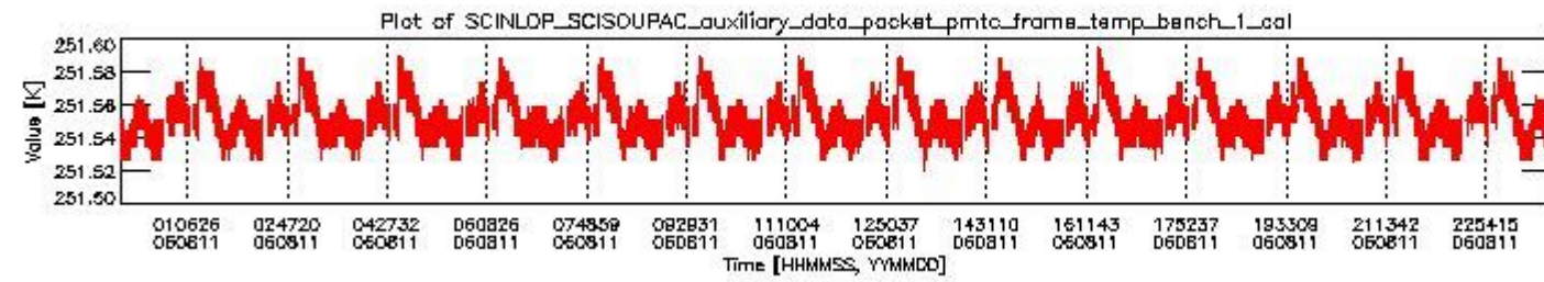
sciamachy_daily_report_level0_PFHS_5_37_N_20060811_0.PNG
