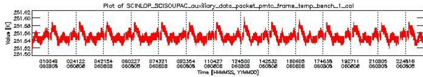
sciamachy_daily_report_level0_PFHS_5_37_N_20060808_0.PNG
