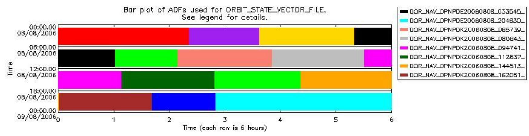
sciamachy_daily_report_level0_PFHS_5_37_N_20060808_8.PNG
