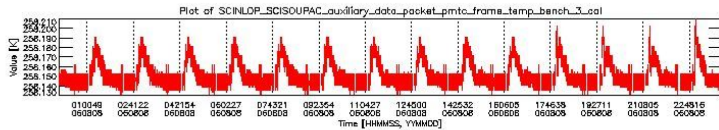
sciamachy_daily_report_level0_PFHS_5_37_N_20060808_2.PNG
