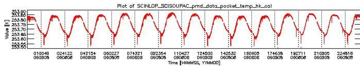
sciamachy_daily_report_level0_PFHS_5_37_N_20060808_3.PNG
