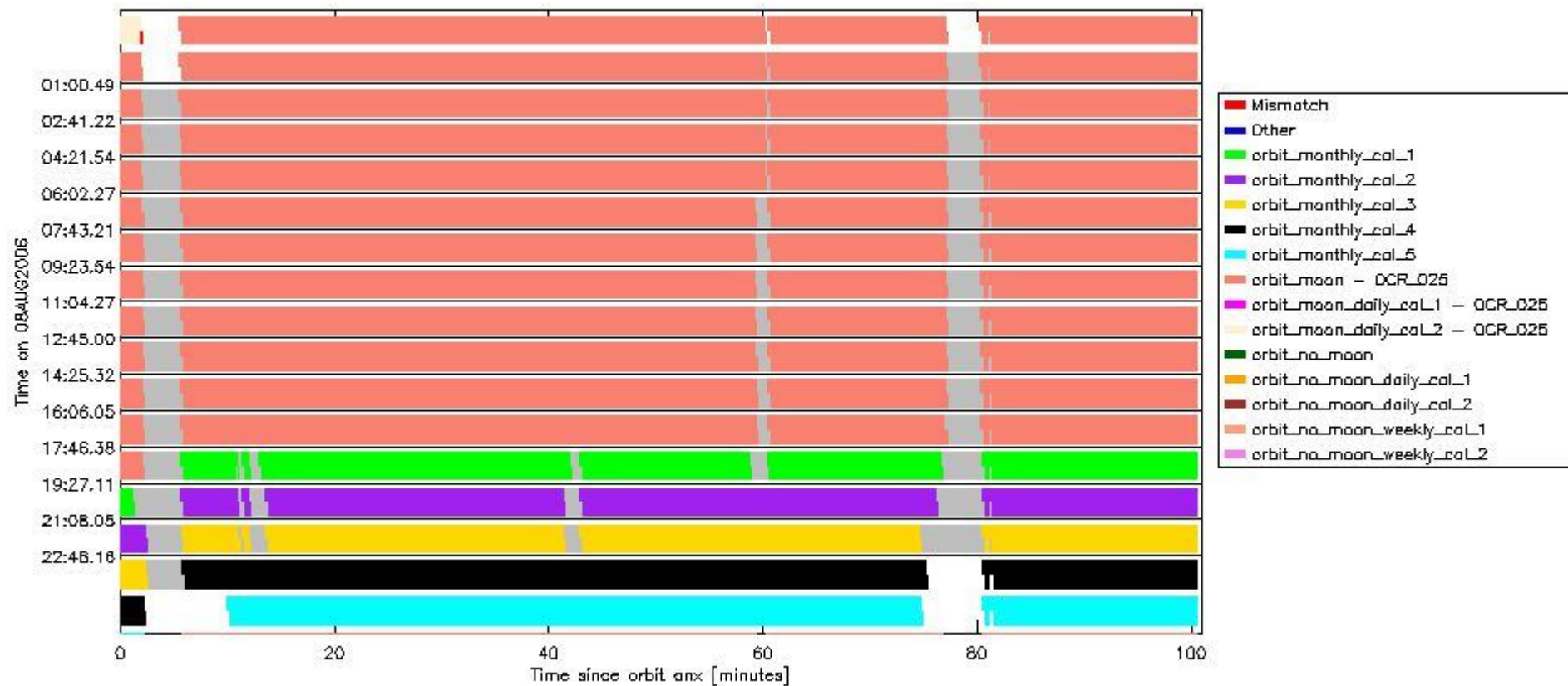
sciamachy_daily_report_level0_PFH5_5_37_N_20060808_6.PNG
