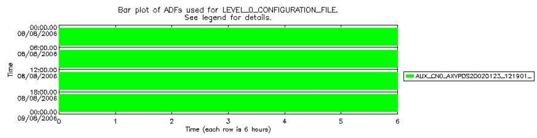
sciamachy_daily_report_level0_PFHS_5_37_N_20060808_7.PNG
