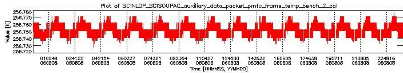
sciamachy_daily_report_level0_PFHS_5_37_N_20060808_1.PNG
