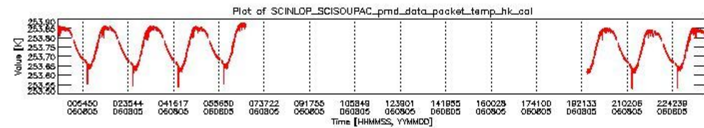
sciamachy_daily_report_level0_PFHS_5_37_N_20060805_3.PNG
