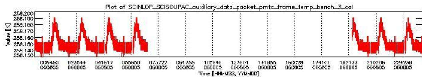
sciamachy_daily_report_level0_PFHS_5_37_N_20060805_2.PNG
