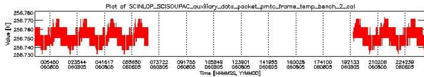
sciamachy_daily_report_level0_PFHS_5_37_N_20060805_1.PNG
