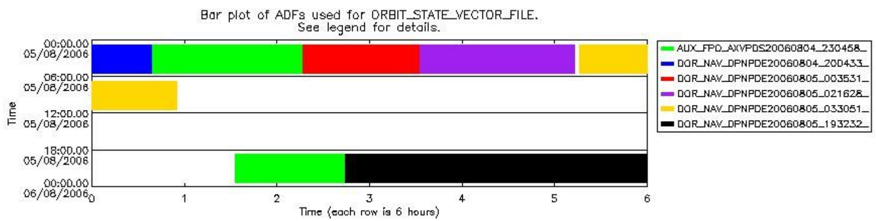
sciamachy_daily_report_level0_PFHS_5_37_N_20060805_7.PNG
