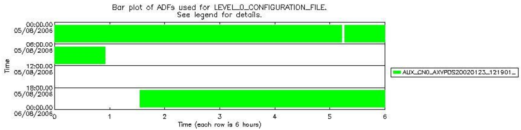
sciamachy_daily_report_level0_PFHS_5_37_N_20060805_6.PNG
