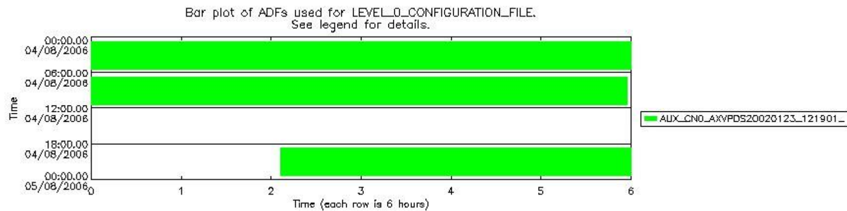
sciamachy_daily_report_level0_PFHS_5_37_N_20060804_6.PNG
