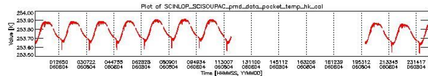
sciamachy_daily_report_level0_PFHS_5_37_N_20060804_3.PNG
