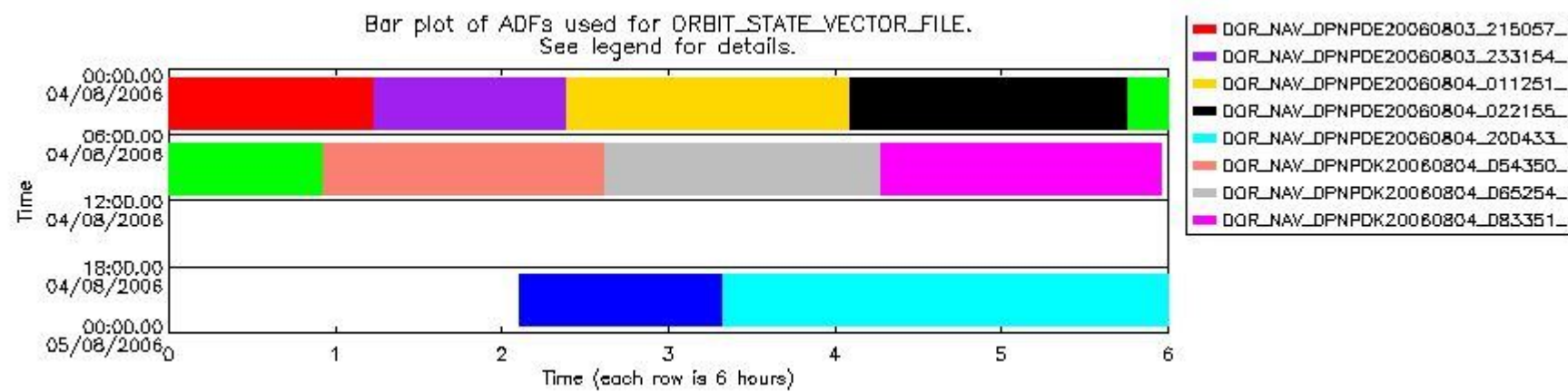
sciamachy_daily_report_level0_PFHS_5_37_N_20060804_7.PNG
