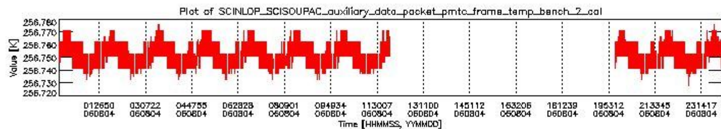
sciamachy_daily_report_level0_PFHS_5_37_N_20060804_1.PNG
