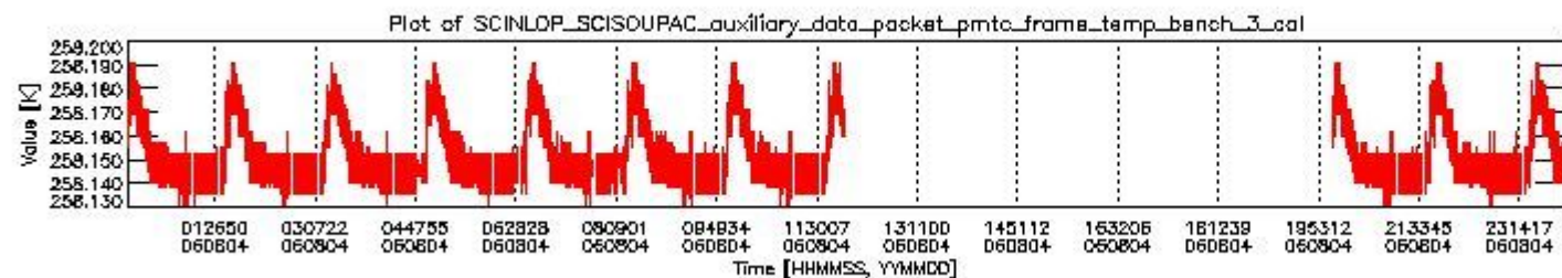
sciamachy_daily_report_level0_PFHS_5_37_N_20060804_2.PNG
