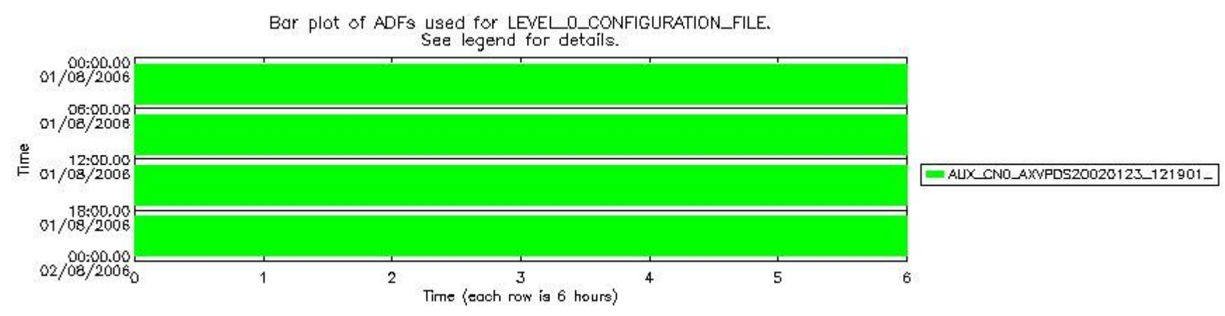
sciamachy_daily_report_level0_PFHS_5_37_N_20060801_7.PNG
