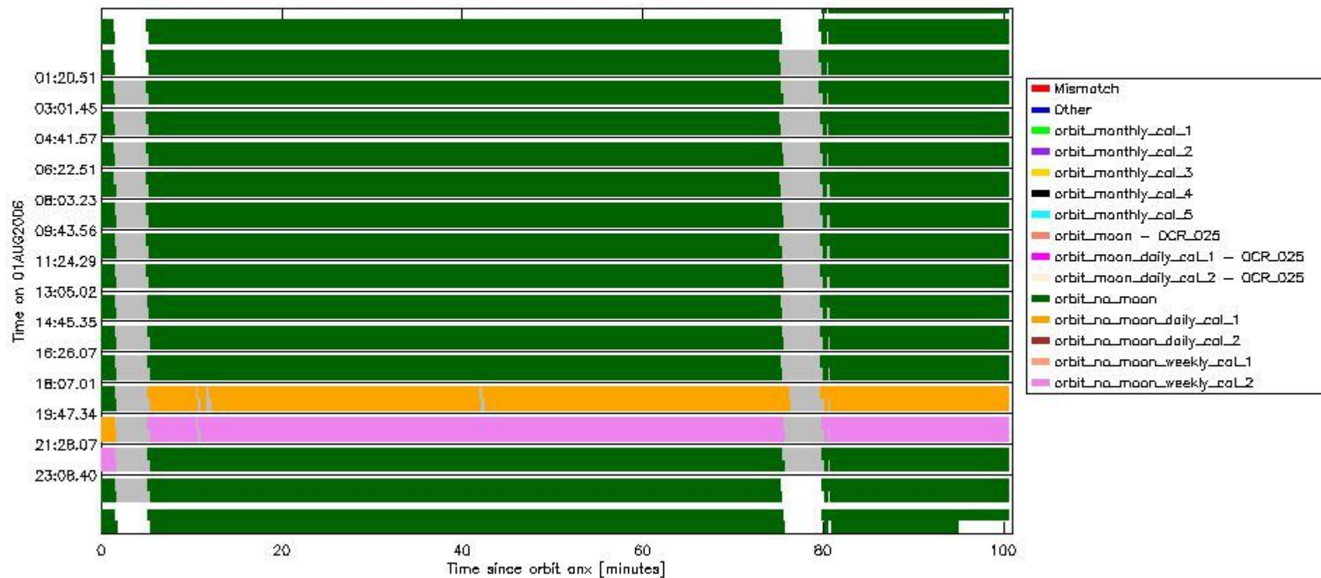
sciamachy_daily_report_level0_PPHS_5_37_N_20060801_6.PNG
