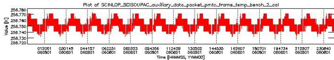
sciamachy_daily_report_level0_PFHS_5_37_N_20060801_1.PNG
