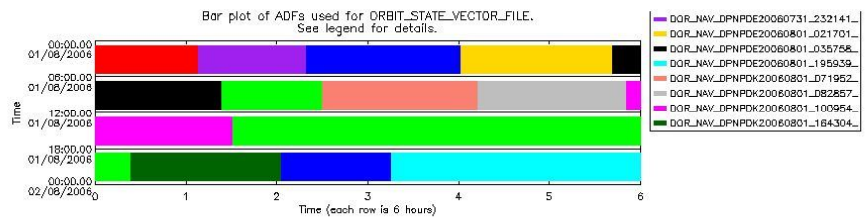
sciamachy_daily_report_level0_PFHS_5_37_N_20060801_8.PNG
