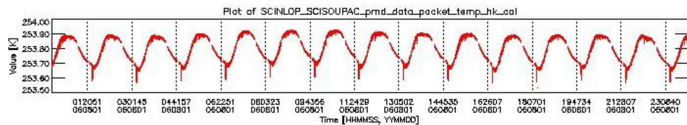
sciamachy_daily_report_level0_PFHS_5_37_N_20060801_3.PNG
