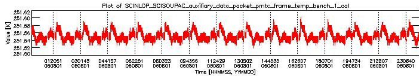
sciamachy_daily_report_level0_PFHS_5_37_N_20060801_0.PNG
