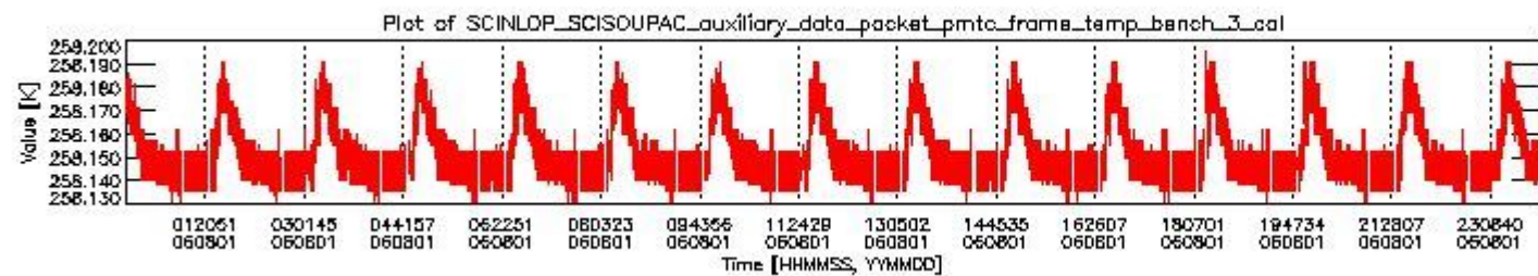
sciamachy_daily_report_level0_PFHS_5_37_N_20060801_2.PNG
