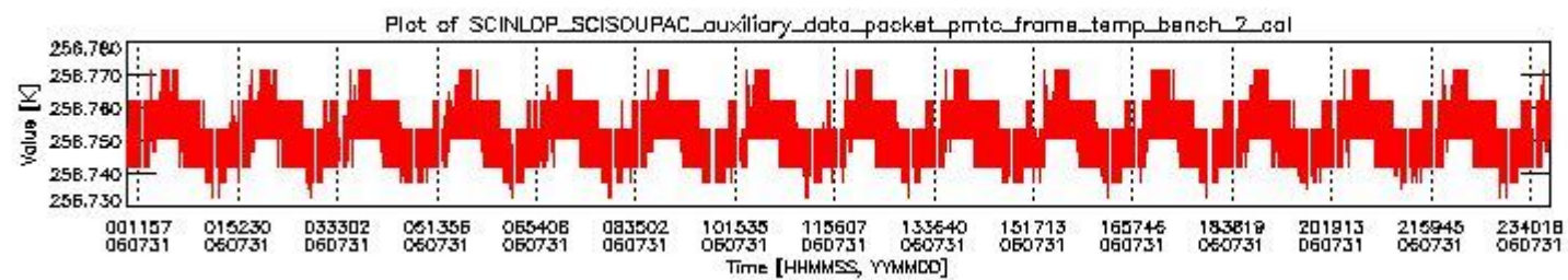
sciamachy_daily_report_level0_PFHS_5_37_N_20060731_1.PNG
