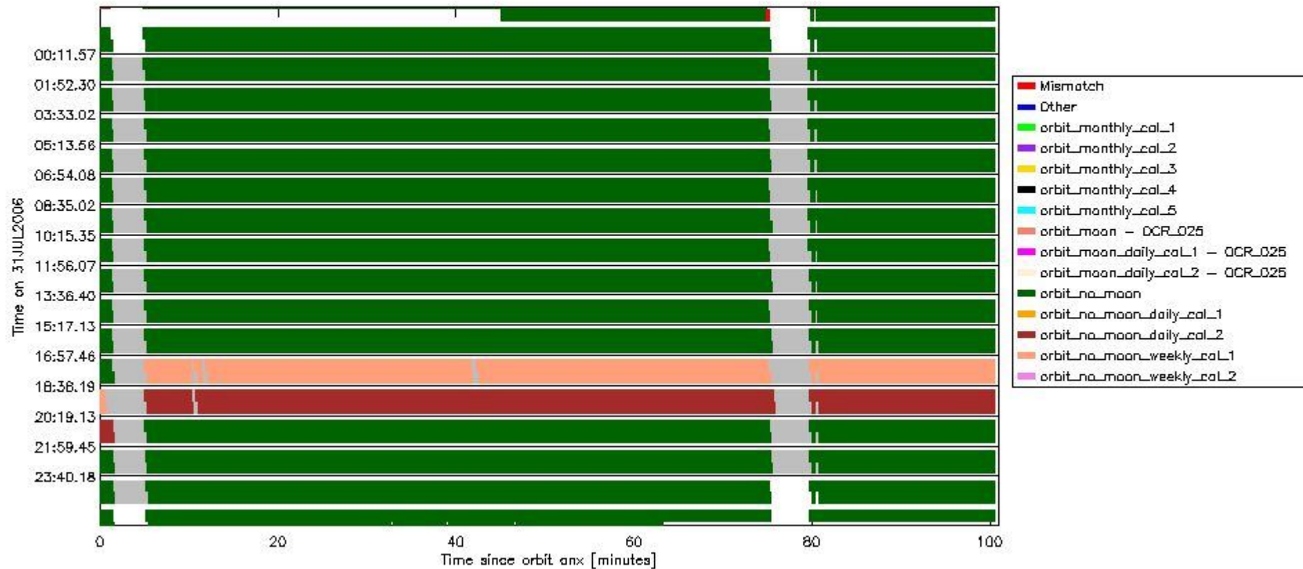
sciamachy_daily_report_level0_PFH5_5_37_N_20060731_6.PNG
