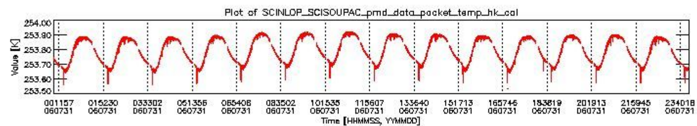
sciamachy_daily_report_level0_PFHS_5_37_N_20060731_3.PNG
