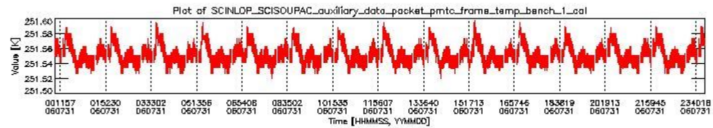
sciamachy_daily_report_level0_PFHS_5_37_N_20060731_0.PNG
