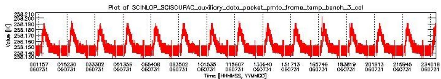
sciamachy_daily_report_level0_PFHS_5_37_N_20060731_2.PNG
