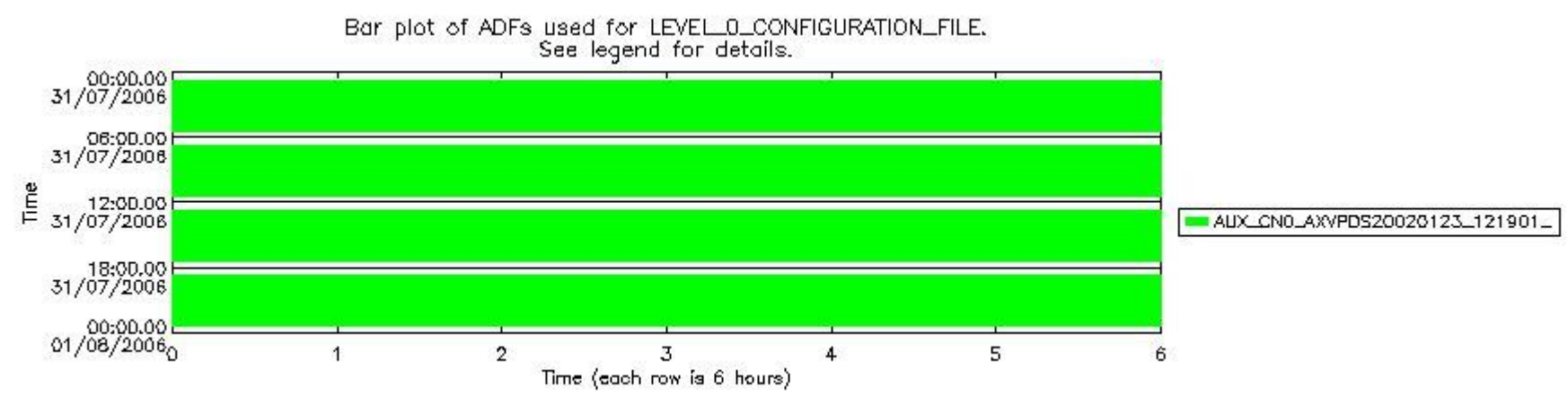
sciamachy_daily_report_level0_PFHS_5_37_N_20060731_7.PNG
