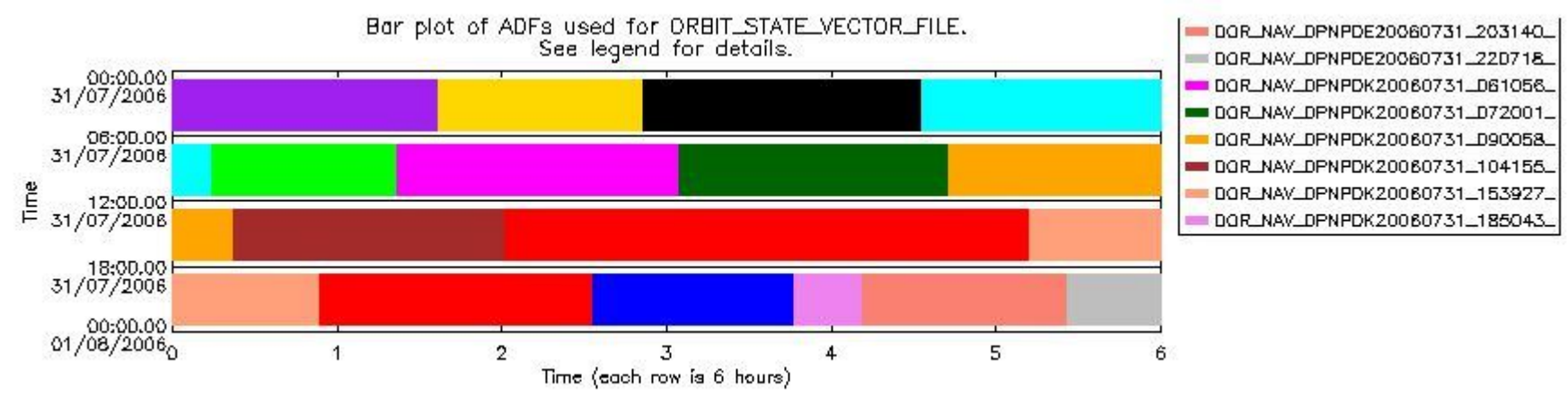
sciamachy_daily_report_level0_PFHS_5_37_N_20060731_8.PNG
