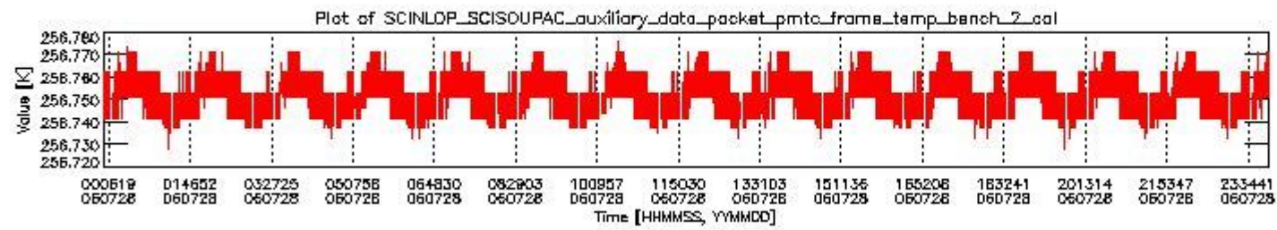
sciamachy_daily_report_level0_PFHS_5_37_N_20060728_1.PNG
