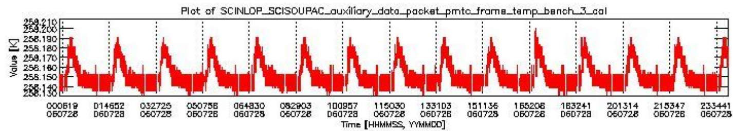
sciamachy_daily_report_level0_PFHS_5_37_N_20060728_2.PNG
