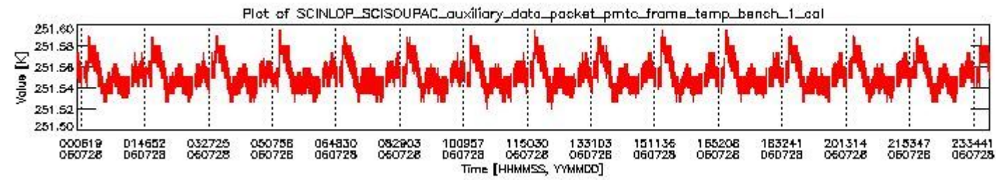
sciamachy_daily_report_level0_PFHS_5_37_N_20060728_0.PNG
