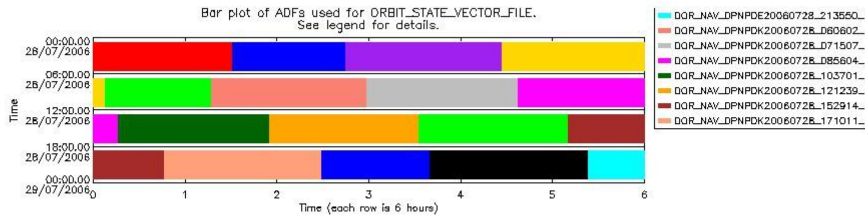
sciamachy_daily_report_level0_PFHS_5_37_N_20060728_8.PNG
