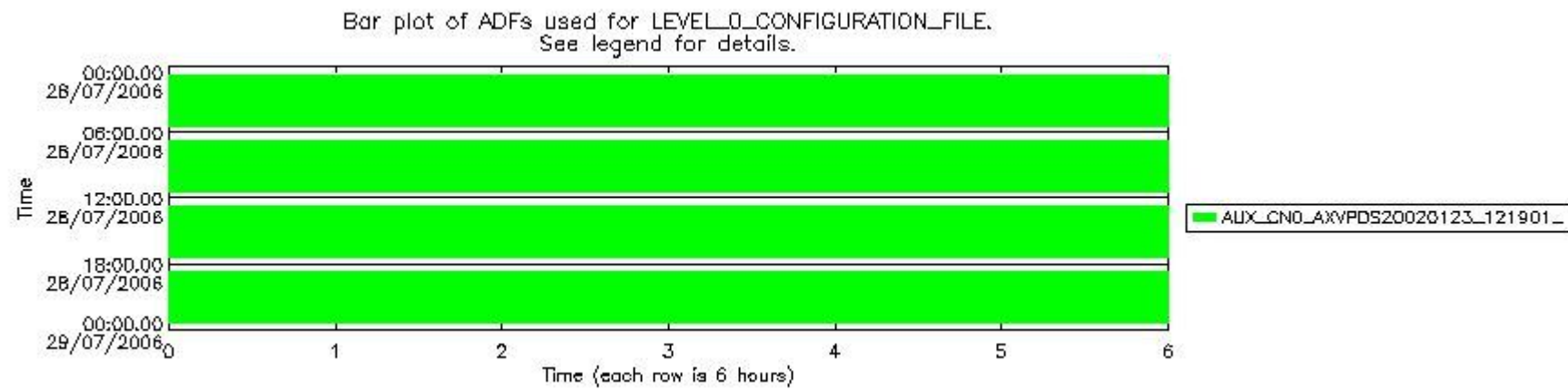
sciamachy_daily_report_level0_PFHS_5_37_N_20060728_7.PNG
