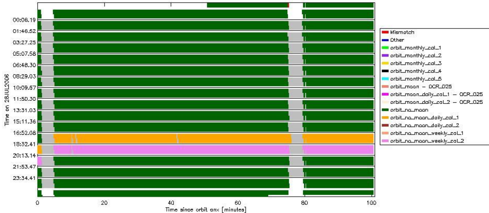
sciamachy_daily_report_level0_PFH5_5_37_N_20060728_6.PNG
