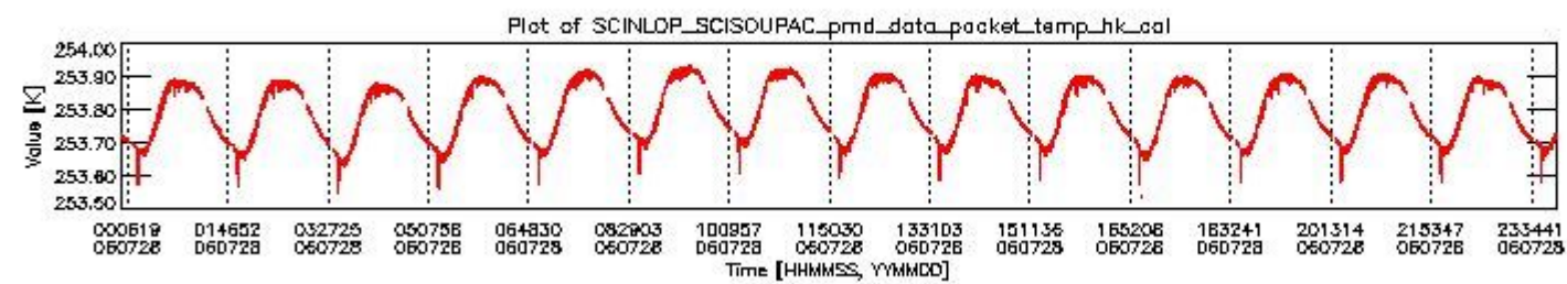
sciamachy_daily_report_level0_PFHS_5_37_N_20060728_3.PNG
