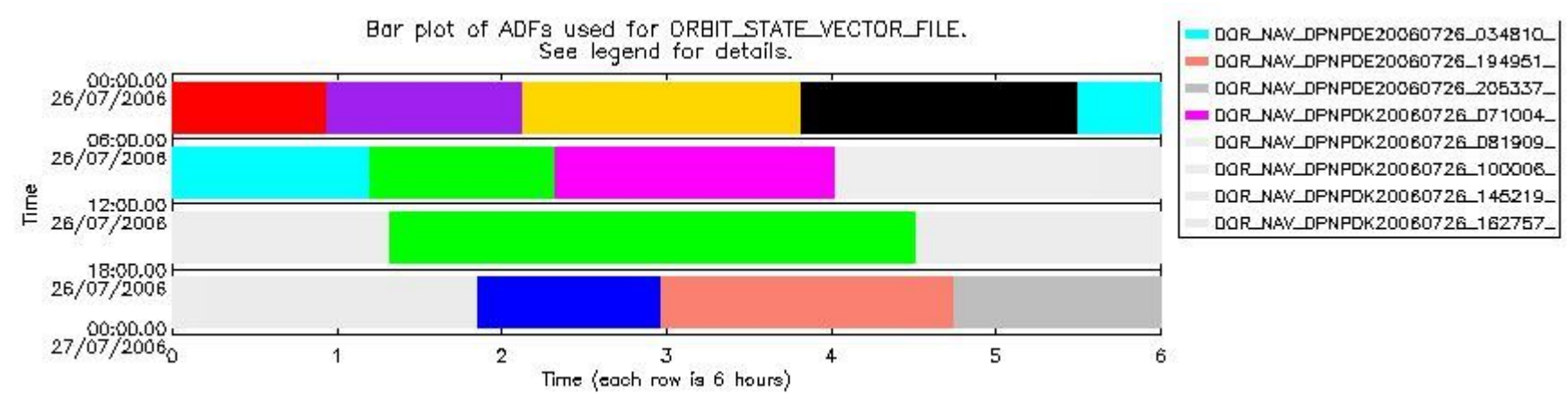
sciamachy_daily_report_level0_PFHS_5_37_N_20060726_6.PNG
