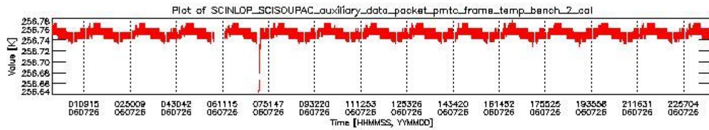
sciamachy_daily_report_level0_PFHS_5_37_N_20060726_1.PNG
