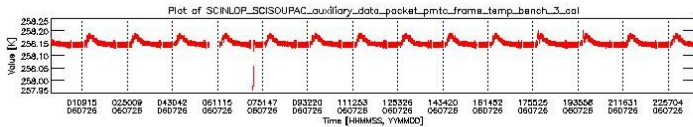
sciamachy_daily_report_level0_PFHS_5_37_N_20060726_2.PNG
