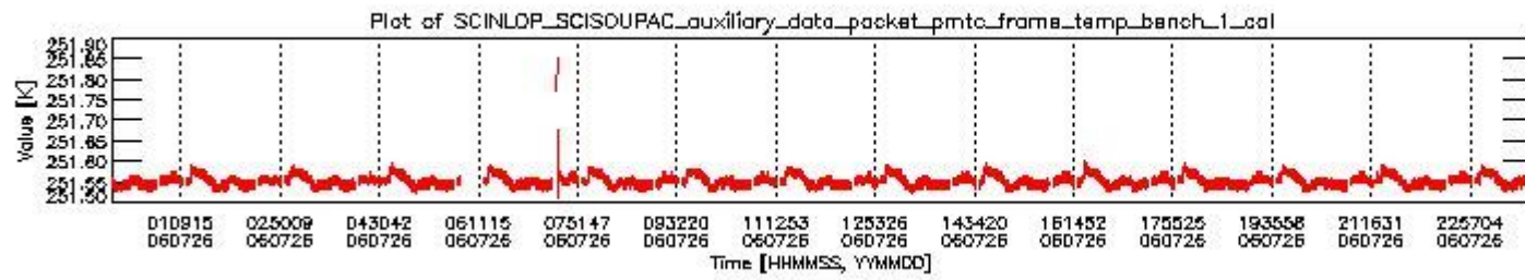
sciamachy_daily_report_level0_PFHS_5_37_N_20060726_0.PNG
