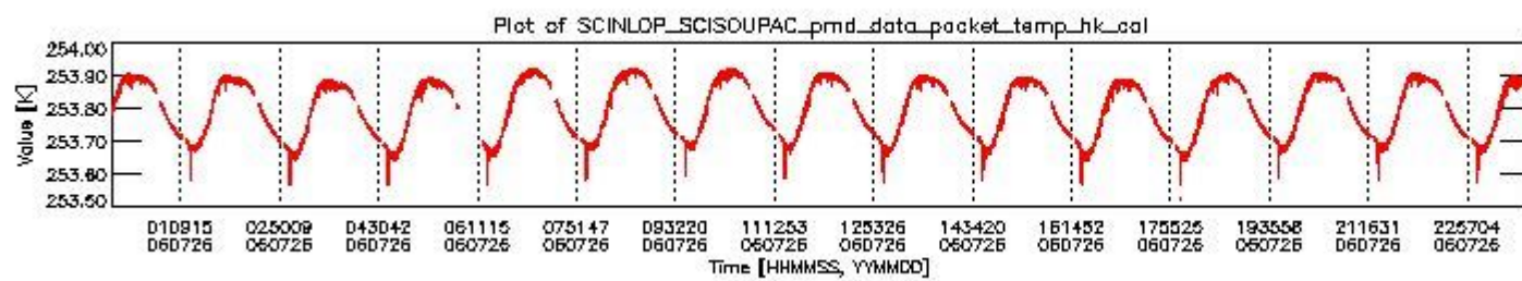
sciamachy_daily_report_level0_PFHS_5_37_N_20060726_3.PNG
