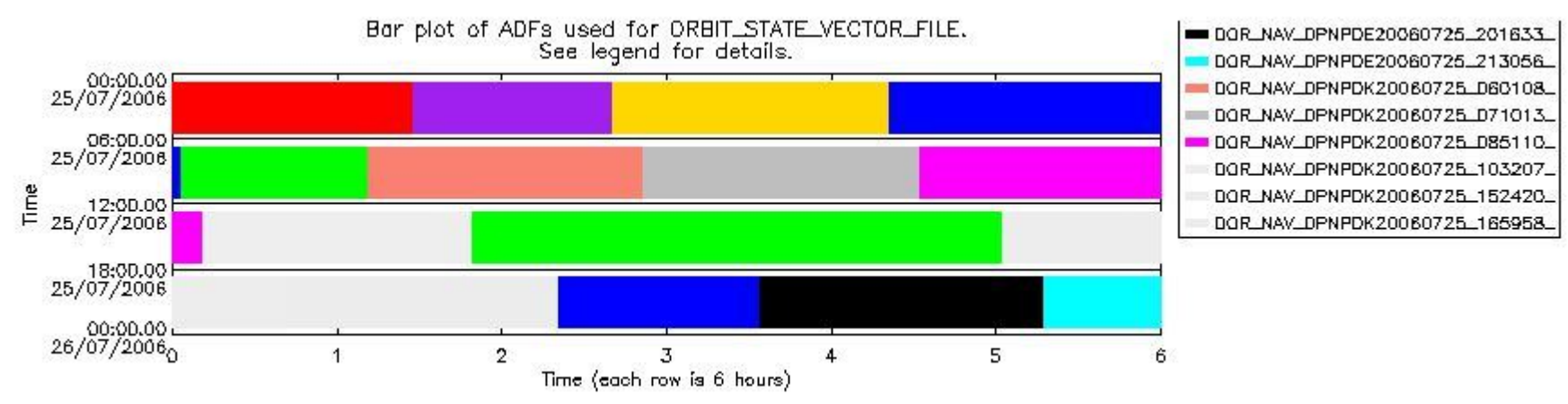
sciamachy_daily_report_level0_PFHS_5_37_N_20060725_6.PNG
