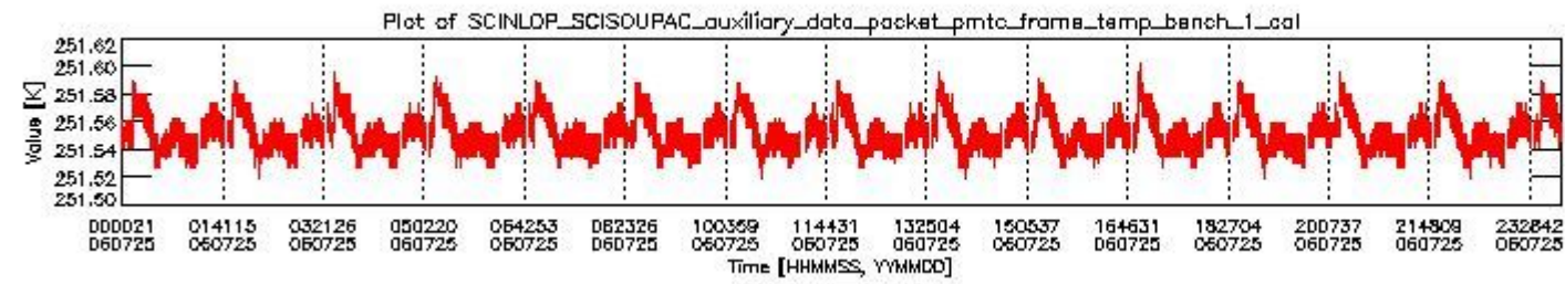
sciamachy_daily_report_level0_PFHS_5_37_N_20060725_0.PNG
