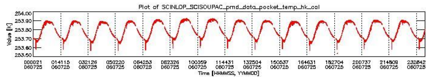
sciamachy_daily_report_level0_PFHS_5_37_N_20060725_3.PNG
