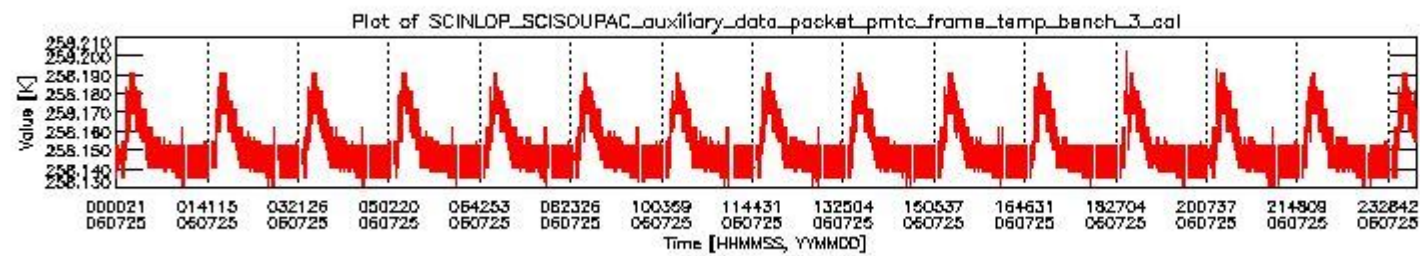
sciamachy_daily_report_level0_PFHS_5_37_N_20060725_2.PNG
