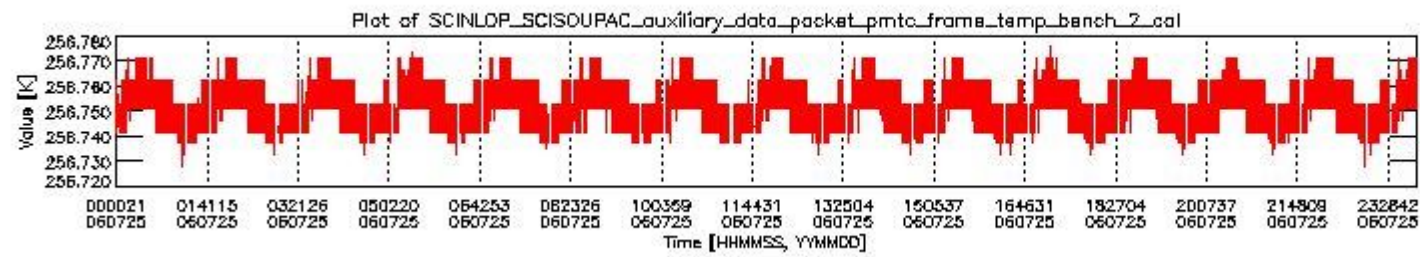
sciamachy_daily_report_level0_PFHS_5_37_N_20060725_1.PNG
