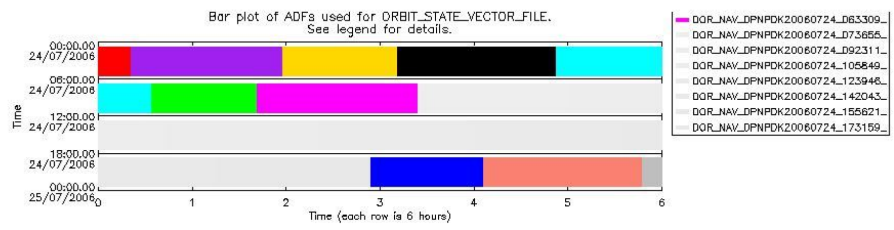
sciamachy_daily_report_level0_PFHS_5_37_N_20060724_6.PNG
