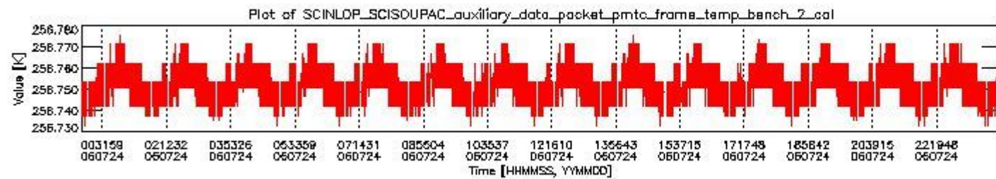
sciamachy_daily_report_level0_PFHS_5_37_N_20060724_1.PNG
