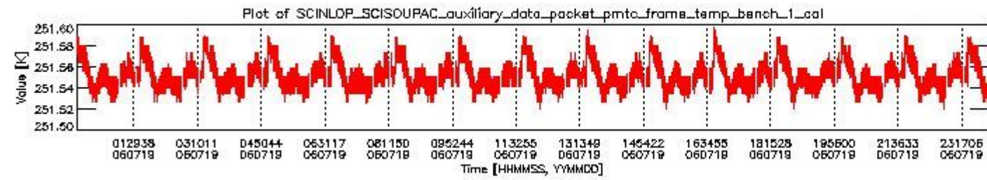
sciamachy_daily_report_level0_PPHS_5_37_N_20060719_0.PNG
