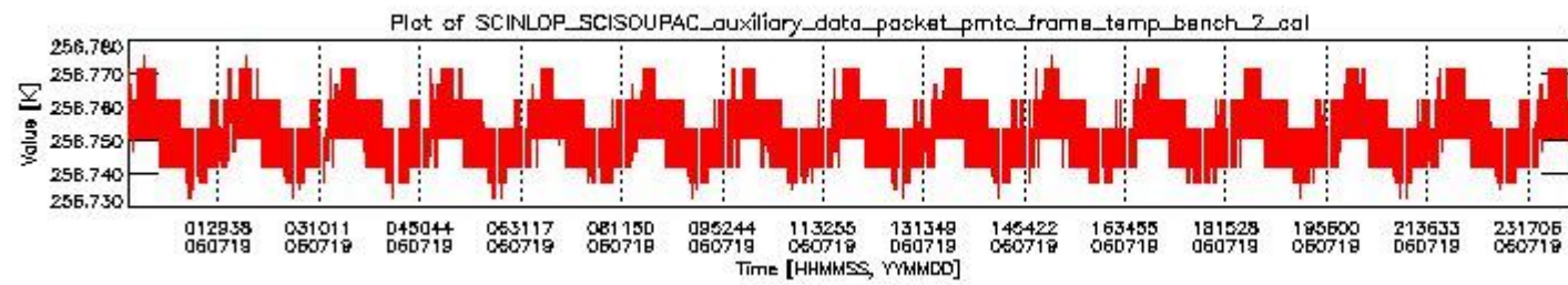
sciamachy_daily_report_level0_PPHS_5_37_N_20060719_1.PNG
