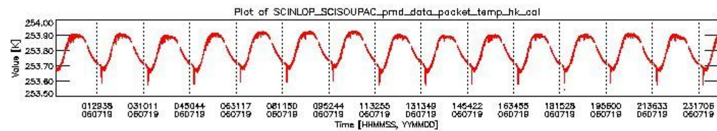
sciamachy_daily_report_level0_PPHS_5_37_N_20060719_3.PNG
