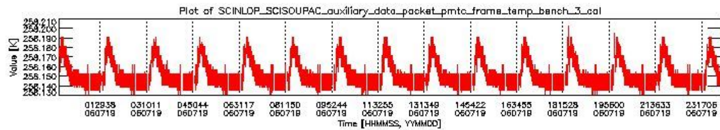
sciamachy_daily_report_level0_PPHS_5_37_N_20060719_2.PNG
