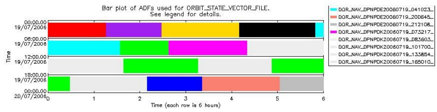
sciamachy_daily_report_level0_PFHS_5_37_N_20060719_6.PNG
