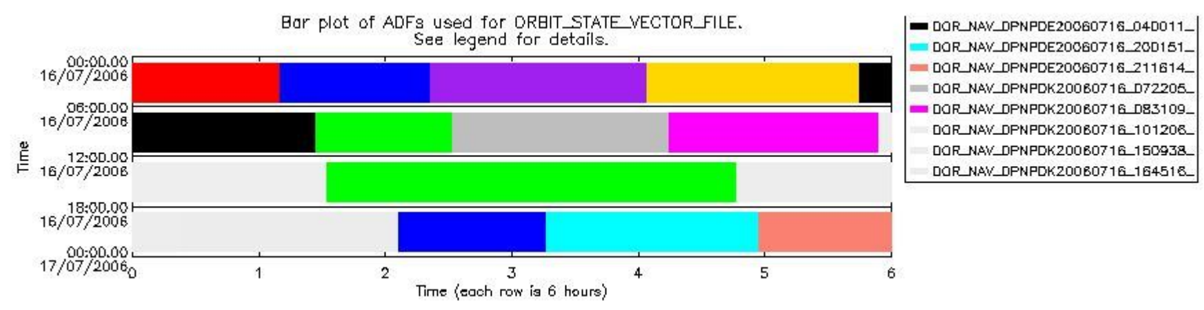
sciamachy_daily_report_level0_PFHS_5_37_N_20060716_6.PNG
