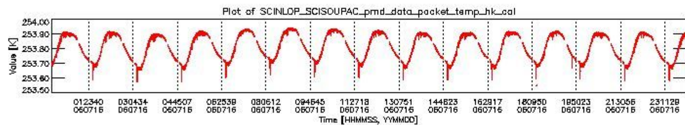
sciamachy_daily_report_level0_PFHS_5_37_N_20060716_3.PNG
