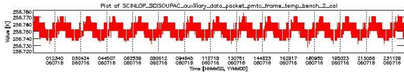
sciamachy_daily_report_level0_PFHS_5_37_N_20060716_1.PNG
