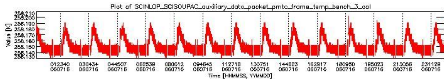
sciamachy_daily_report_level0_PFHS_5_37_N_20060716_2.PNG
