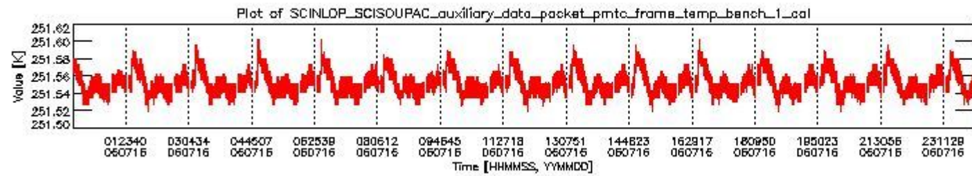
sciamachy_daily_report_level0_PFHS_5_37_N_20060716_0.PNG
