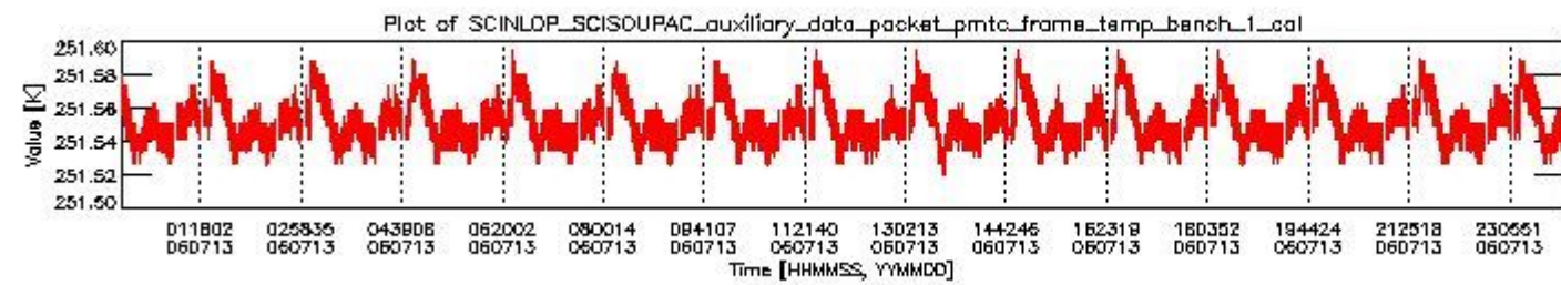
sciamachy_daily_report_level0_PFHS_5_37_N_20060713_0.PNG
