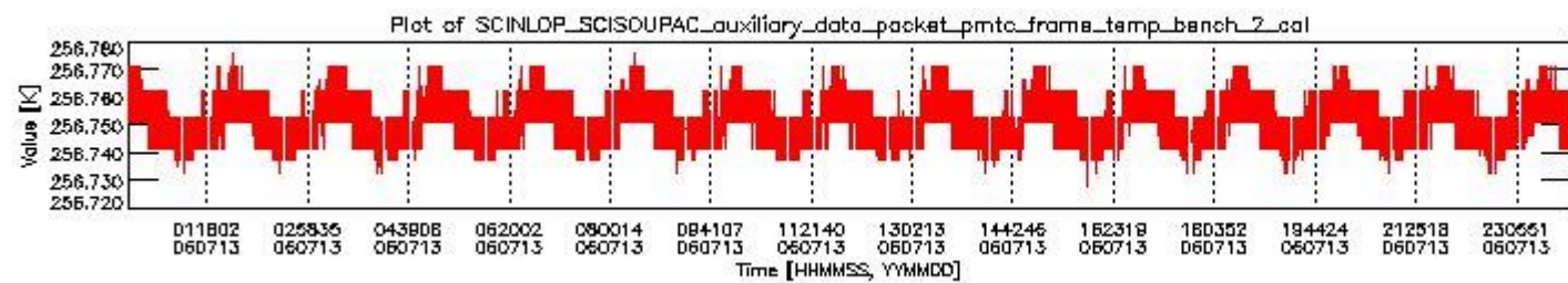
sciamachy_daily_report_level0_PFHS_5_37_N_20060713_1.PNG
