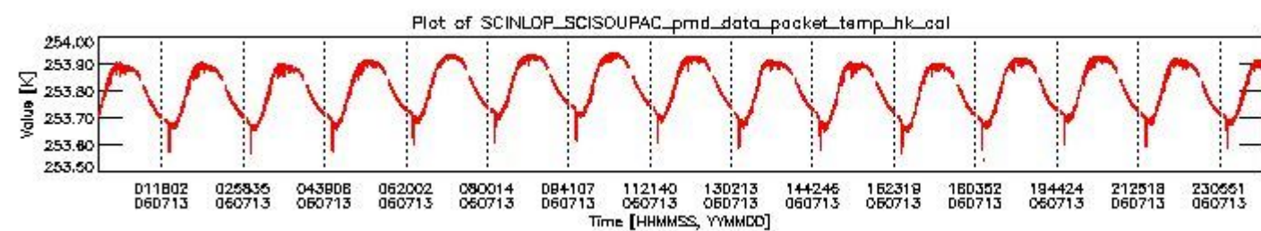
sciamachy_daily_report_level0_PFHS_5_37_N_20060713_3.PNG
