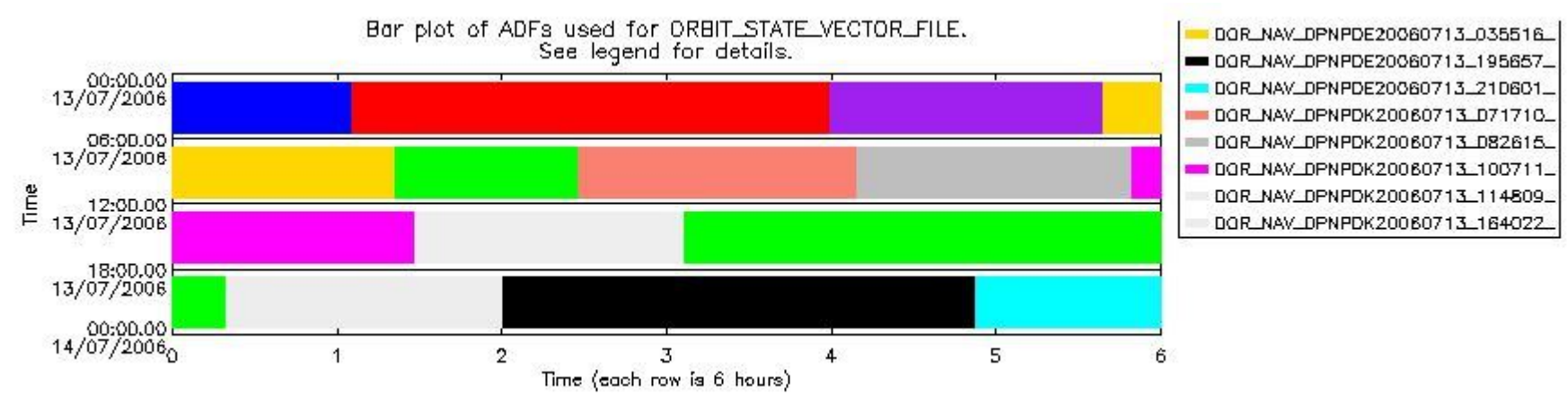
sciamachy_daily_report_level0_PFHS_5_37_N_20060713_6.PNG
