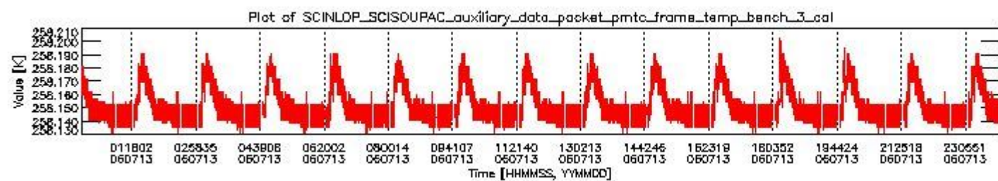
sciamachy_daily_report_level0_PFHS_5_37_N_20060713_2.PNG
