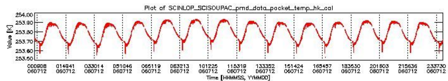
sciamachy_daily_report_level0_PFHS_5_37_N_20060712_3.PNG
