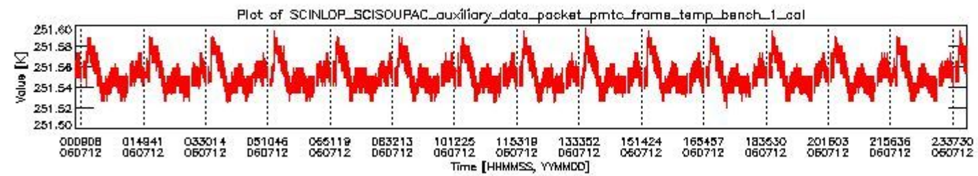
sciamachy_daily_report_level0_PFHS_5_37_N_20060712_0.PNG
