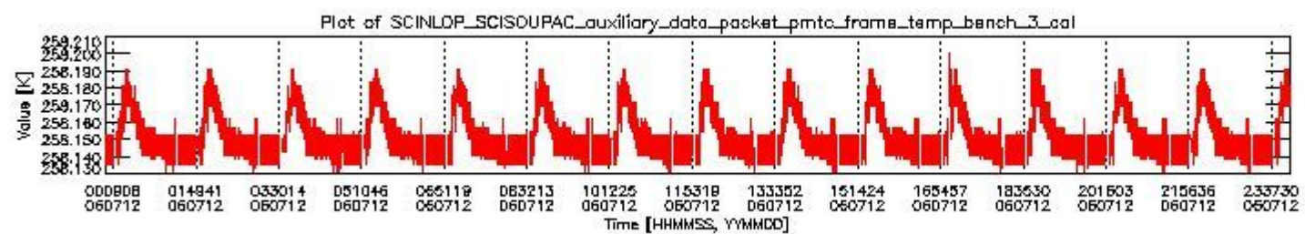
sciamachy_daily_report_level0_PFHS_5_37_N_20060712_2.PNG
