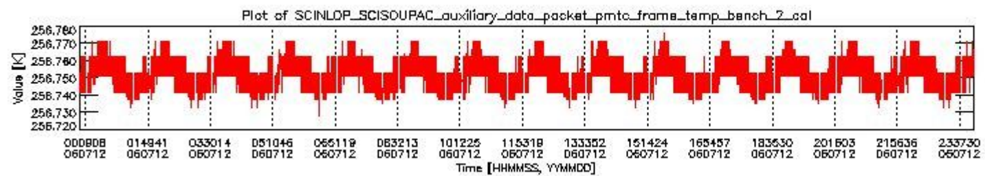
sciamachy_daily_report_level0_PFHS_5_37_N_20060712_1.PNG
