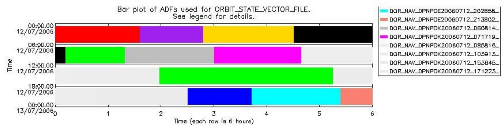
sciamachy_daily_report_level0_PFHS_5_37_N_20060712_6.PNG
