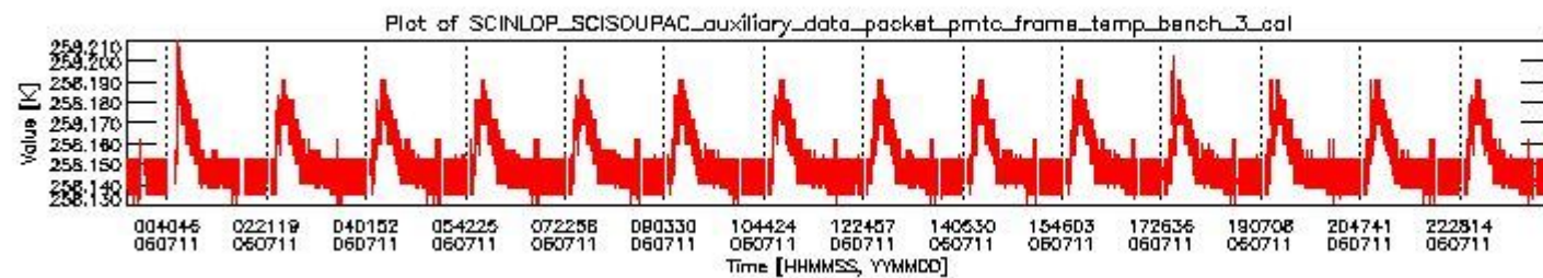
sciamachy_daily_report_level0_PFHS_5_37_N_20060711_2.PNG
