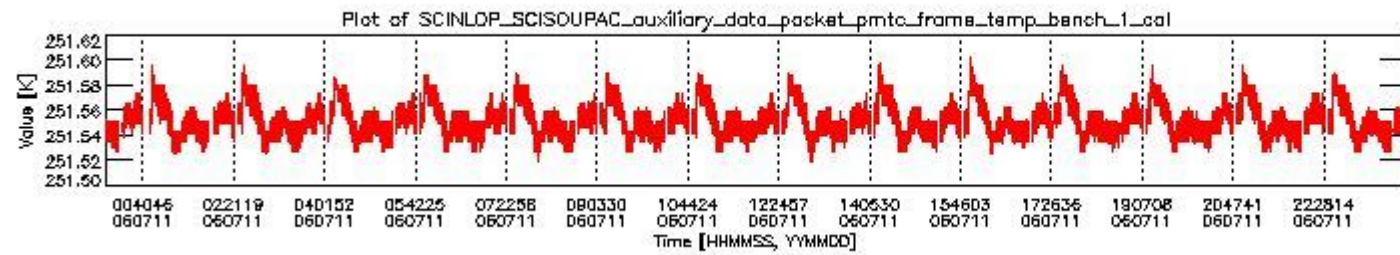
sciamachy_daily_report_level0_PFHS_5_37_N_20060711_0.PNG
