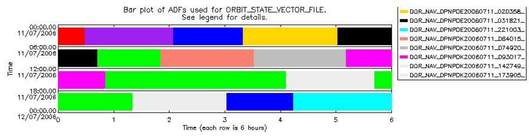
sciamachy_daily_report_level0_PFHS_5_37_N_20060711_6.PNG
