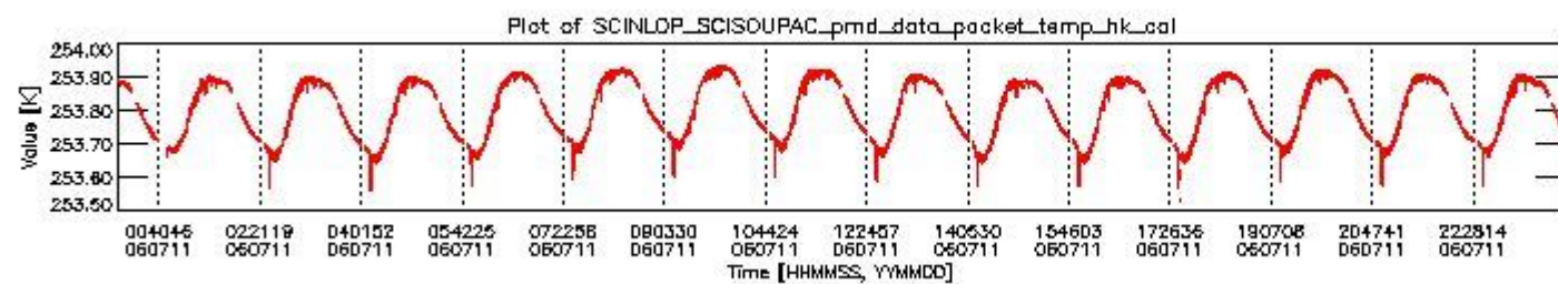
sciamachy_daily_report_level0_PFHS_5_37_N_20060711_3.PNG
