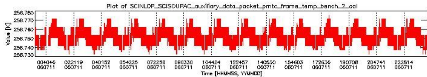
sciamachy_daily_report_level0_PFHS_5_37_N_20060711_1.PNG
