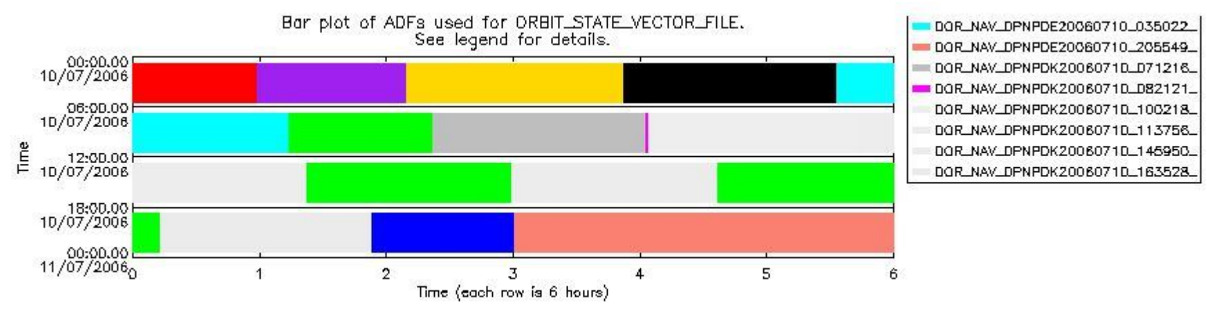
sciamachy_daily_report_level0_PFHS_5_37_N_20060710_6.PNG
