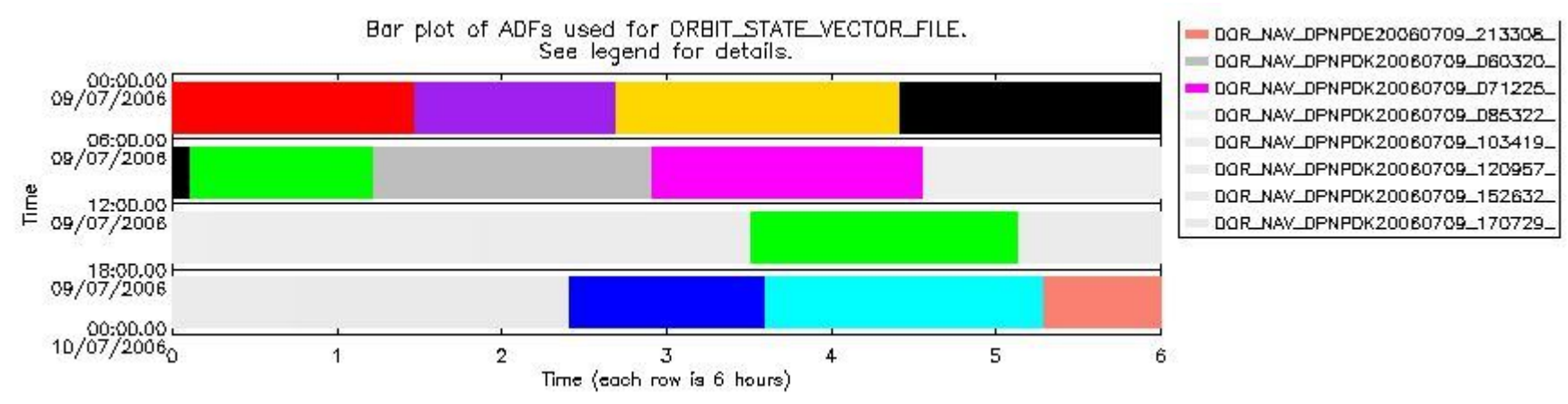
sciamachy_daily_report_level0_PFHS_5_37_N_20060709_6.PNG
