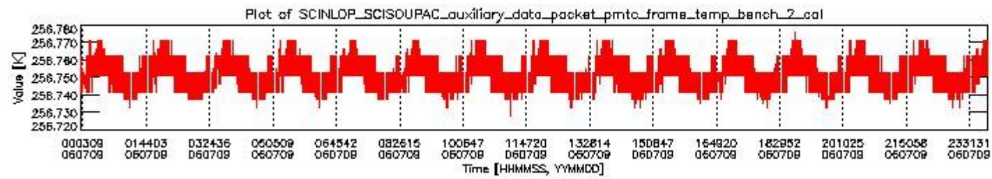
sciamachy_daily_report_level0_PFHS_5_37_N_20060709_1.PNG
