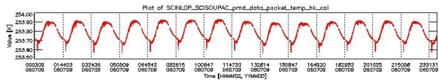
sciamachy_daily_report_level0_PFHS_5_37_N_20060709_3.PNG
