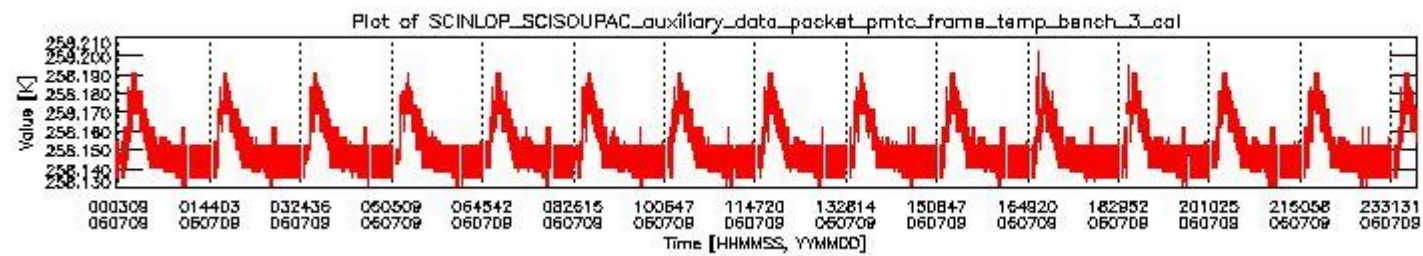
sciamachy_daily_report_level0_PFHS_5_37_N_20060709_2.PNG
