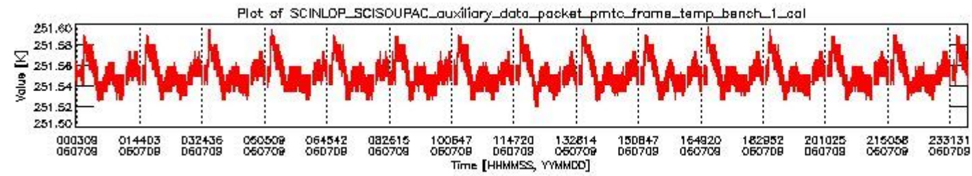
sciamachy_daily_report_level0_PFHS_5_37_N_20060709_0.PNG
