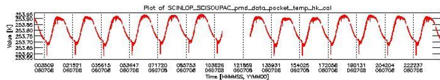
sciamachy_daily_report_level0_PFHS_5_37_N_20060708_3.PNG
