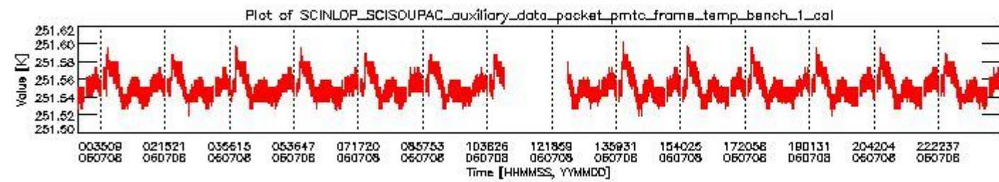
sciamachy_daily_report_level0_PFHS_5_37_N_20060708_0.PNG
