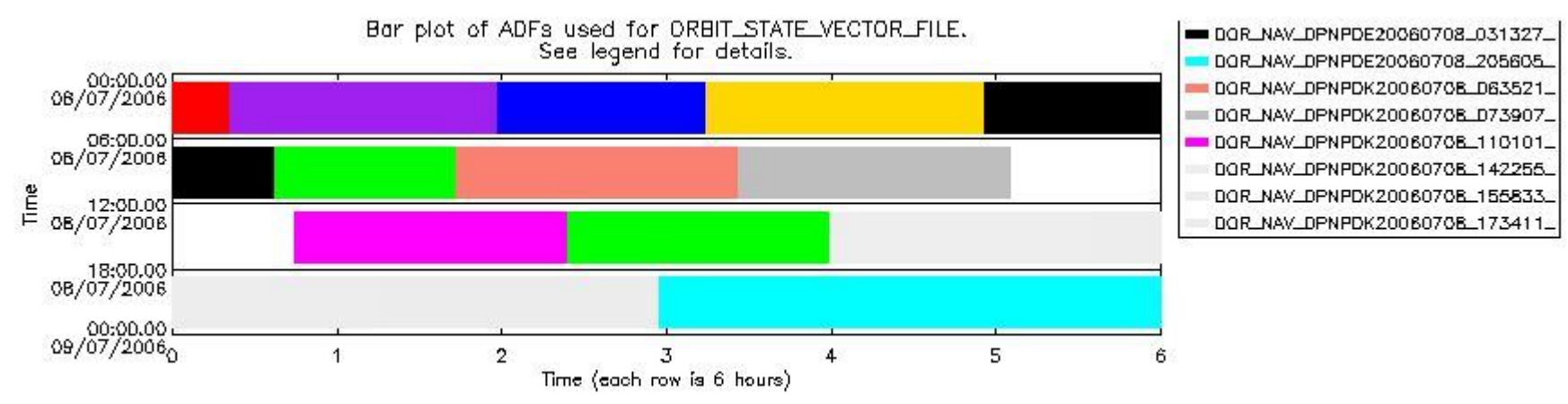
sciamachy_daily_report_level0_PFHS_5_37_N_20060708_6.PNG
