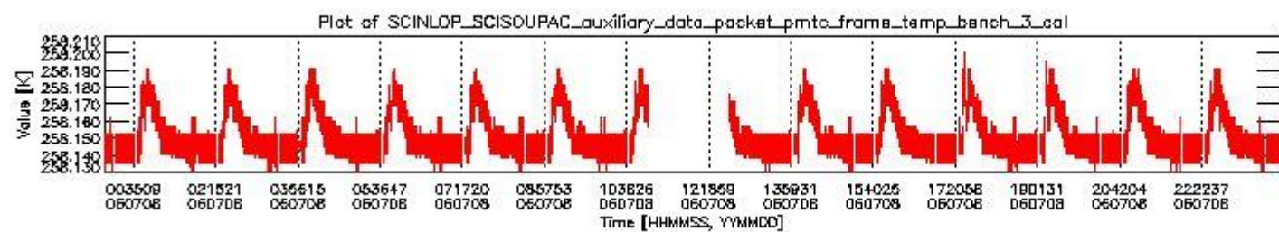
sciamachy_daily_report_level0_PFHS_5_37_N_20060708_2.PNG
