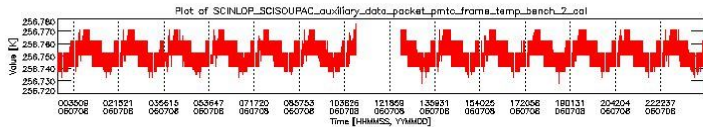
sciamachy_daily_report_level0_PFHS_5_37_N_20060708_1.PNG
