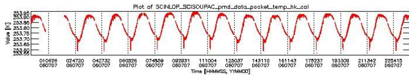
sciamachy_daily_report_level0_PFHS_5_37_N_20060707_3.PNG
