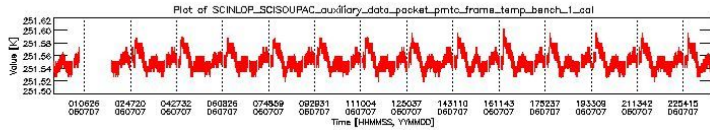
sciamachy_daily_report_level0_PFHS_5_37_N_20060707_0.PNG
