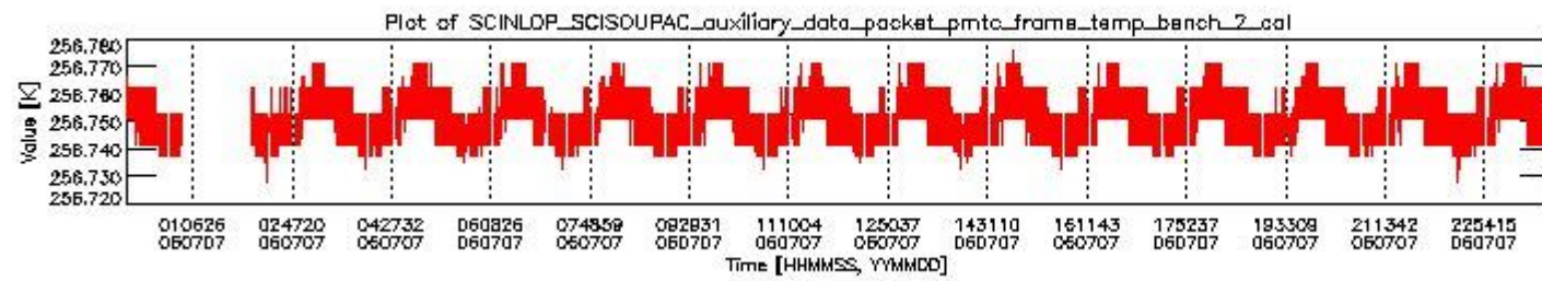
sciamachy_daily_report_level0_PFHS_5_37_N_20060707_1.PNG
