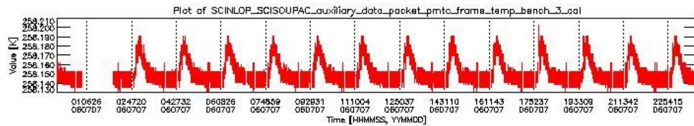
sciamachy_daily_report_level0_PFHS_5_37_N_20060707_2.PNG
