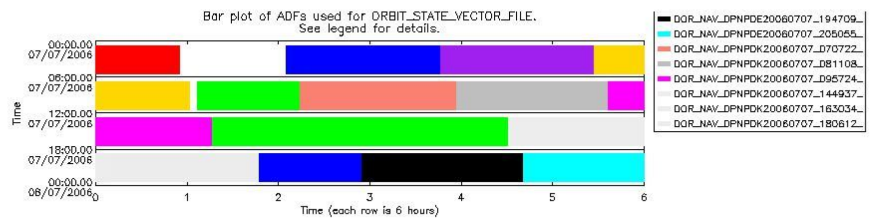
sciamachy_daily_report_level0_PFHS_5_37_N_20060707_6.PNG
