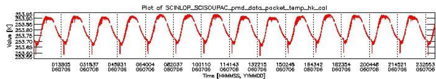
sciamachy_daily_report_level0_PFH5_5_37_N_20060706_3.PNG
