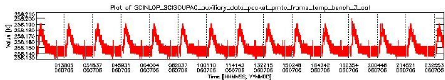
sciamachy_daily_report_level0_PFH5_5_37_N_20060706_2.PNG
