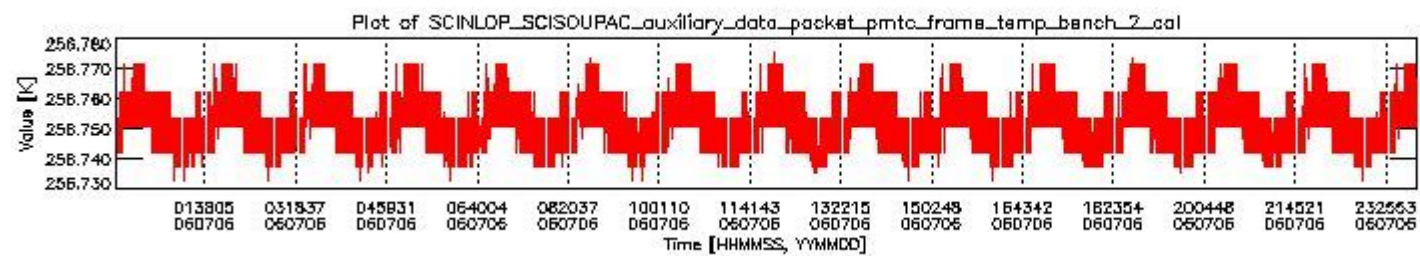
sciamachy_daily_report_level0_PFH5_5_37_N_20060706_1.PNG
