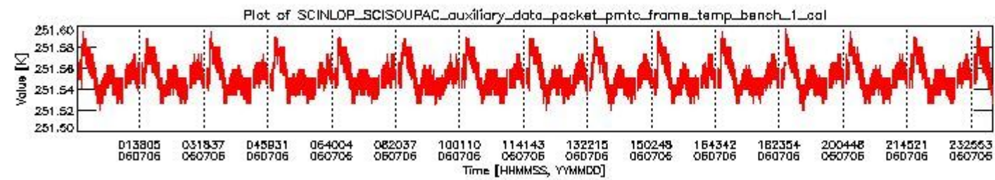
sciamachy_daily_report_level0_PFH5_5_37_N_20060706_0.PNG
