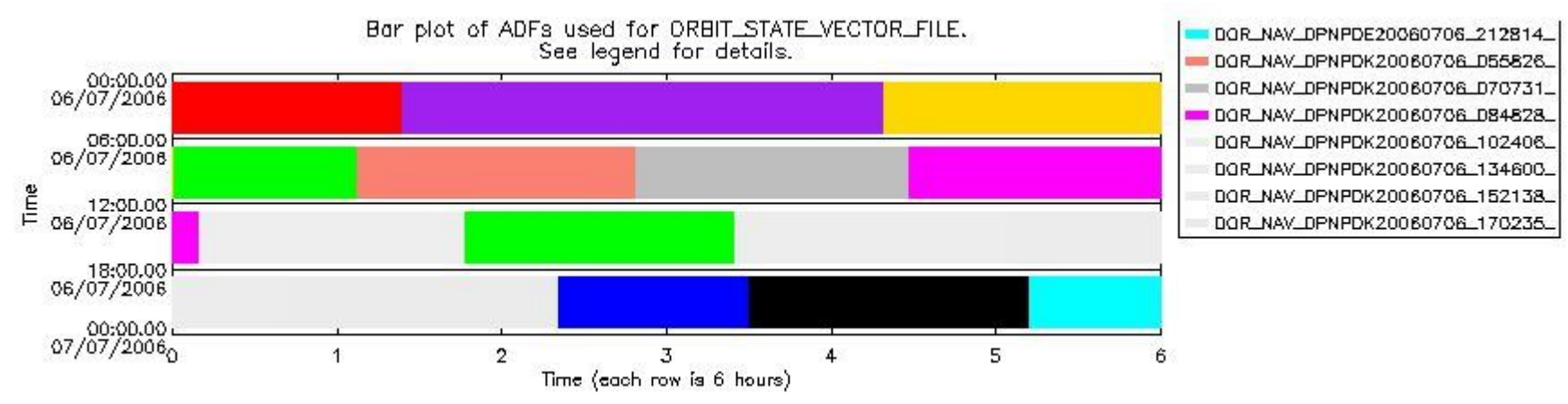
sciamachy_daily_report_level0_PFHS_5_37_N_20060706_6.PNG
