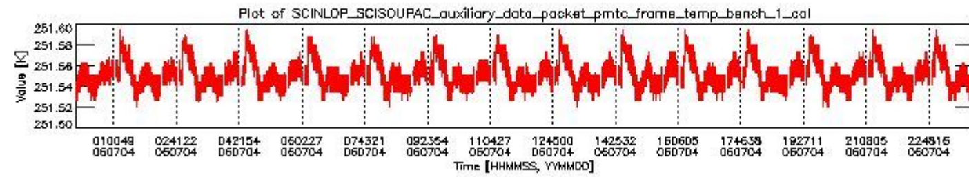
sciamachy_daily_report_level0_PFHS_5_37_N_20060704_0.PNG
