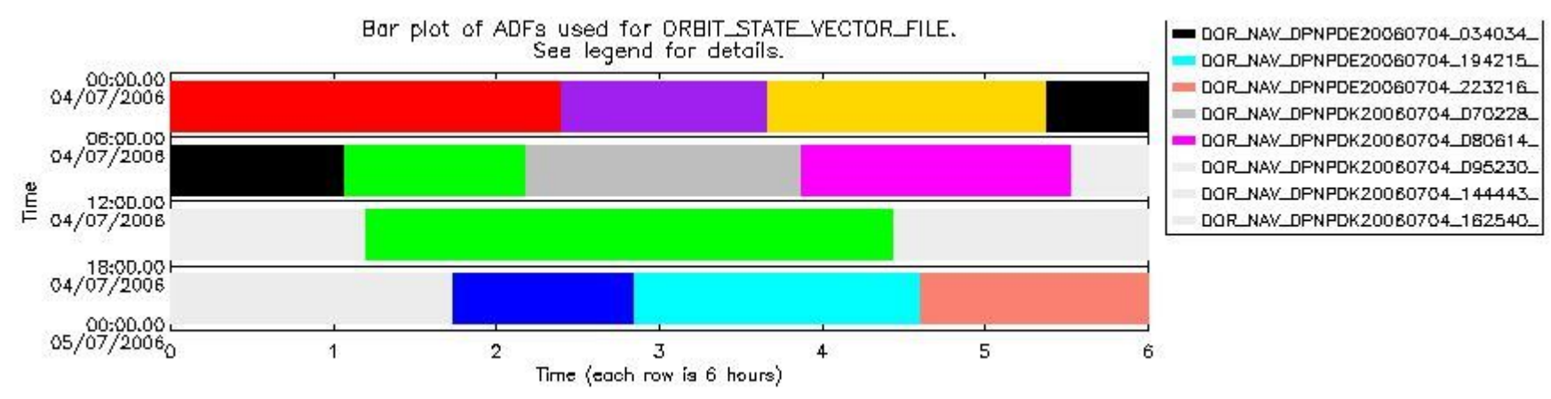
sciamachy_daily_report_level0_PFHS_5_37_N_20060704_6.PNG
