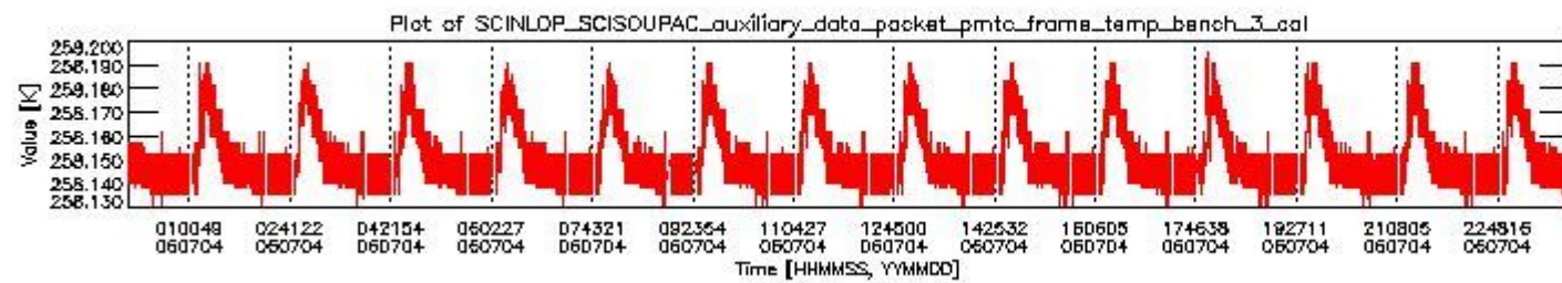
sciamachy_daily_report_level0_PFHS_5_37_N_20060704_2.PNG
