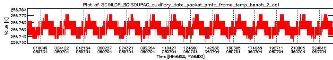
sciamachy_daily_report_level0_PFHS_5_37_N_20060704_1.PNG
