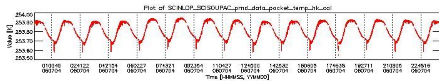
sciamachy_daily_report_level0_PFHS_5_37_N_20060704_3.PNG
