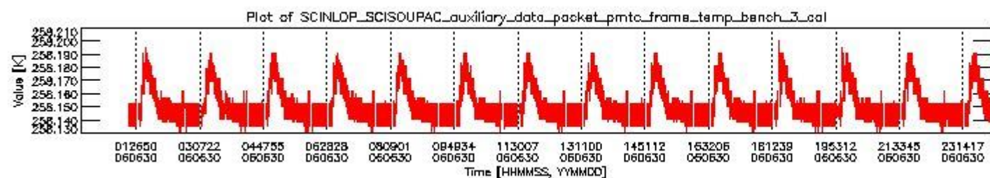
sciamachy_daily_report_level0_PFHS_5_37_N_20060630_2.PNG
