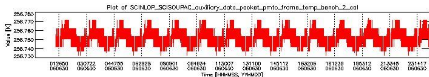
sciamachy_daily_report_level0_PFHS_5_37_N_20060630_1.PNG
