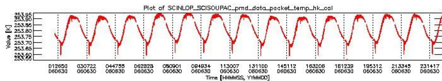
sciamachy_daily_report_level0_PFHS_5_37_N_20060630_3.PNG
