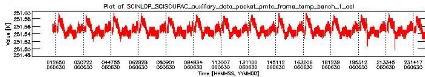
sciamachy_daily_report_level0_PFHS_5_37_N_20060630_0.PNG
