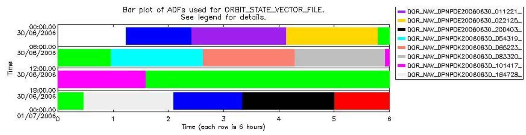
sciamachy_daily_report_level0_PFHS_5_37_N_20060630_6.PNG
