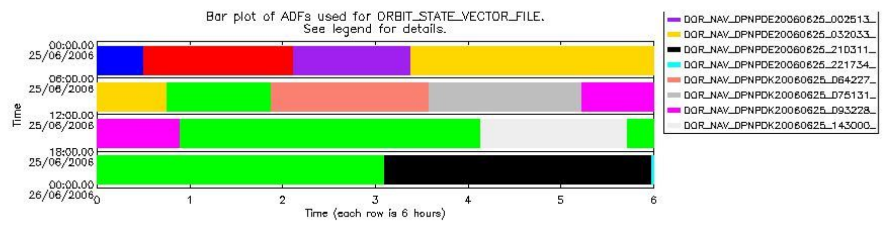
sciamachy_daily_report_level0_PFHS_5_36_N_20060625_6.PNG
