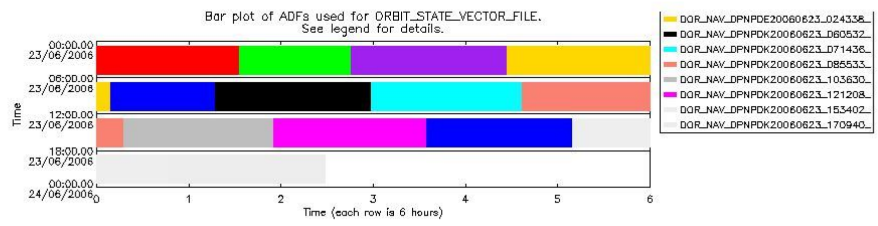
sciamachy_daily_report_level0_PFHS_5_36_N_20060623_6.PNG
