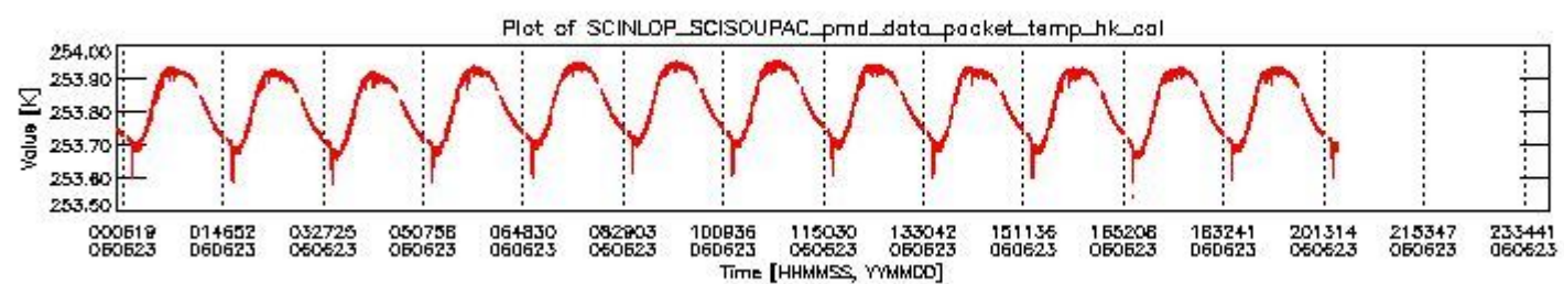
sciamachy_daily_report_level0_PFHS_5_36_N_20060623_3.PNG
