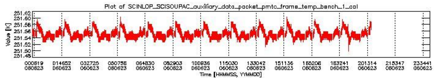
sciamachy_daily_report_level0_PFHS_5_36_N_20060623_0.PNG
