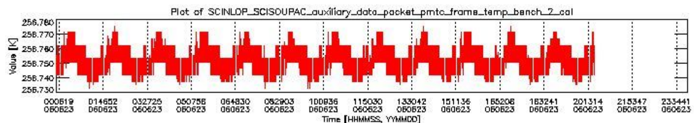
sciamachy_daily_report_level0_PFHS_5_36_N_20060623_1.PNG
